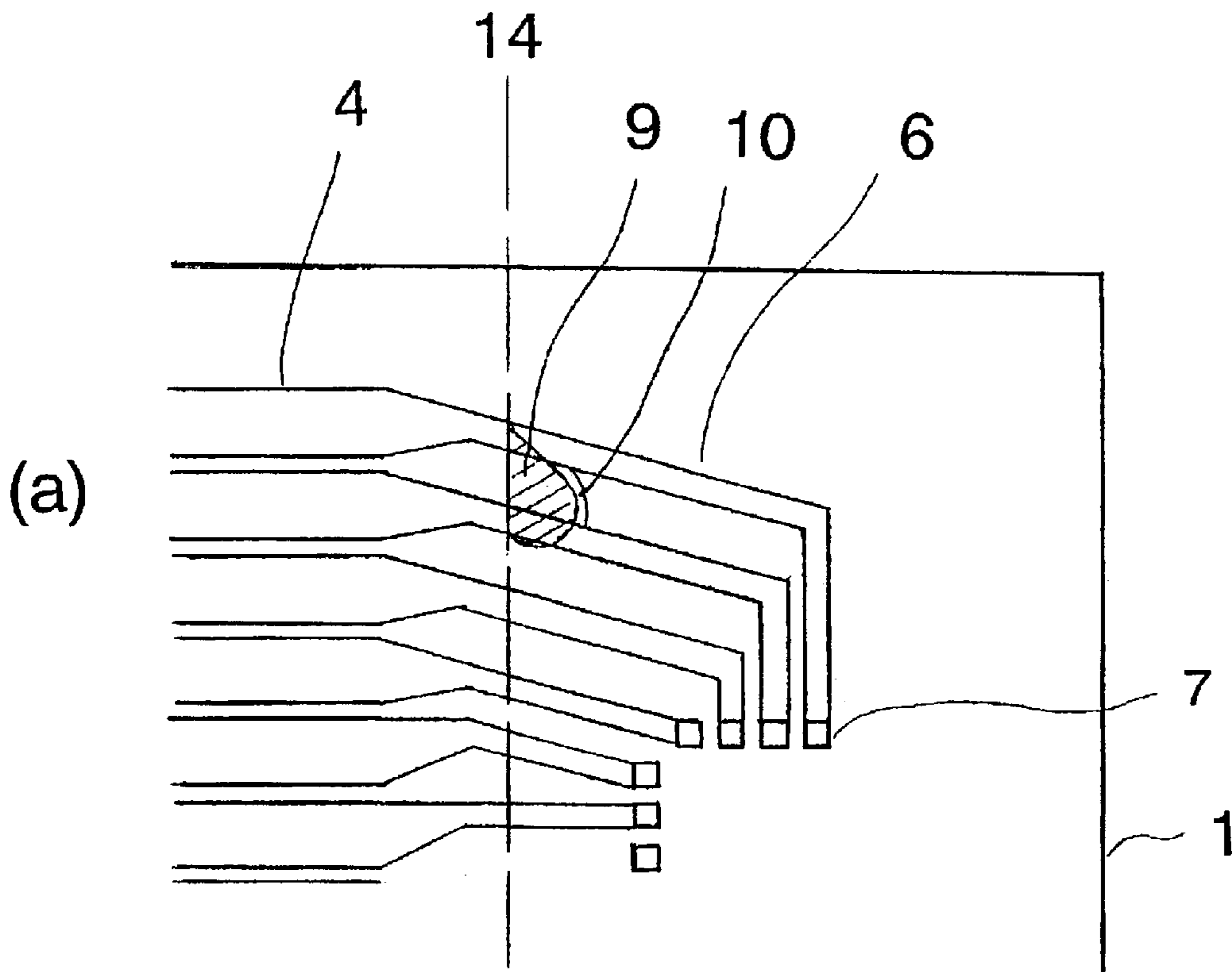
FIG. 2B
