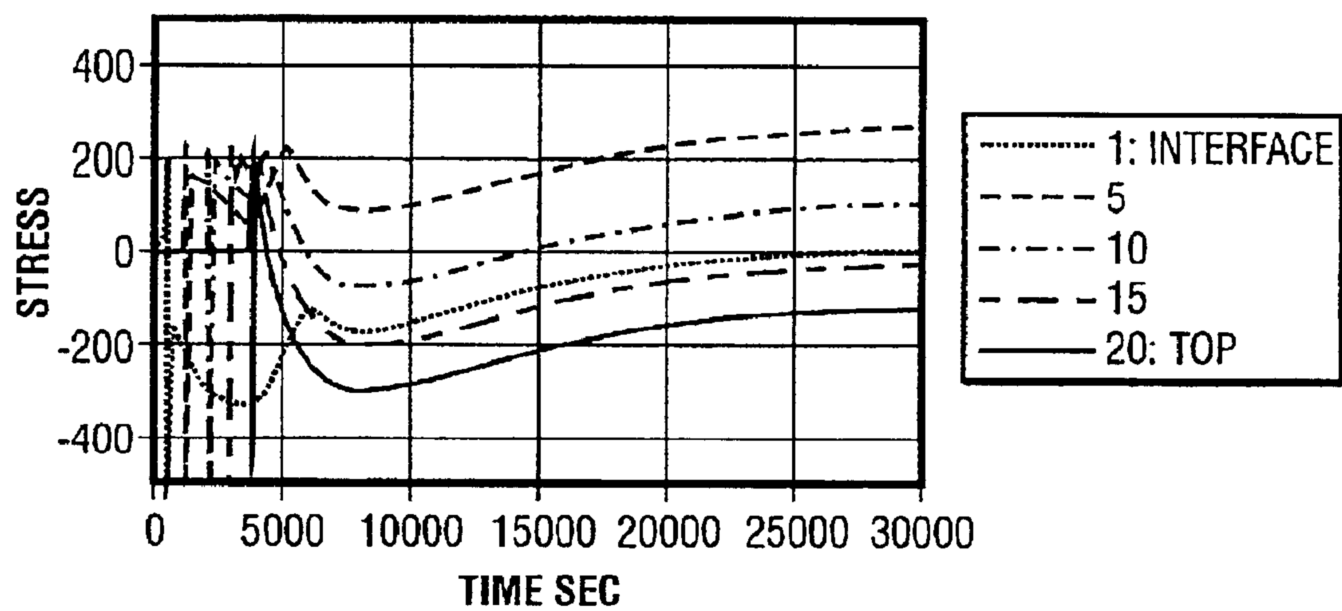
In-Plane Stress FIG. 16
