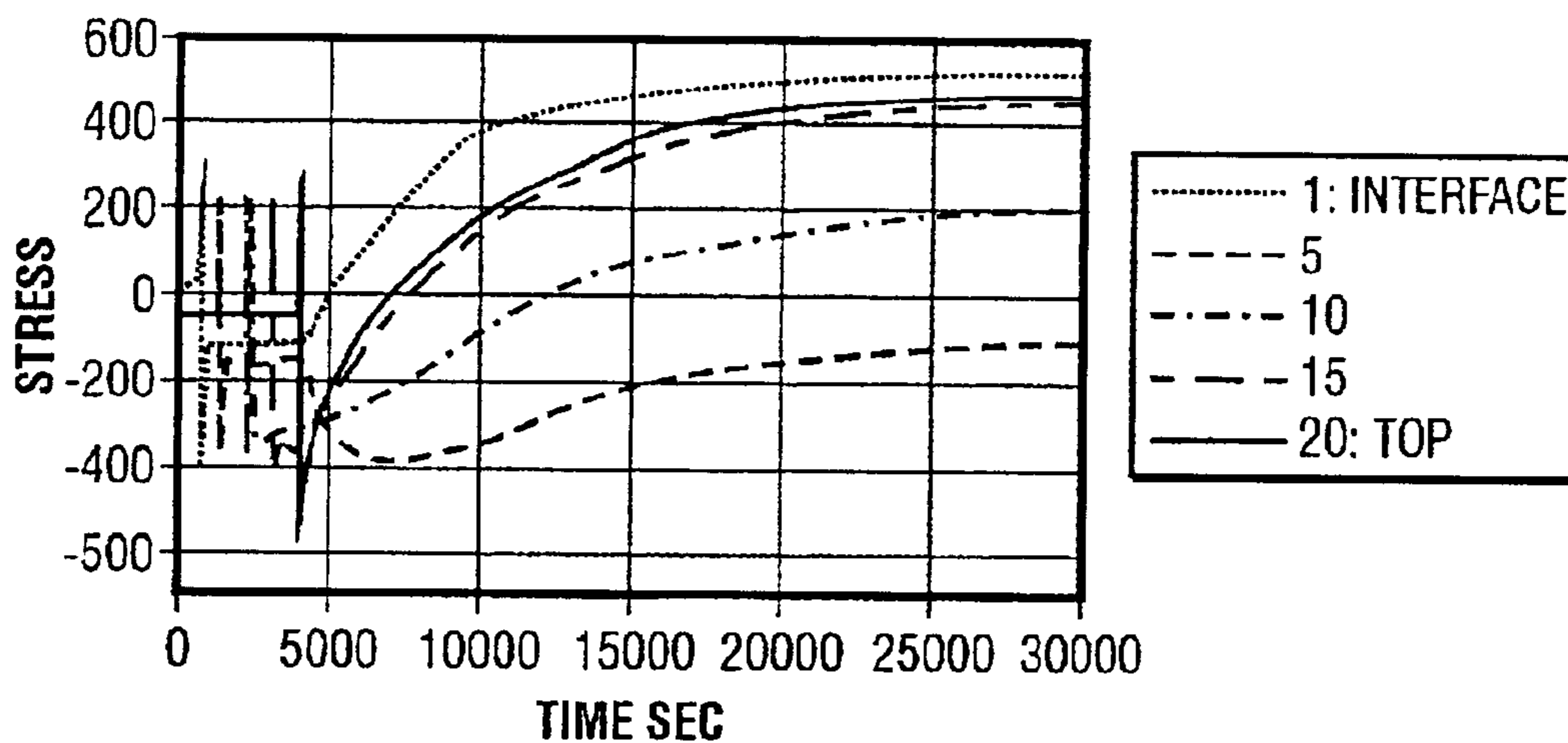
In-Plane Stress FIG. 11
