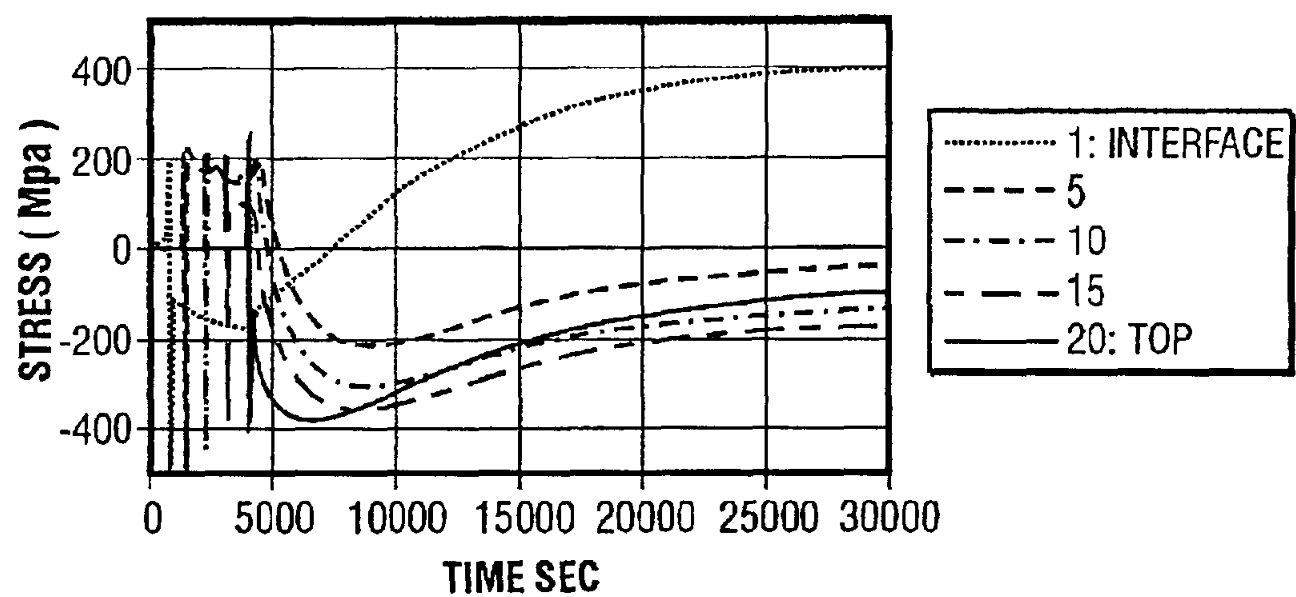
In-Plane Stress FIG. 6
