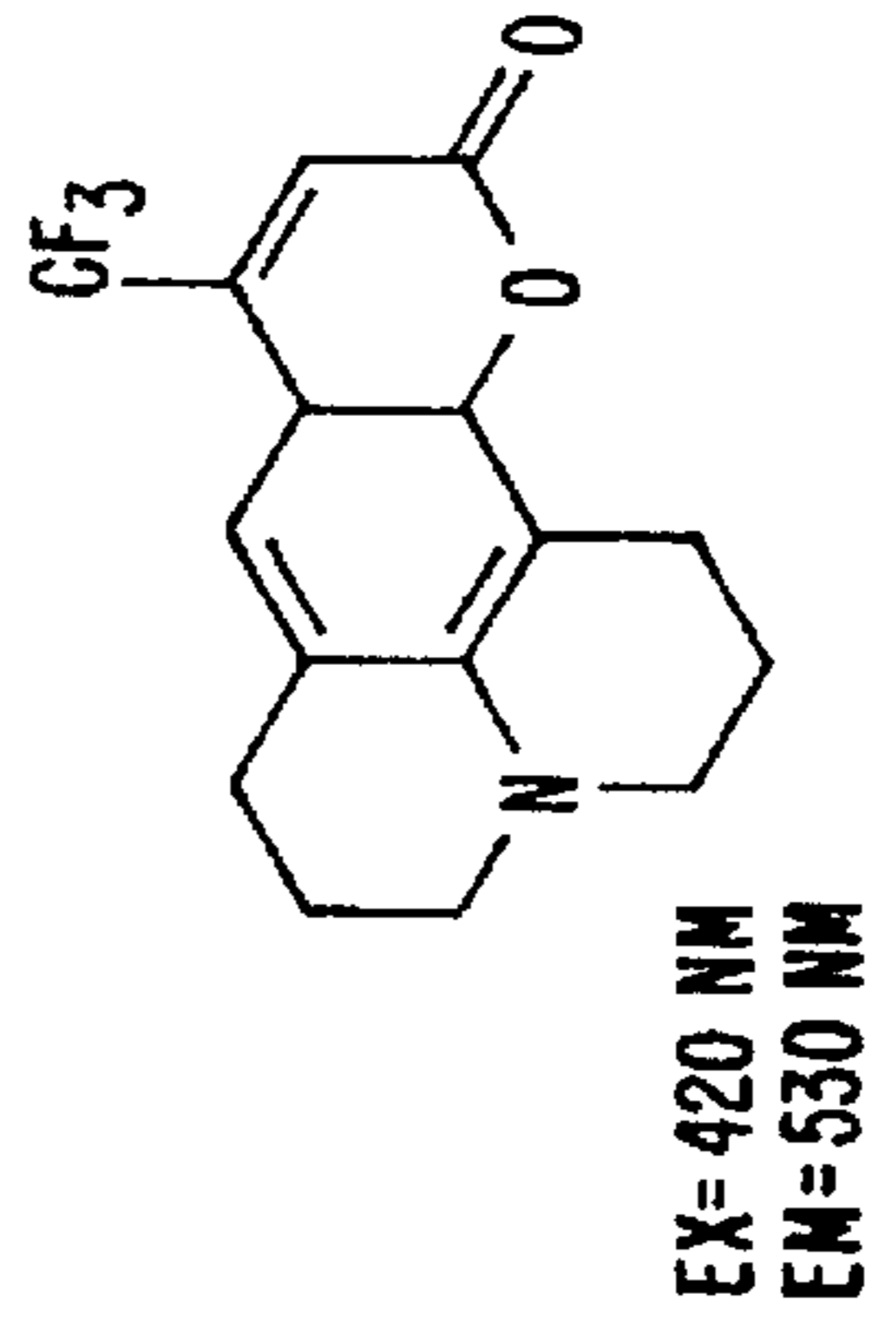
COUMARIN 153
