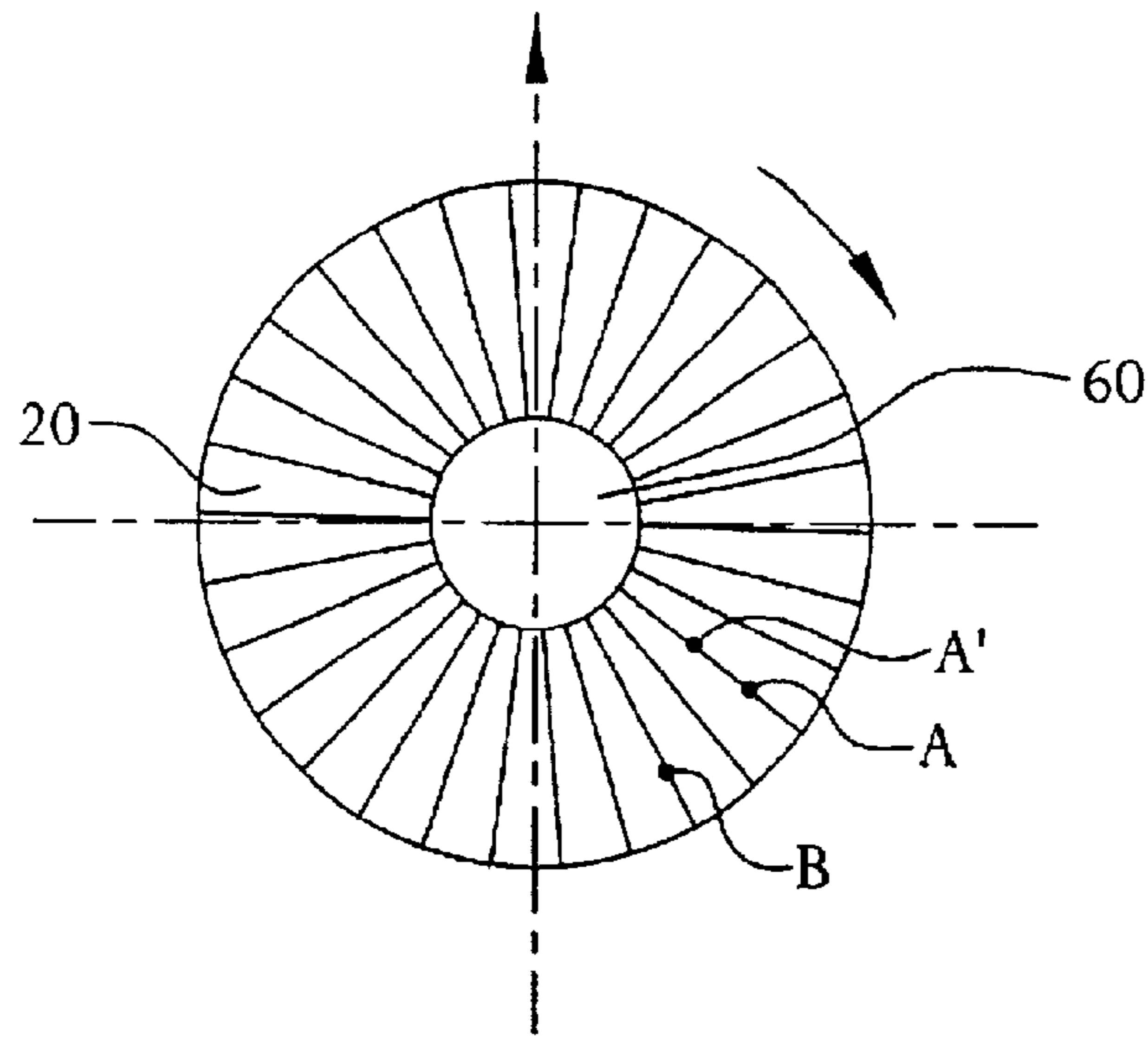
FIG. 10
