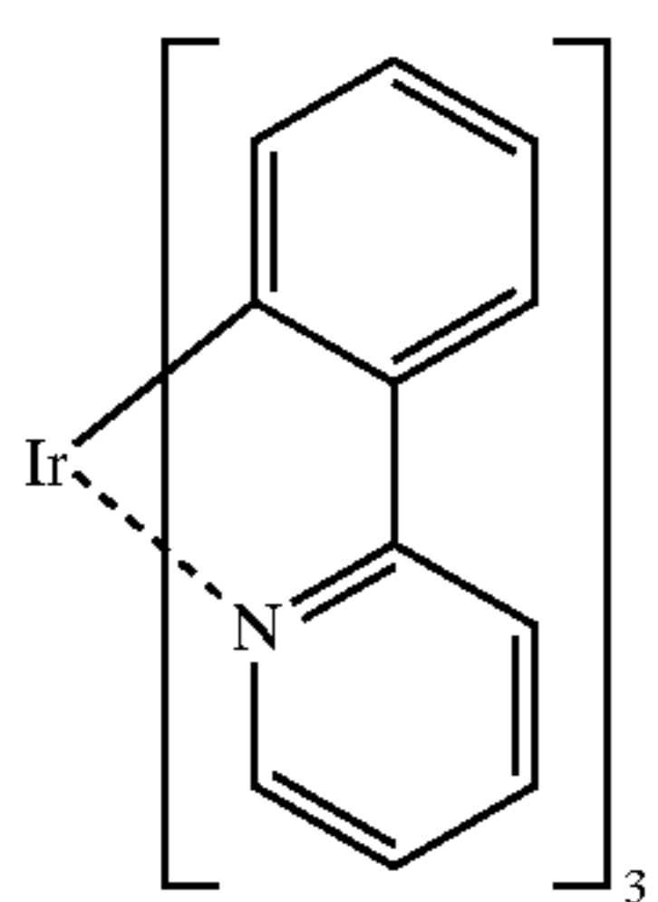
Ir(ppy) 3
