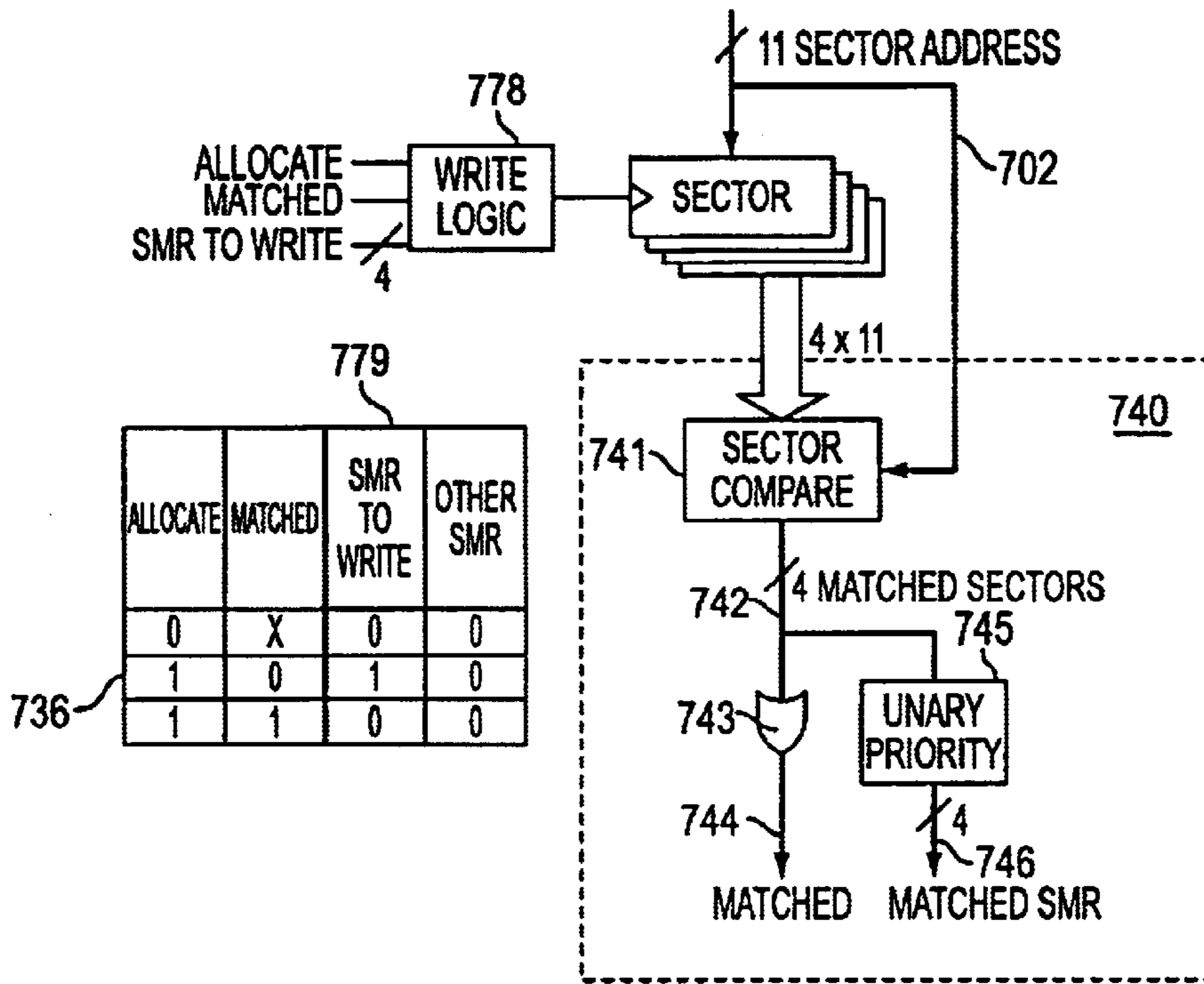
Sector match logic FIG. 7E
