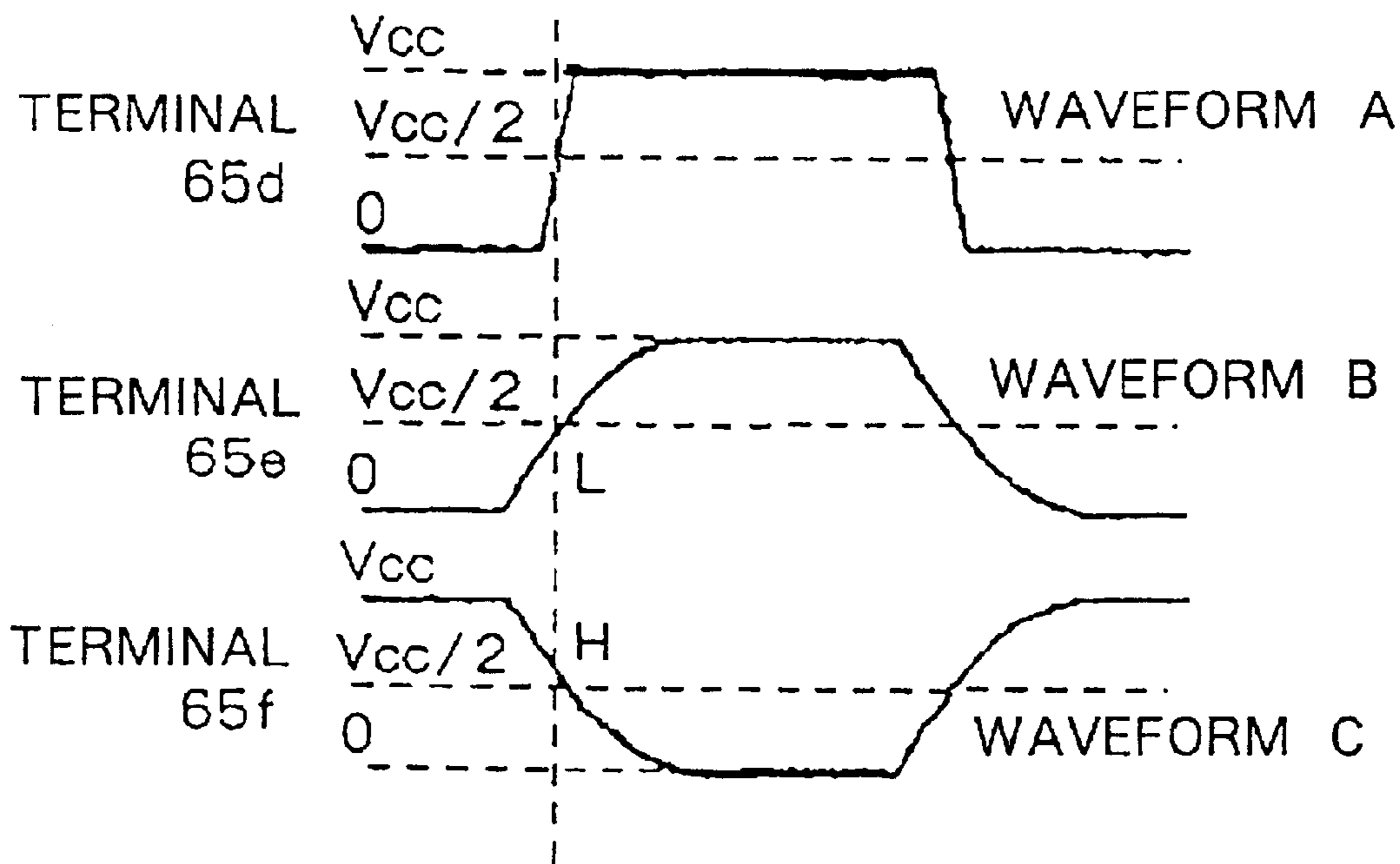
FIG. 6E (PRIOR ART)
