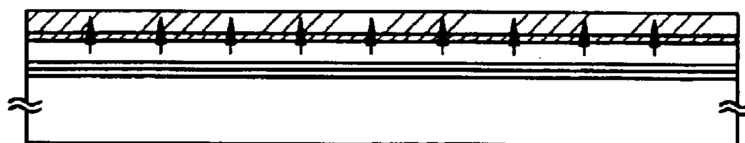
FIG. 37D GETTERING
