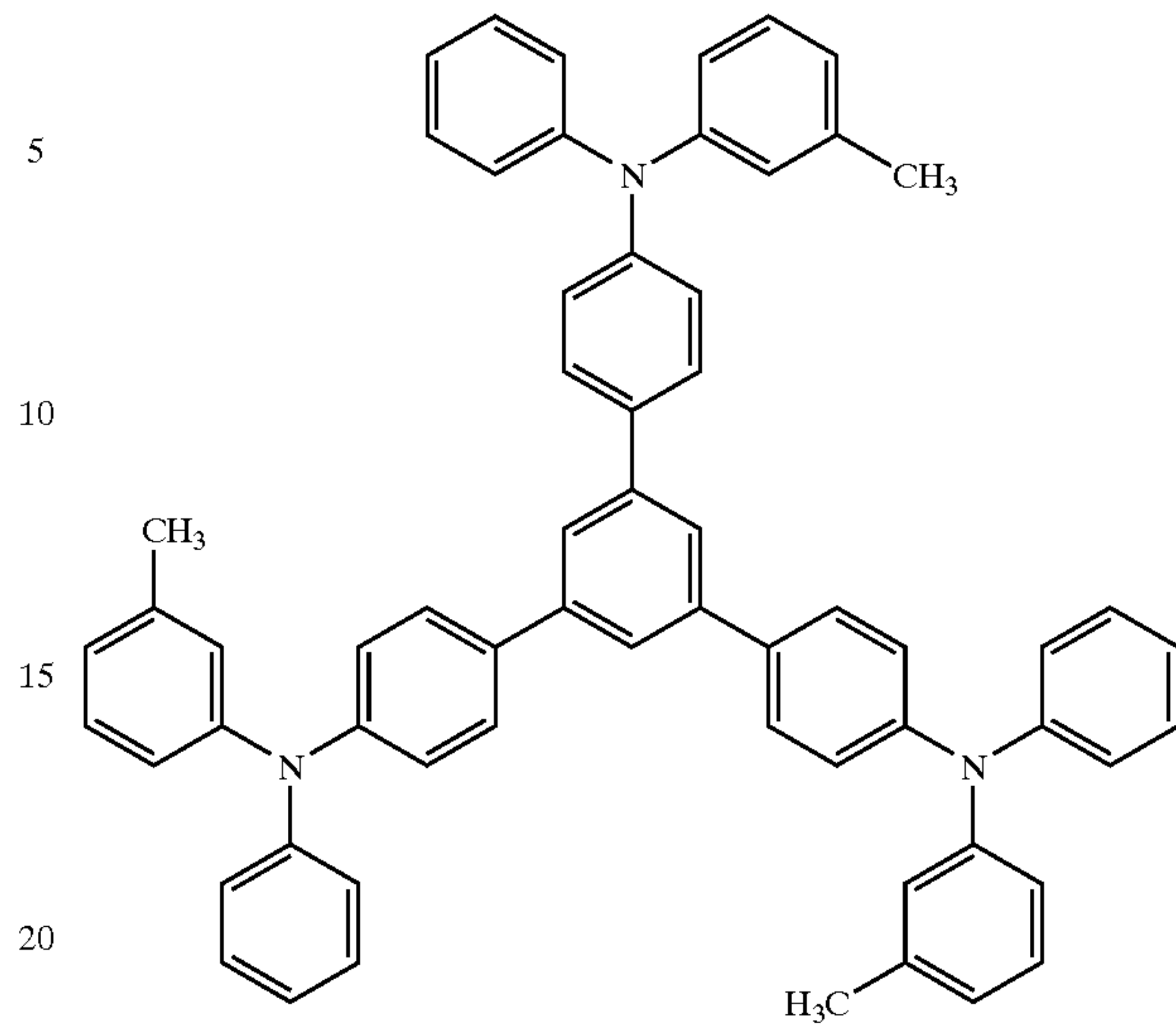
m-MTDAPB T g = 105° C. J. Mater. Chem., 3,319 (1993). Mol. Cryst. Liq. Cryst., 280,331(1996).
