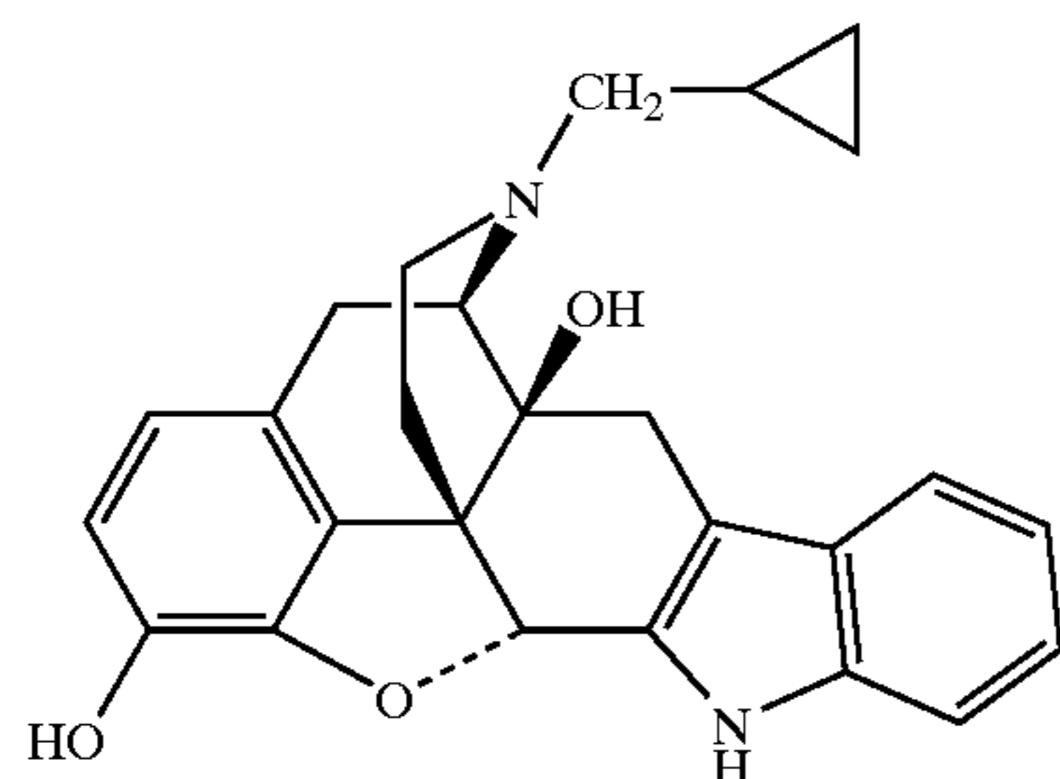
Naltrindole
