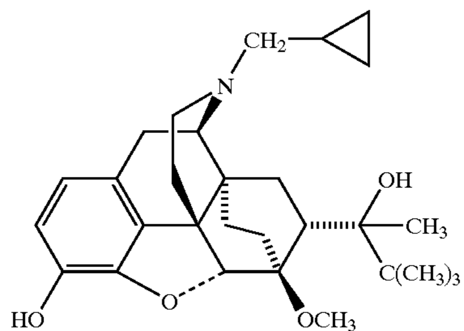
Buprenorphine
