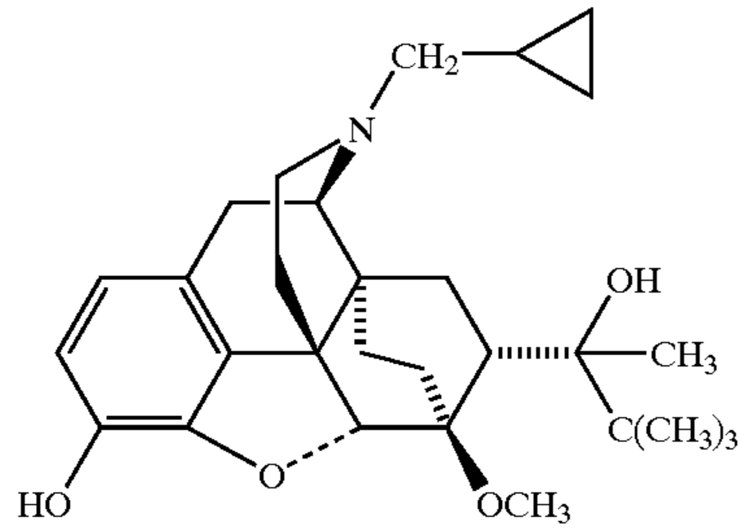
Buprenorphine
