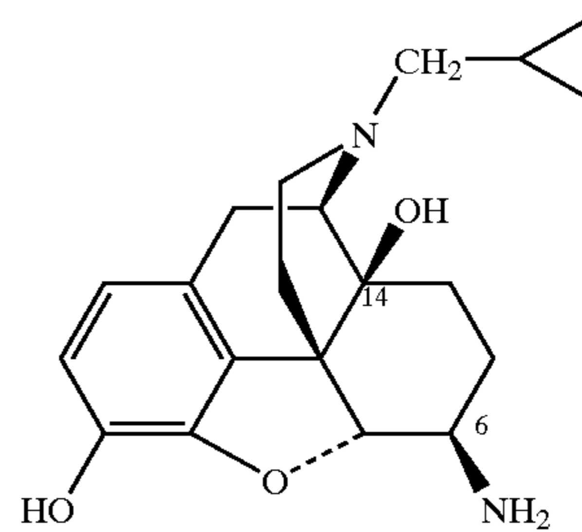
β-Naltrexamine
