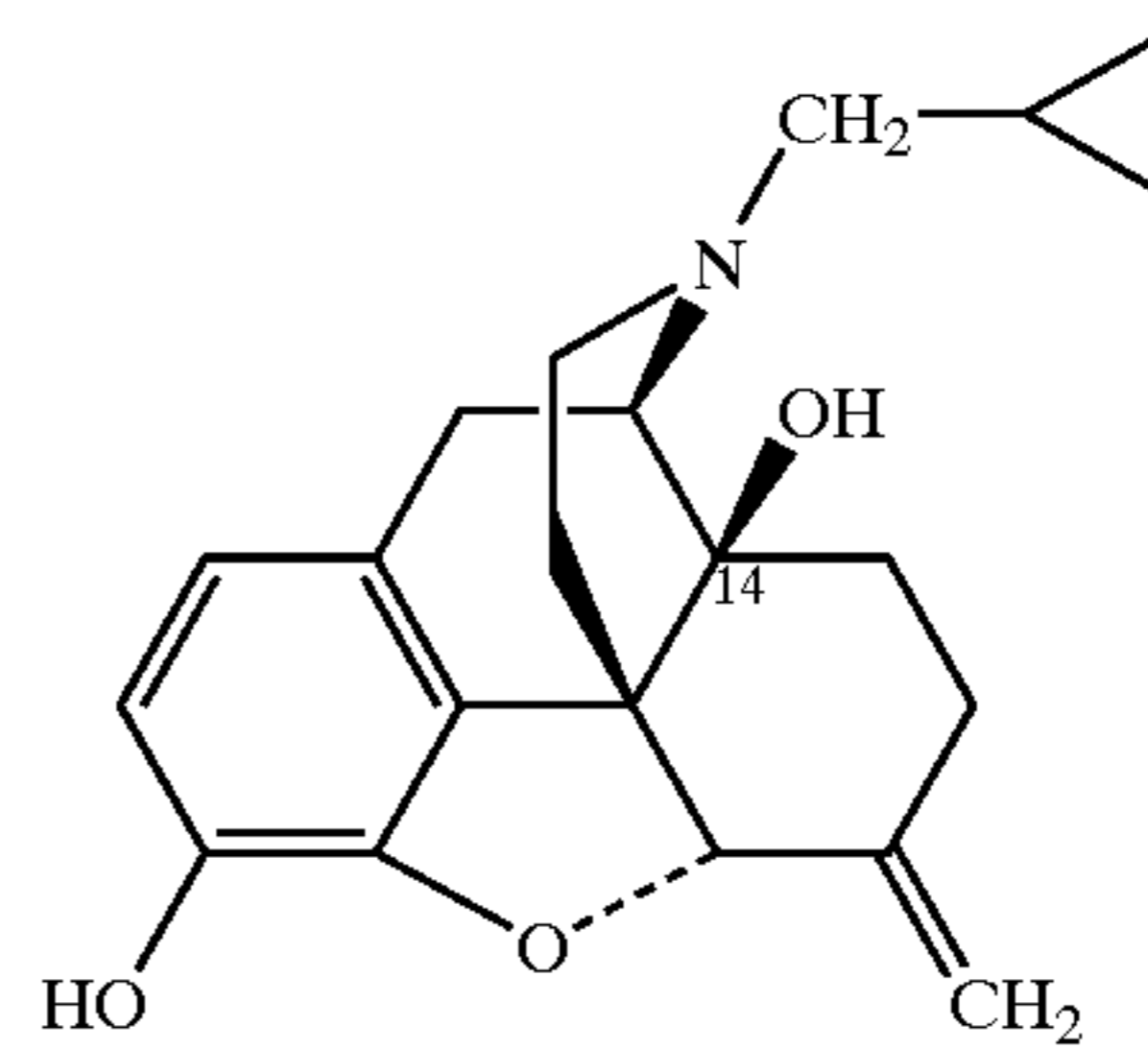
Nalmefene
