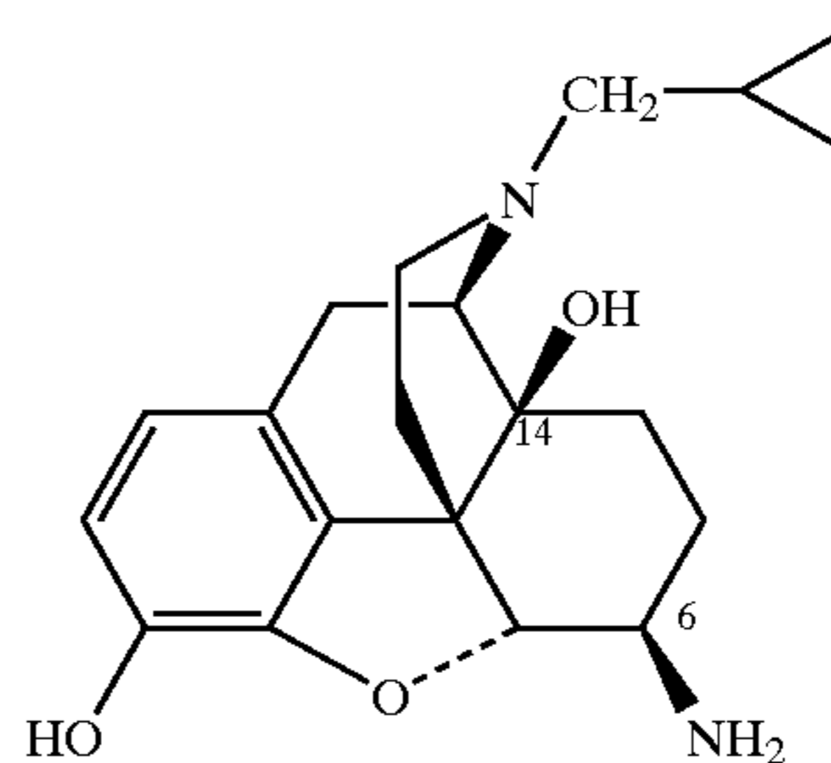
\beta -Naltrexamine
