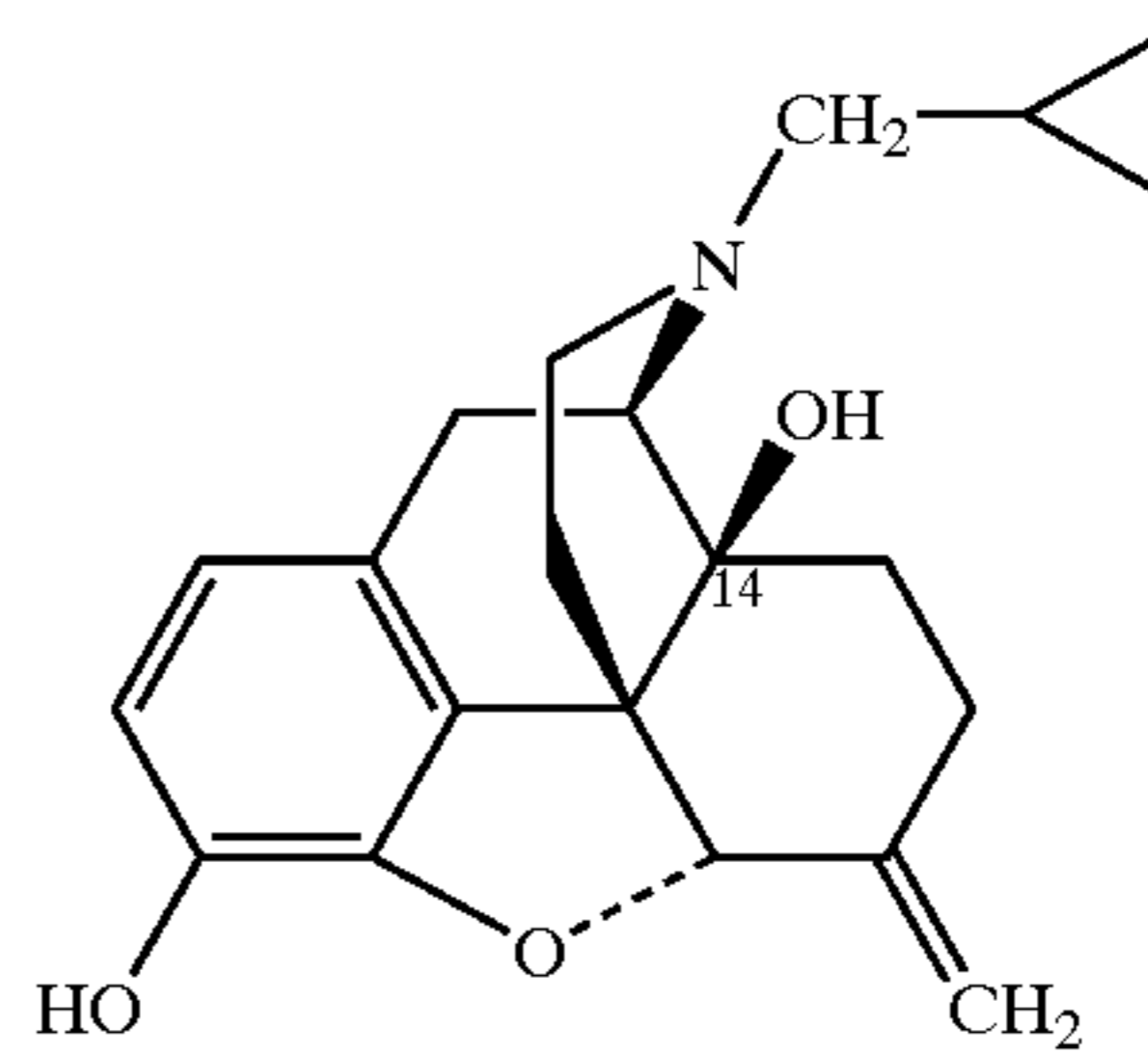
Nalmefene
