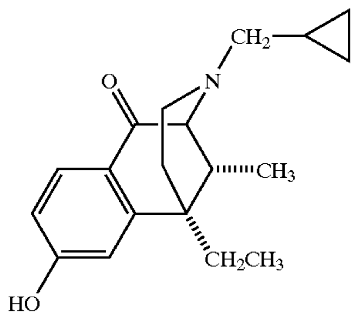
Ethylketocyclazocine (EKC)
