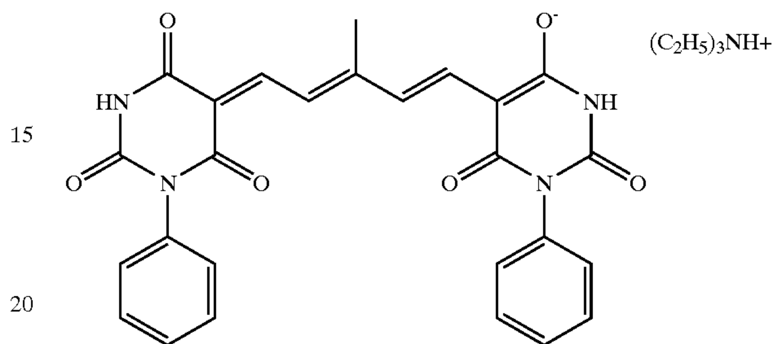
Dye-3c-A
