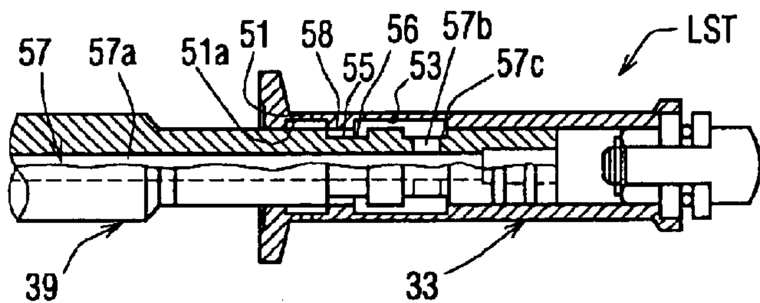
FIG. 4B
