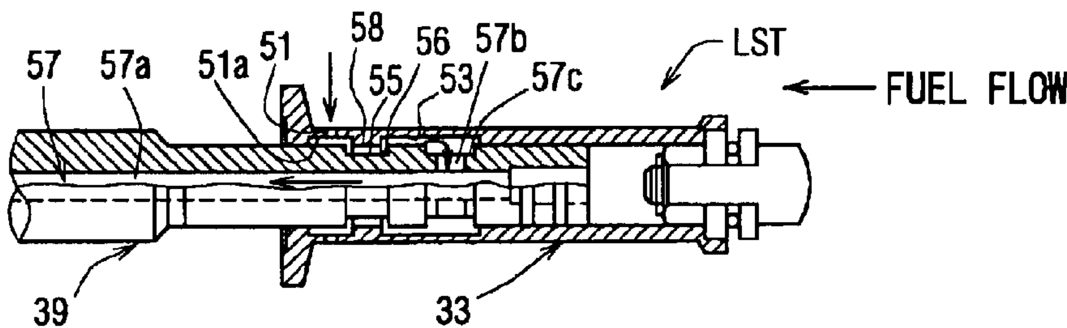
FIG. 4C
