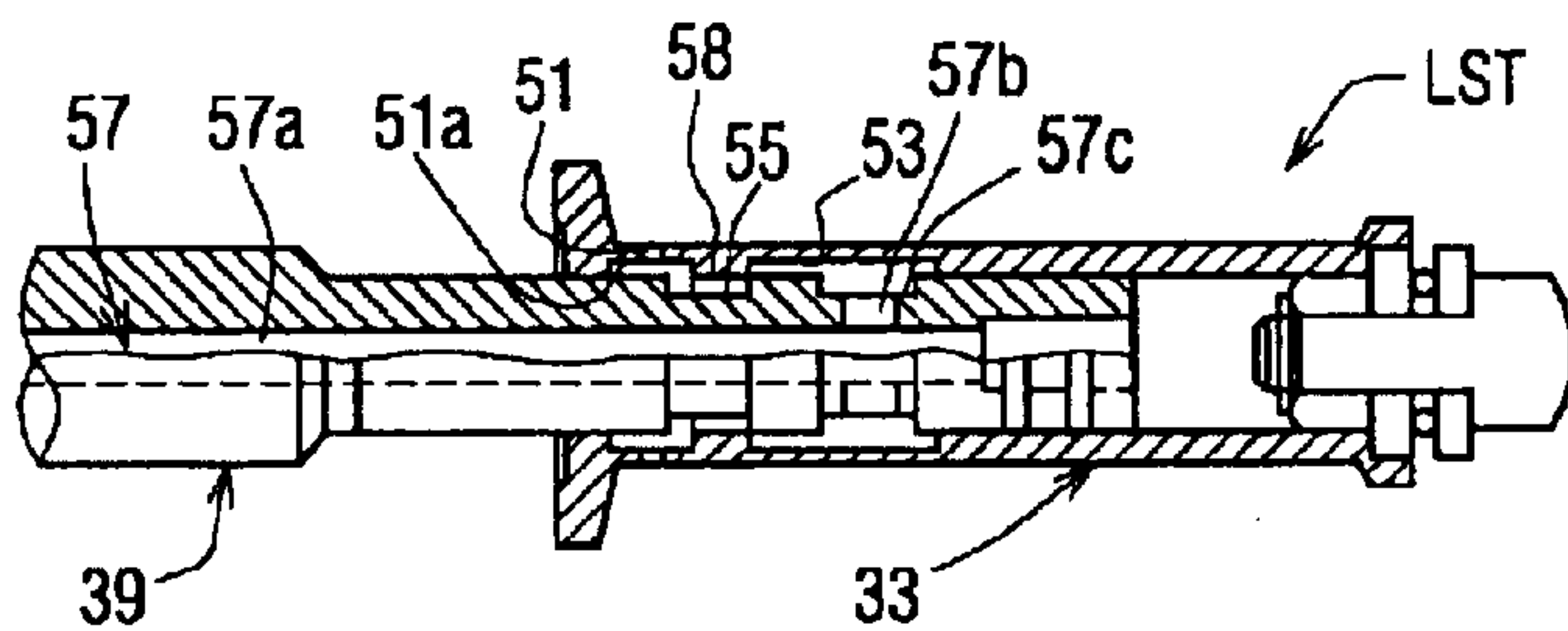
FIG. 4D
