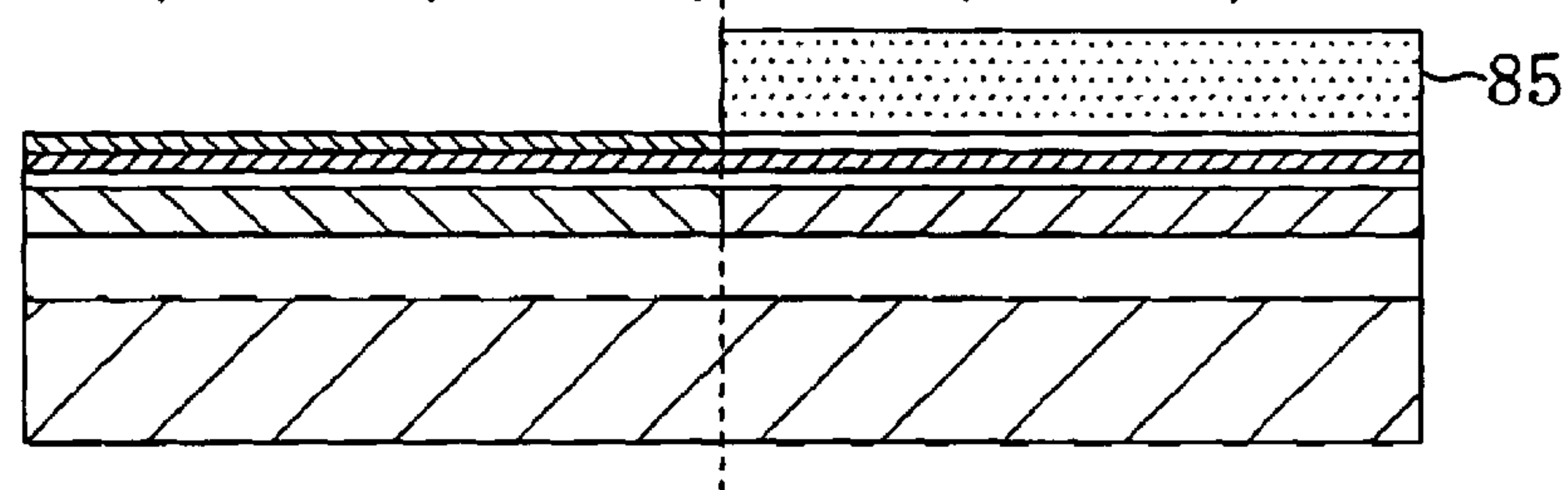
FIG. 12(b) ↓ ↓ ↓ ↓ ↓ P-type impurity ions
