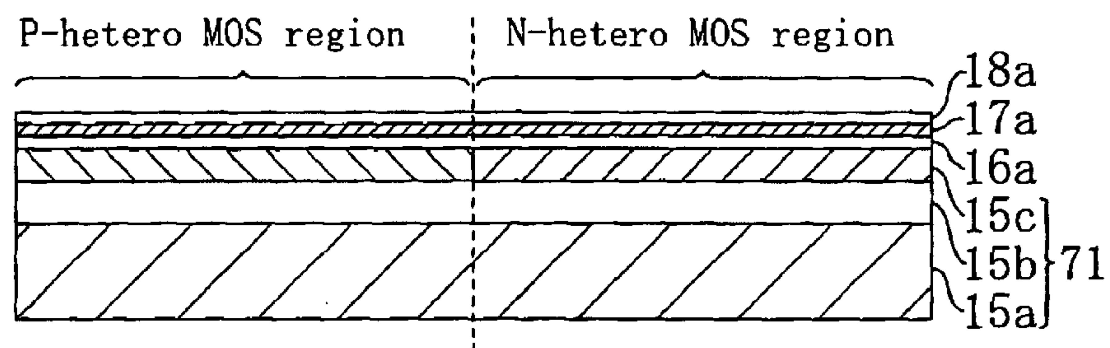
FIG. 12(b) ↓ ↓ ↓ ↓ ↓ P-type impurity ions
