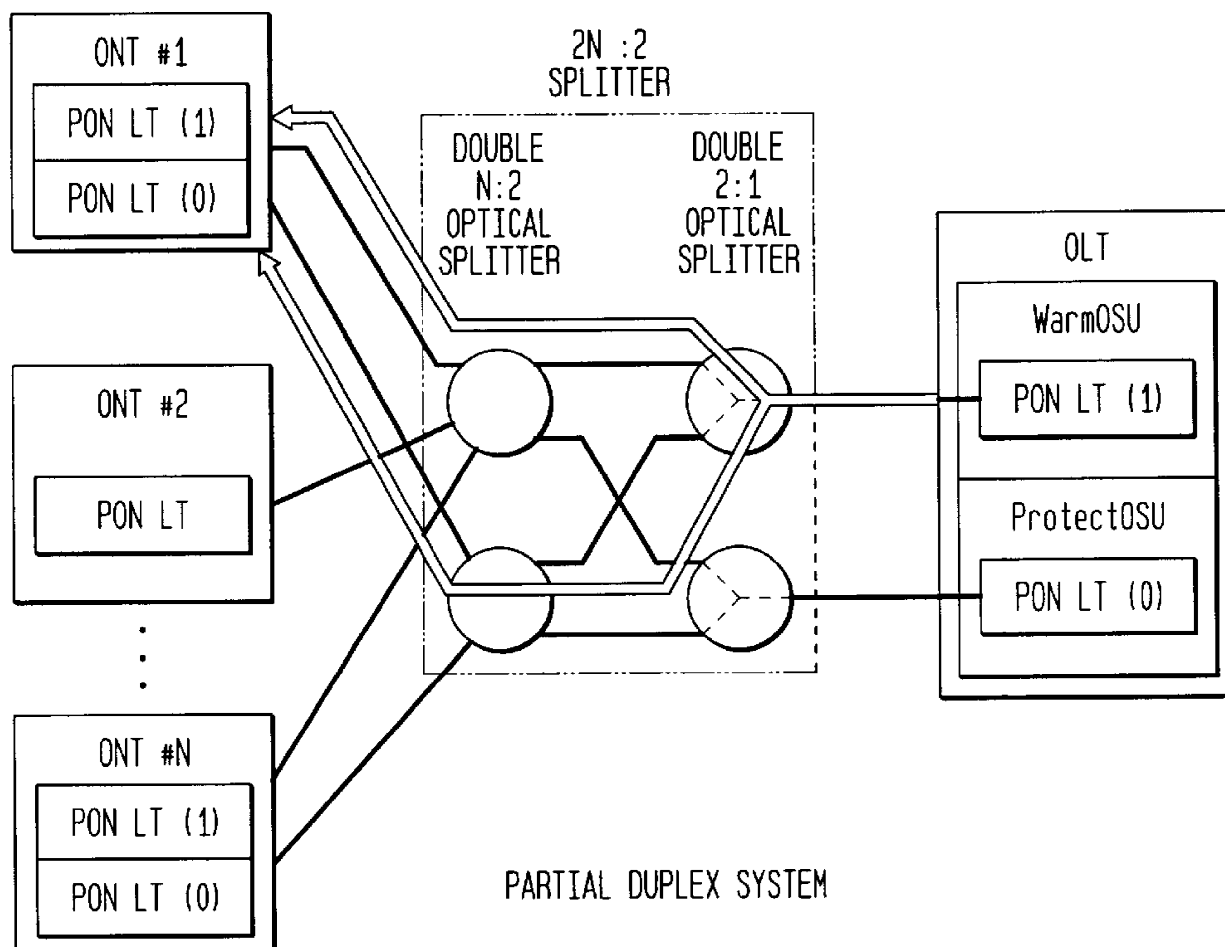
FIG. 14
