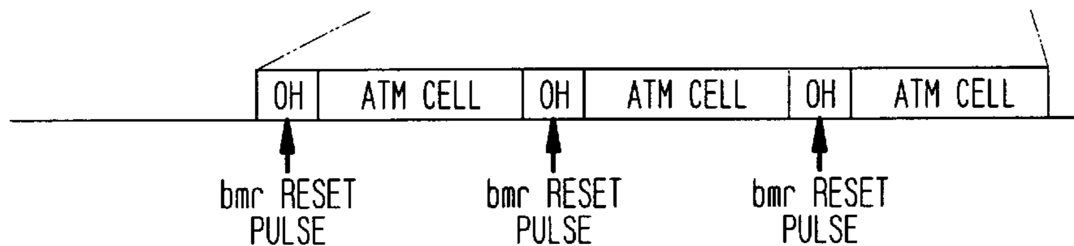
FIG. 3H
