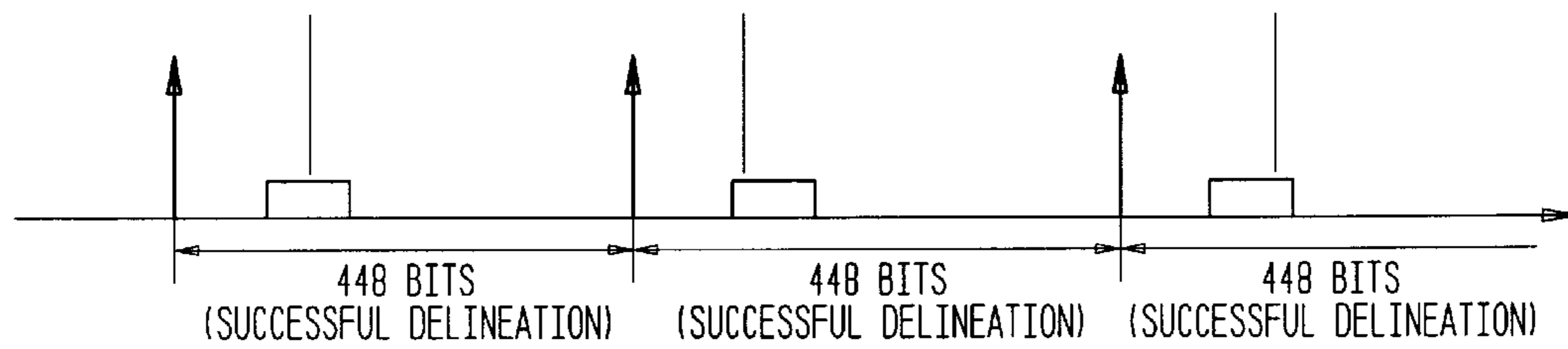
FIG. 9B
