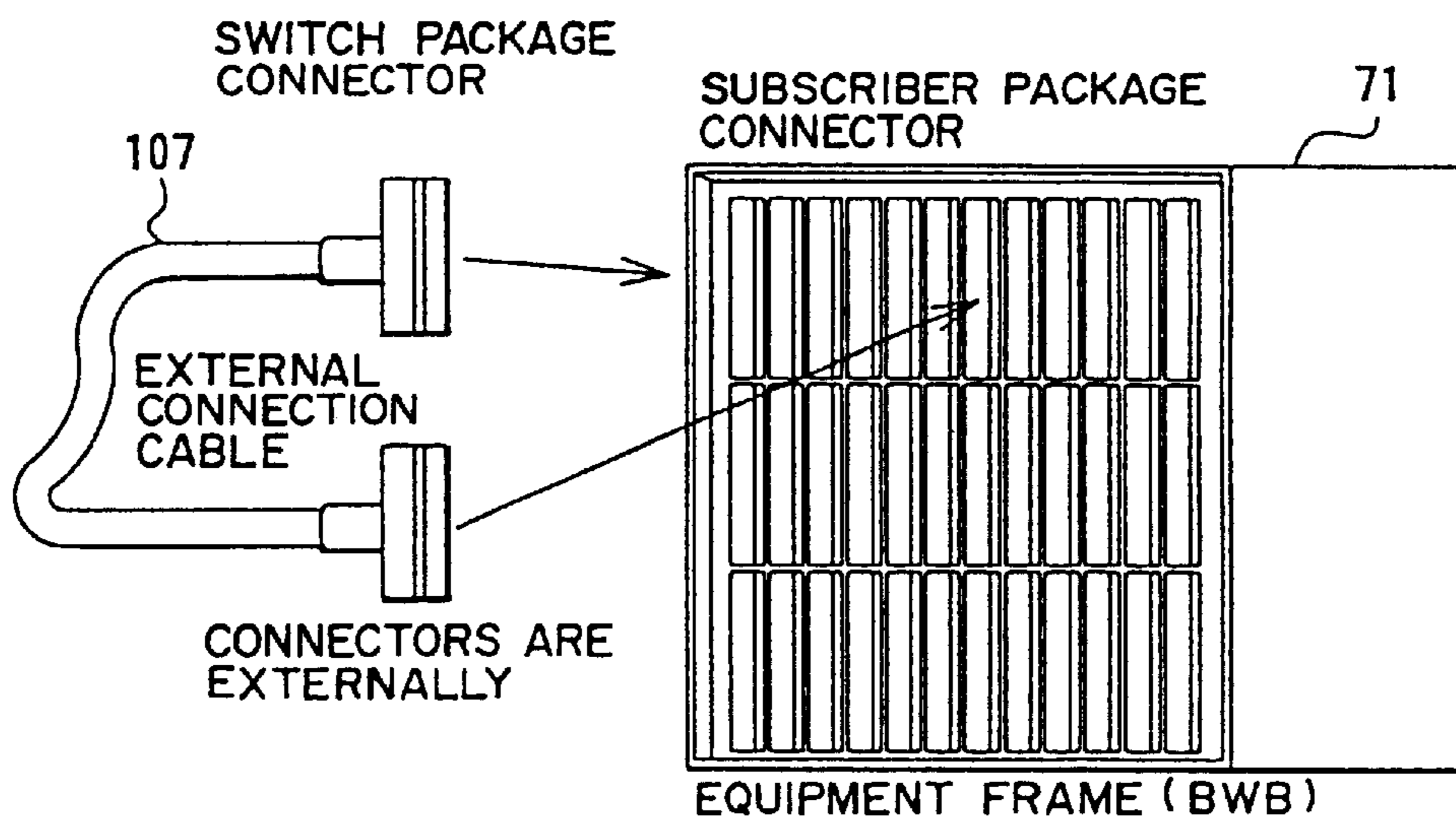
FIG. 55(b)
