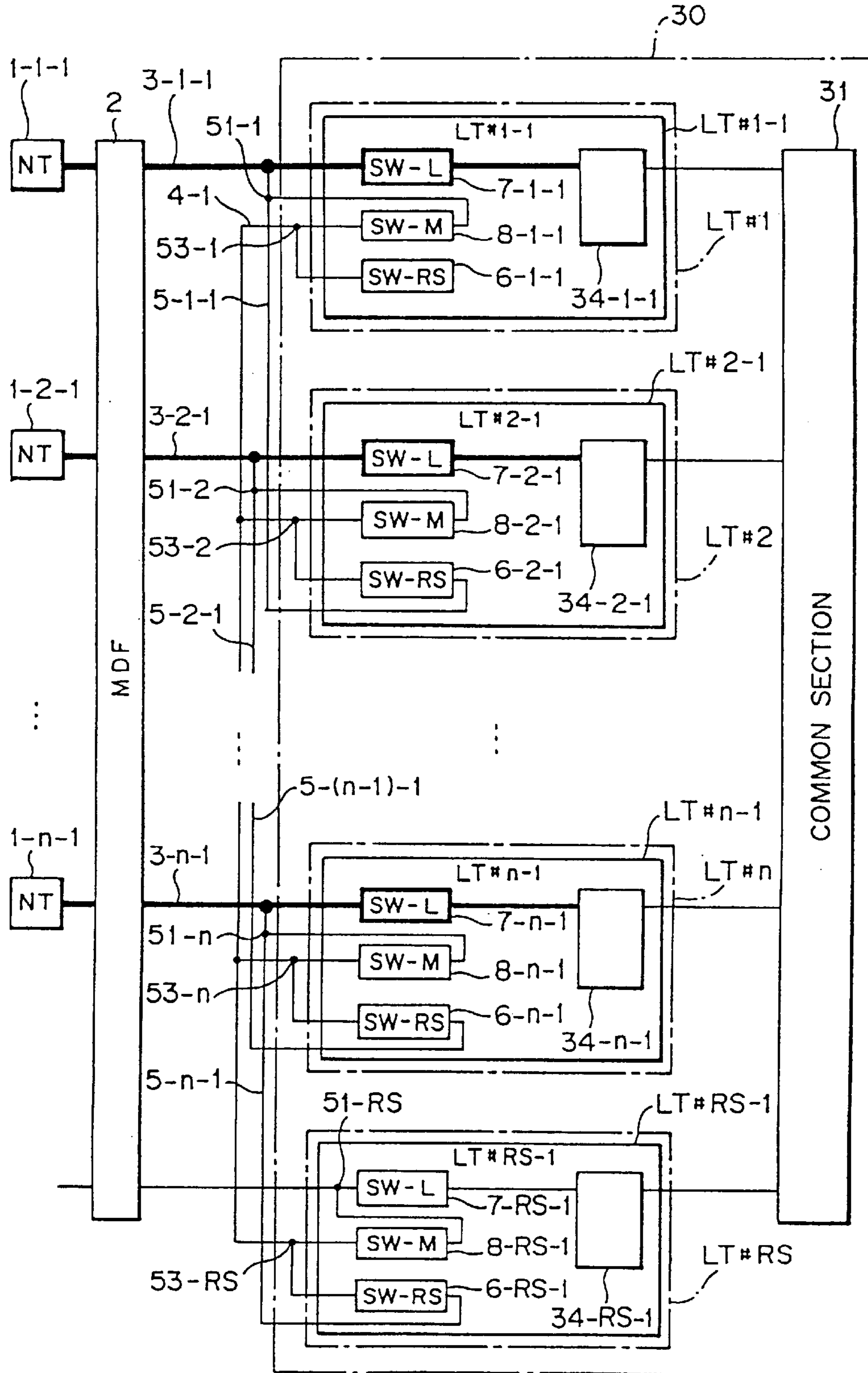
FIG. 39
