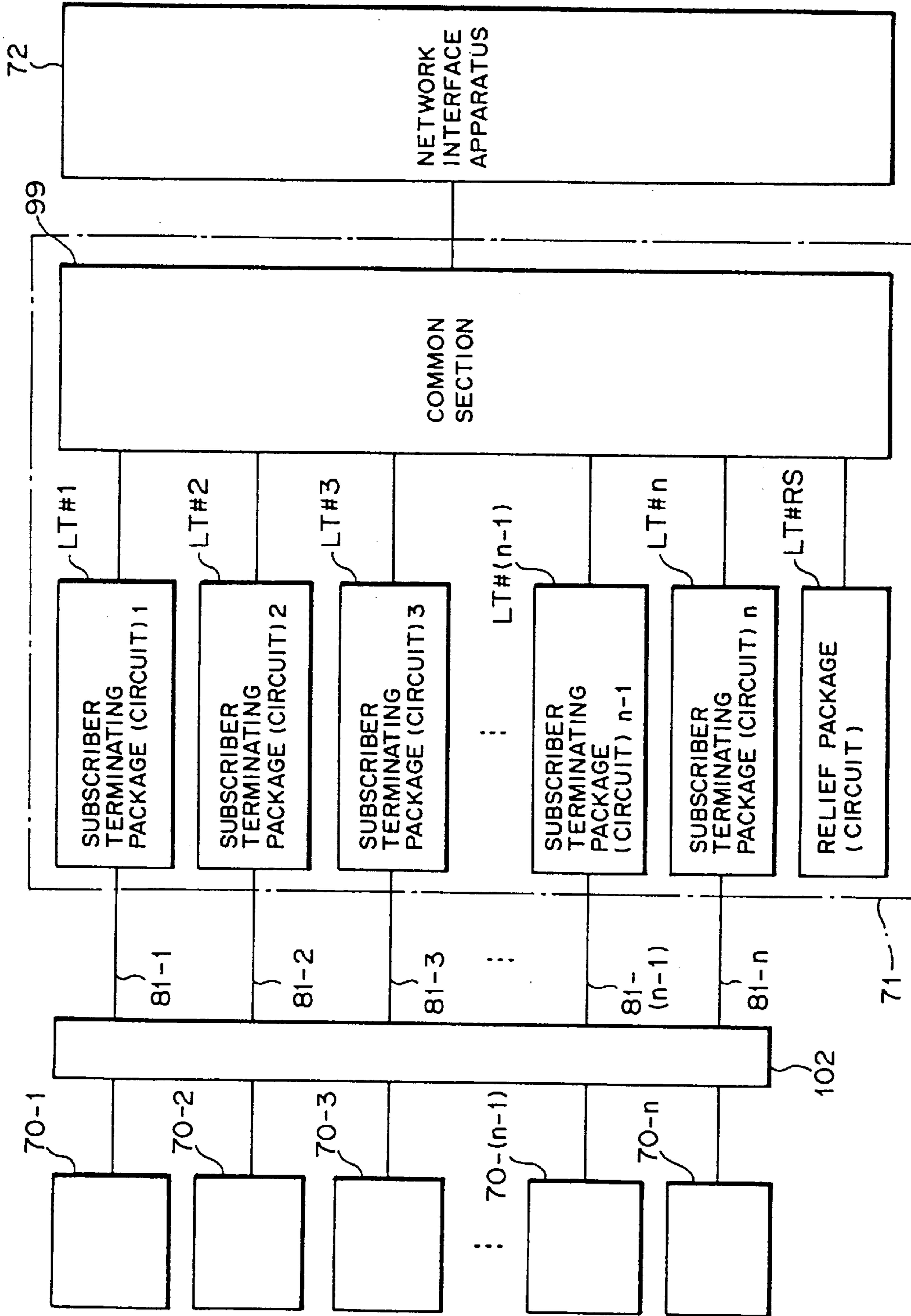
FIG. 46
