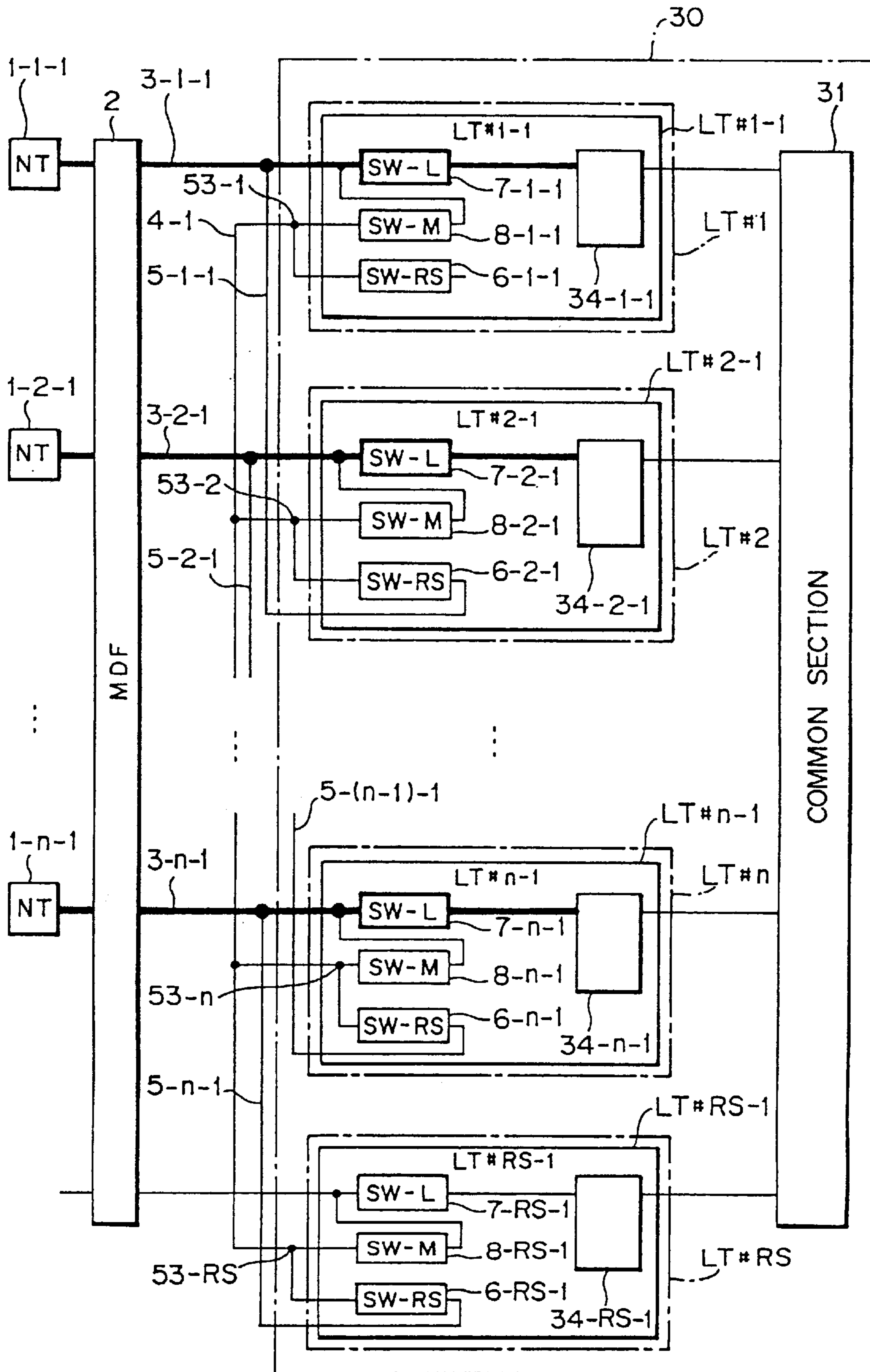
FIG. 38
