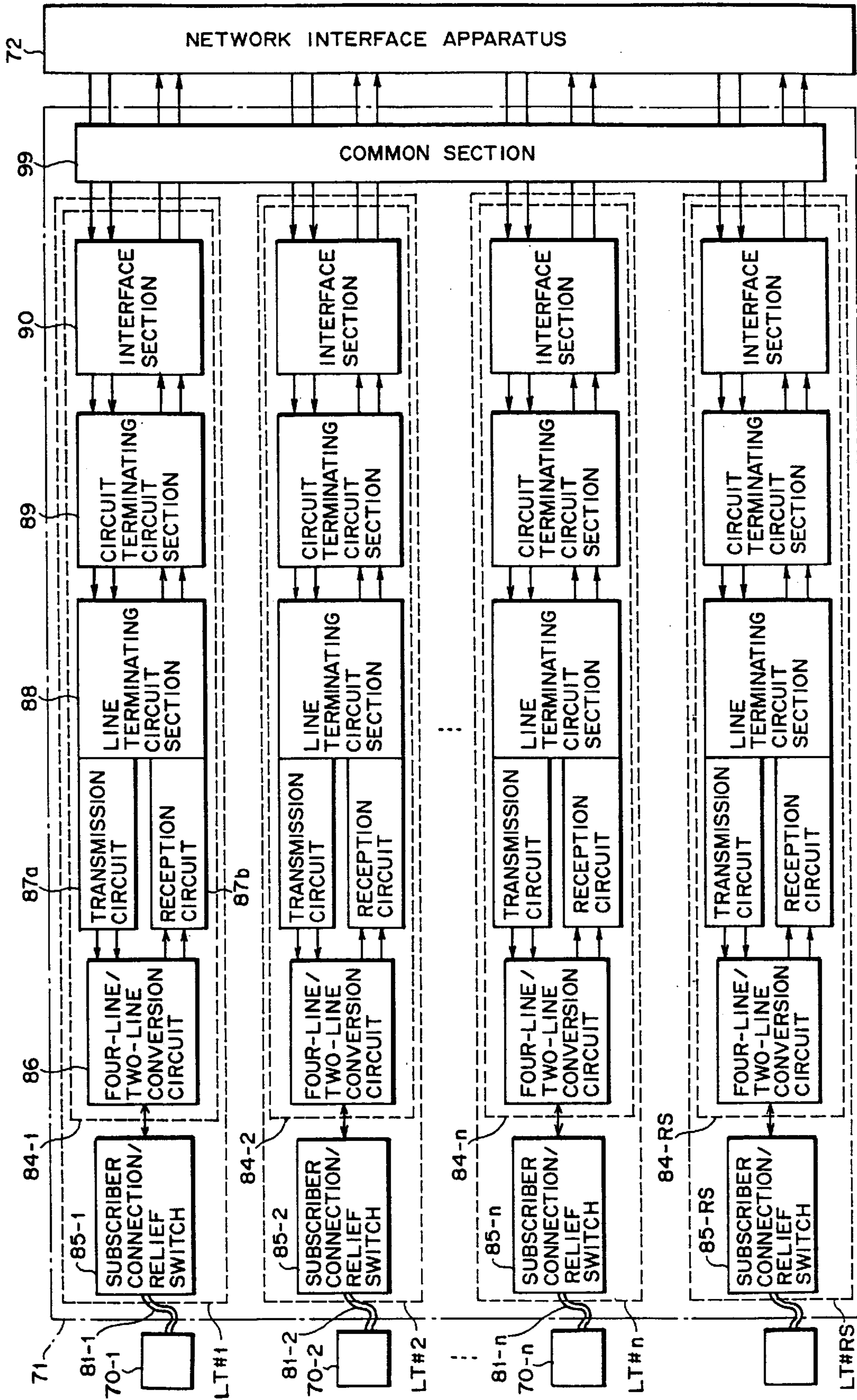
FIG. 45
