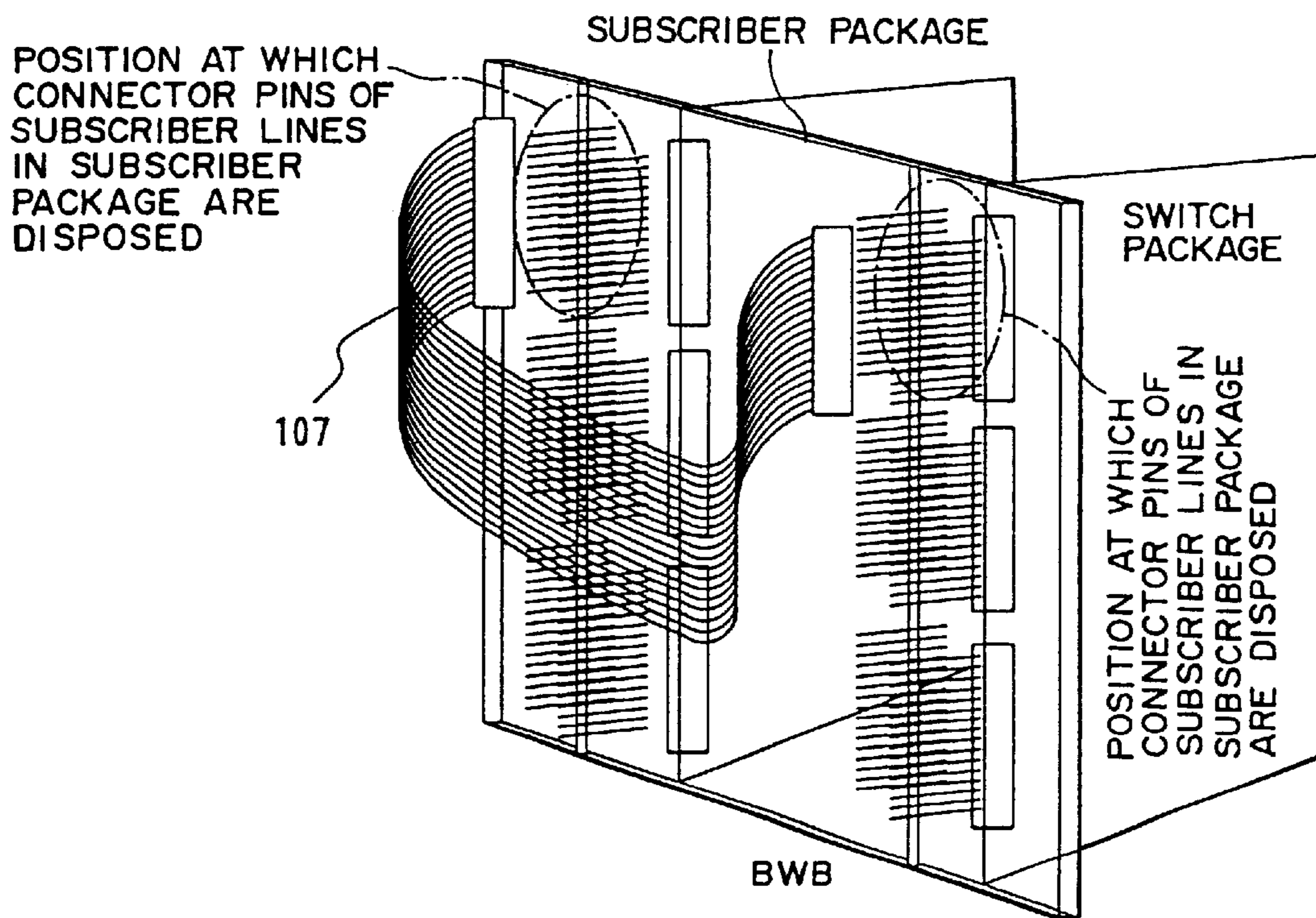
FIG. 55(b)
