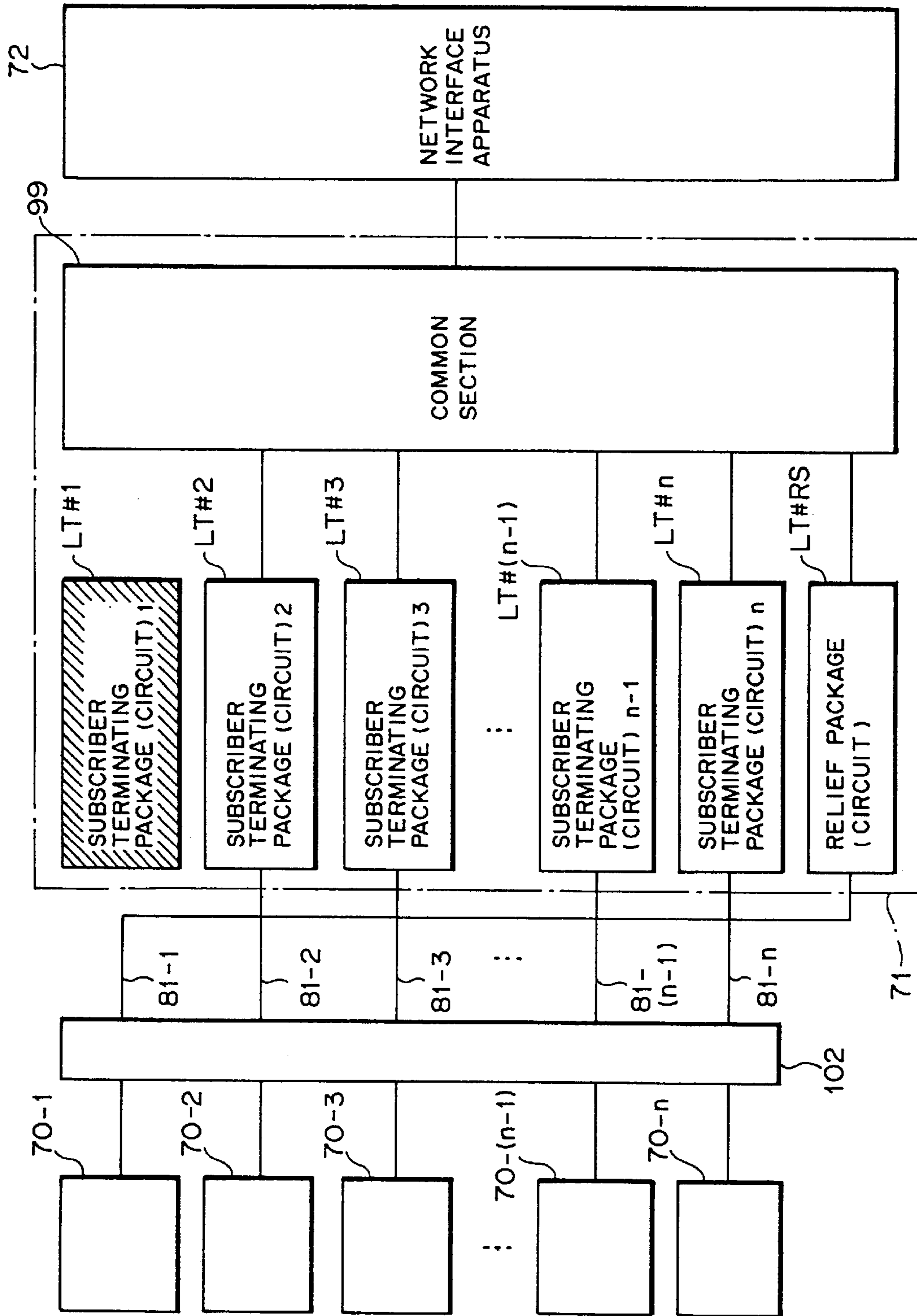
FIG. 47
