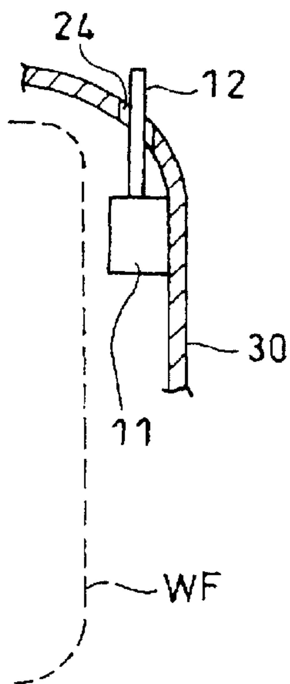
FIG. 6(a)
