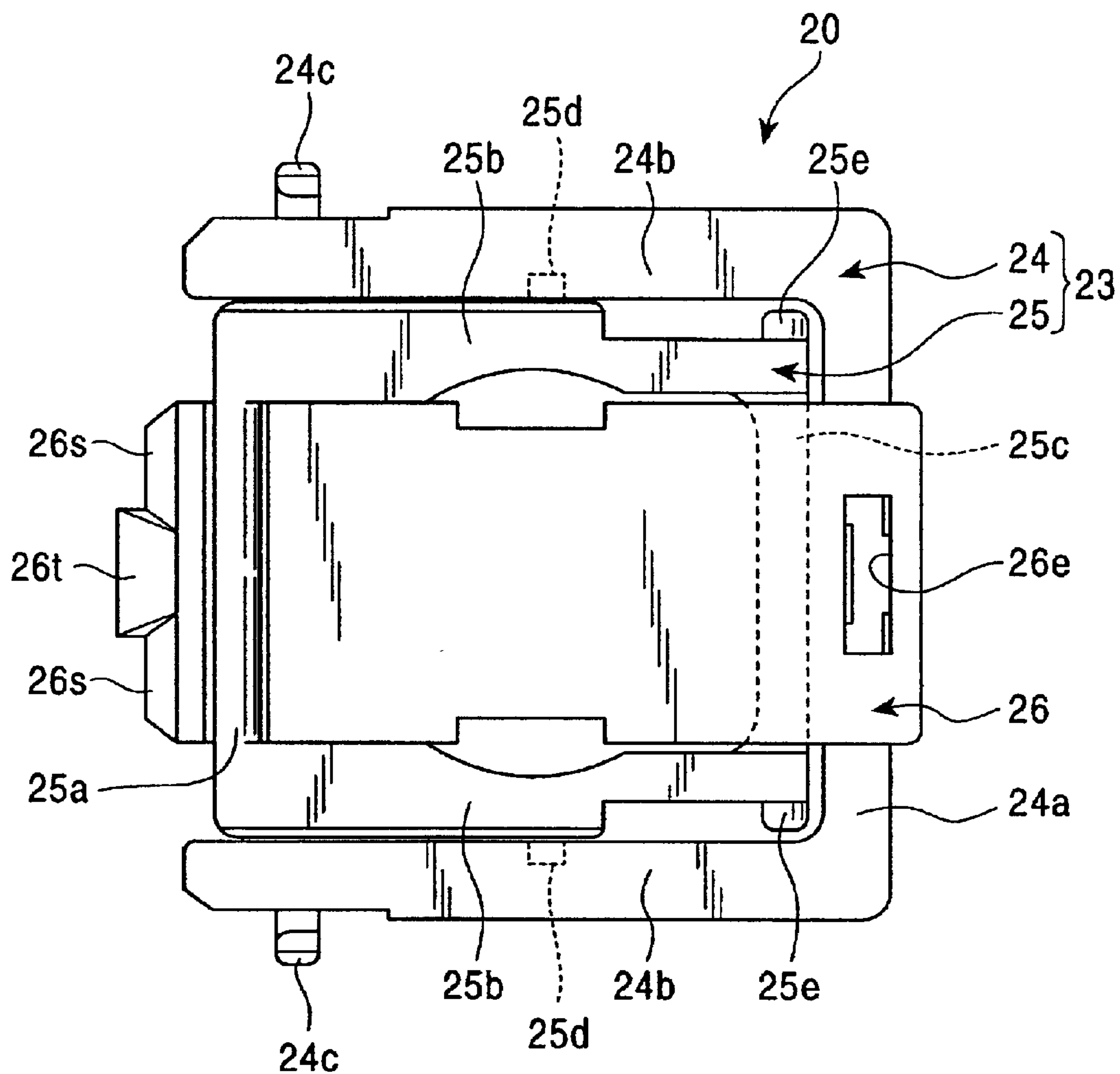
FIG. 21A
