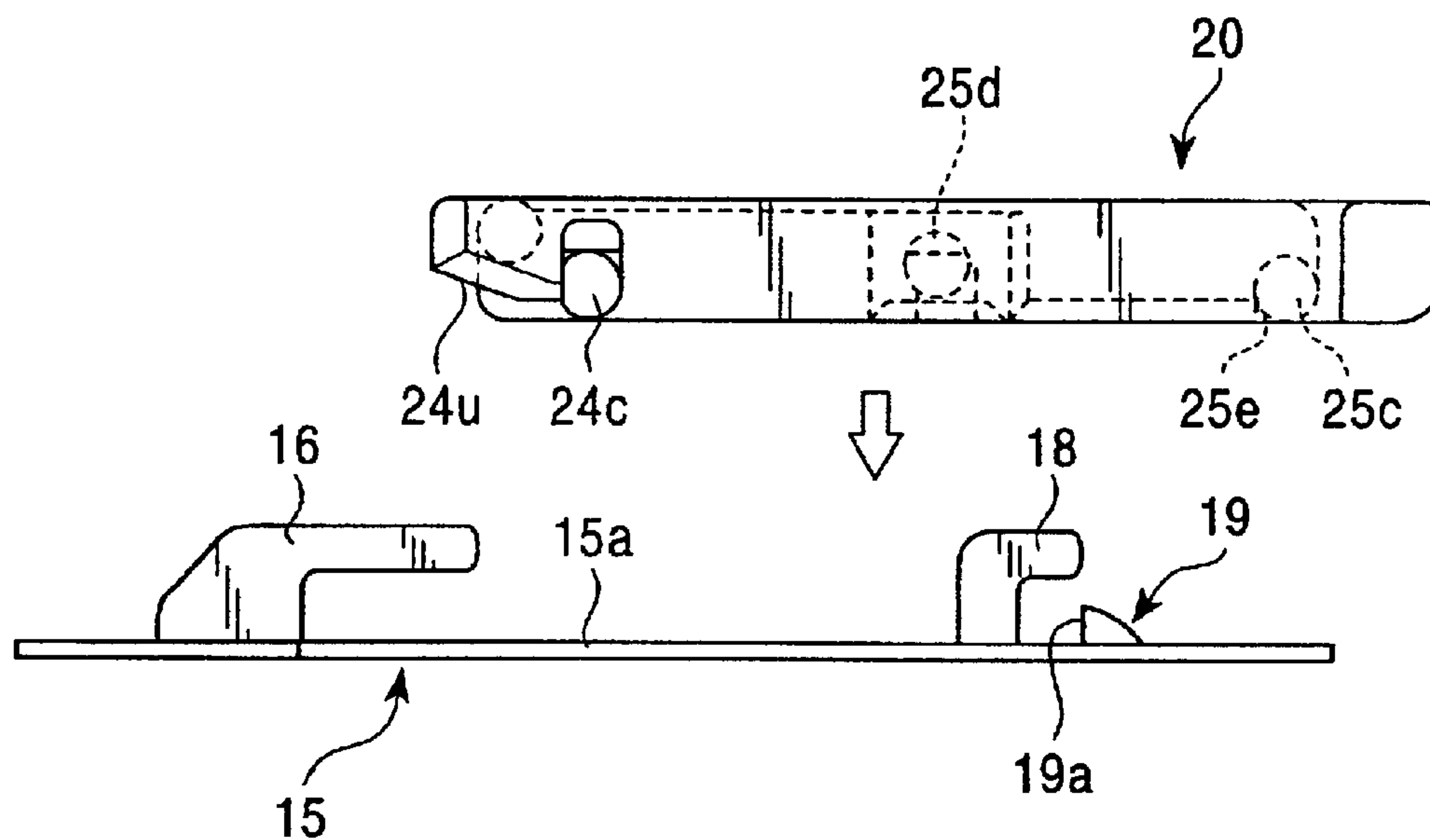
FIG. 23A
