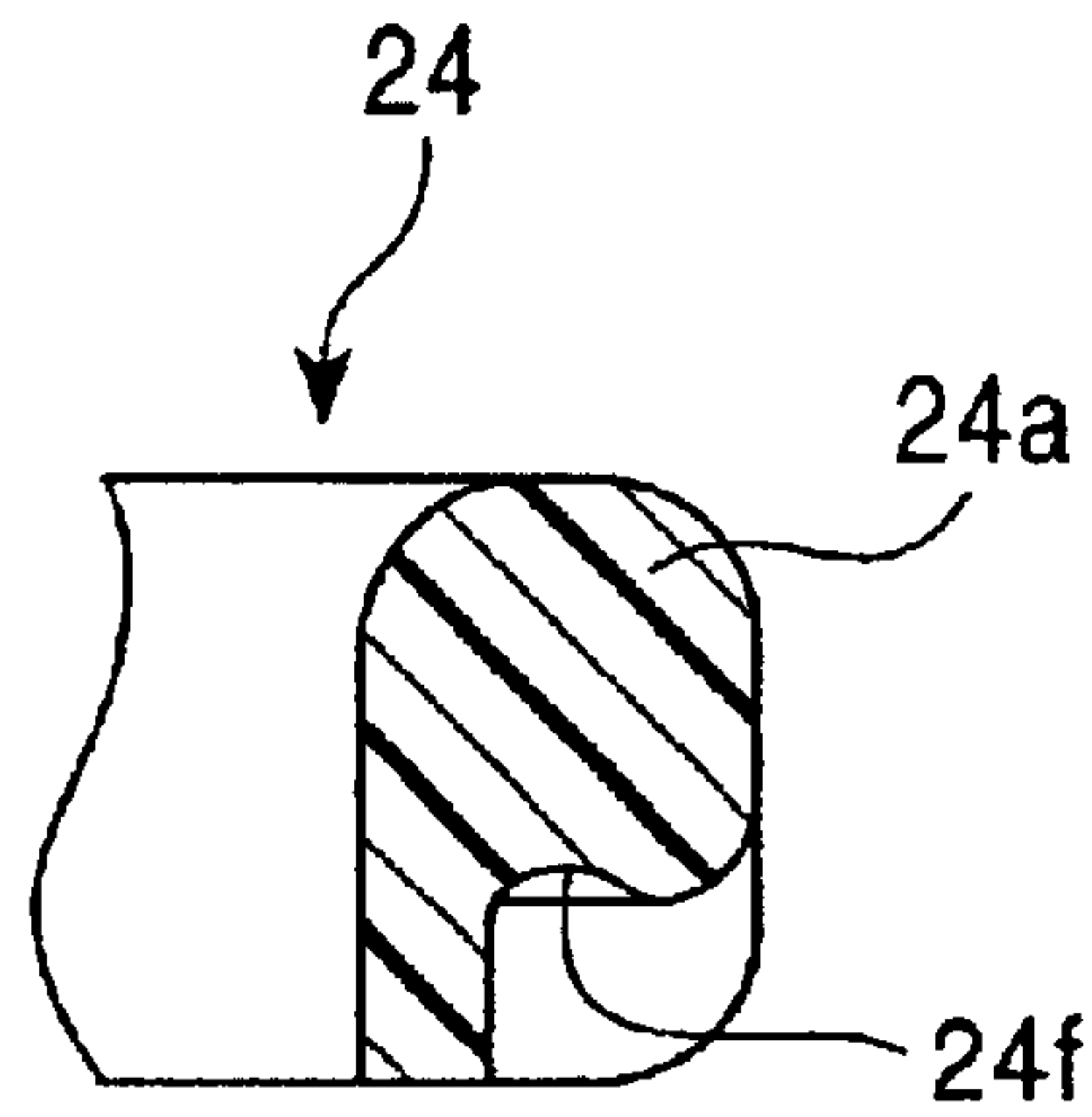
FIG. 14
