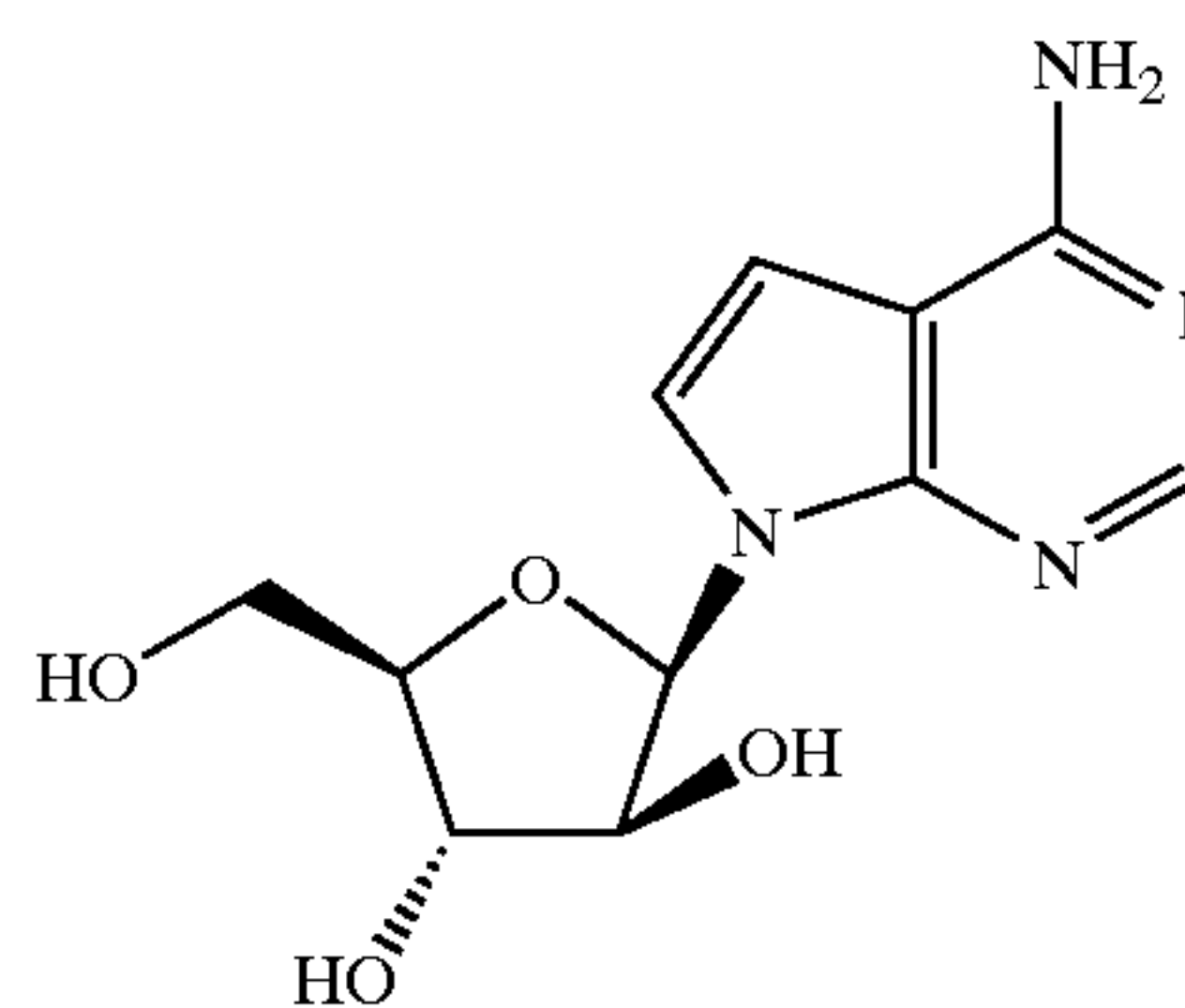
4-Amino-7-(β-D-arabinofuranosyl)-7H-pyrrolo[2,3- d]pyrimidine
