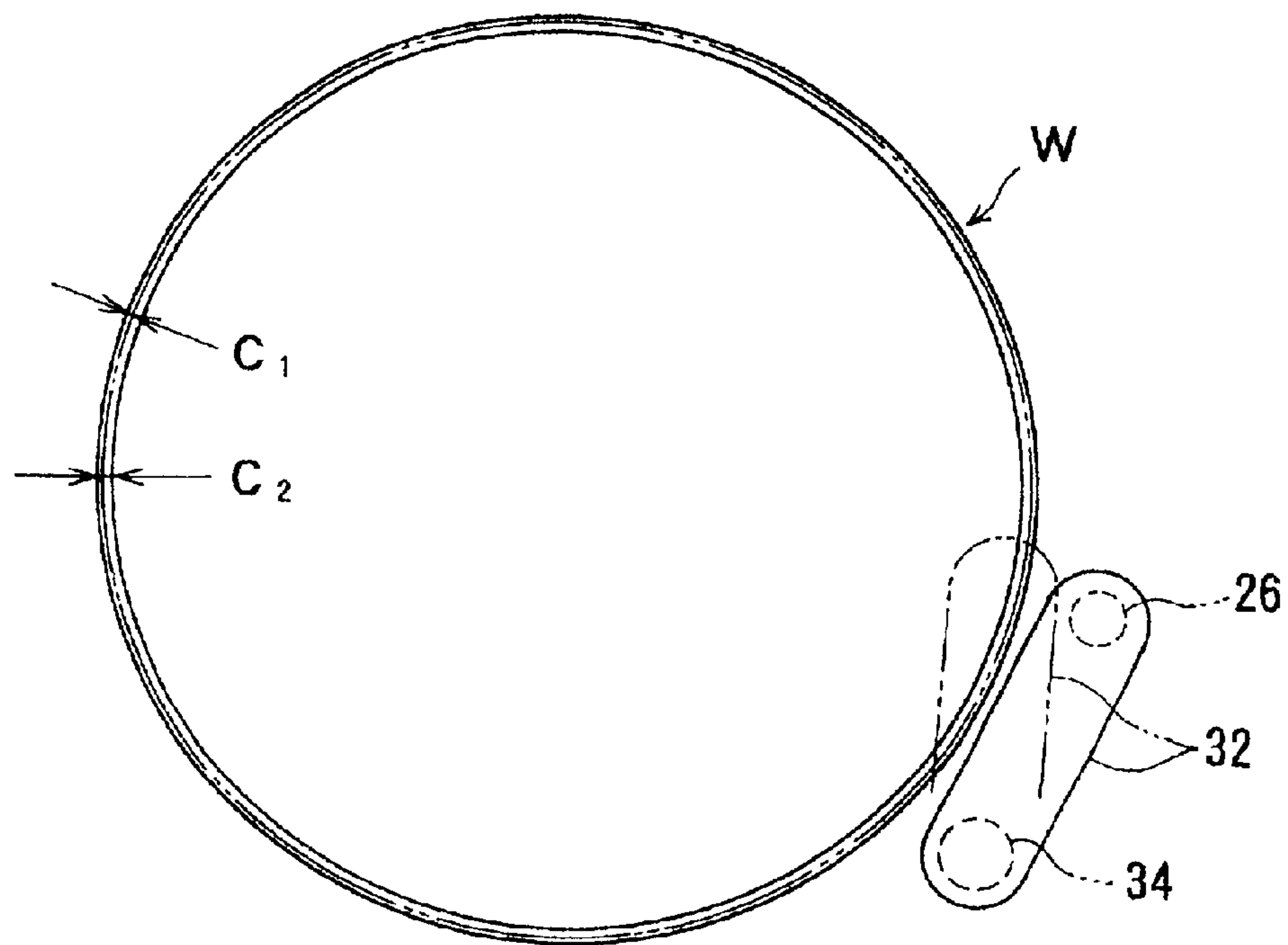
FIG. 10
