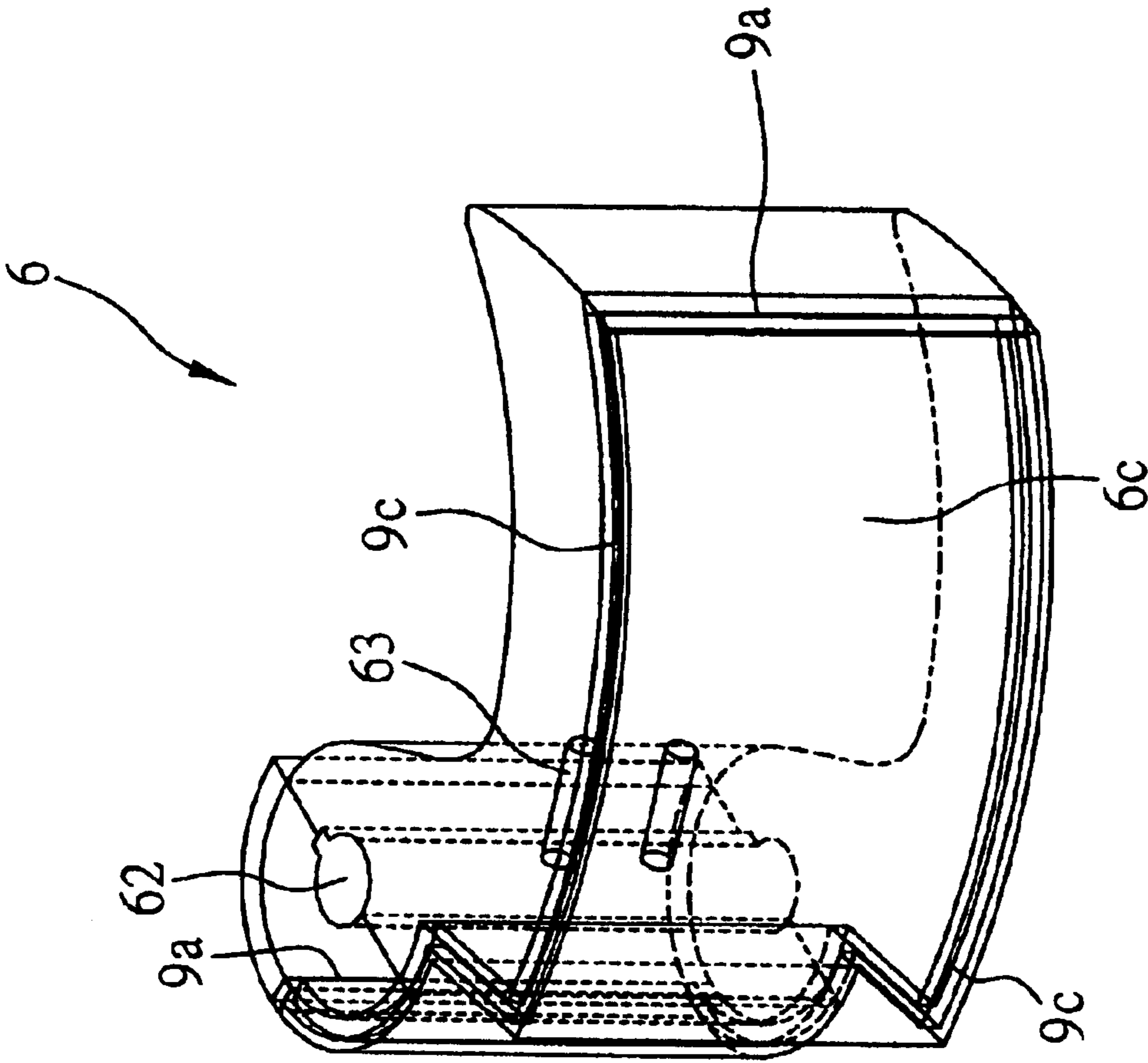
FIG. 9A
