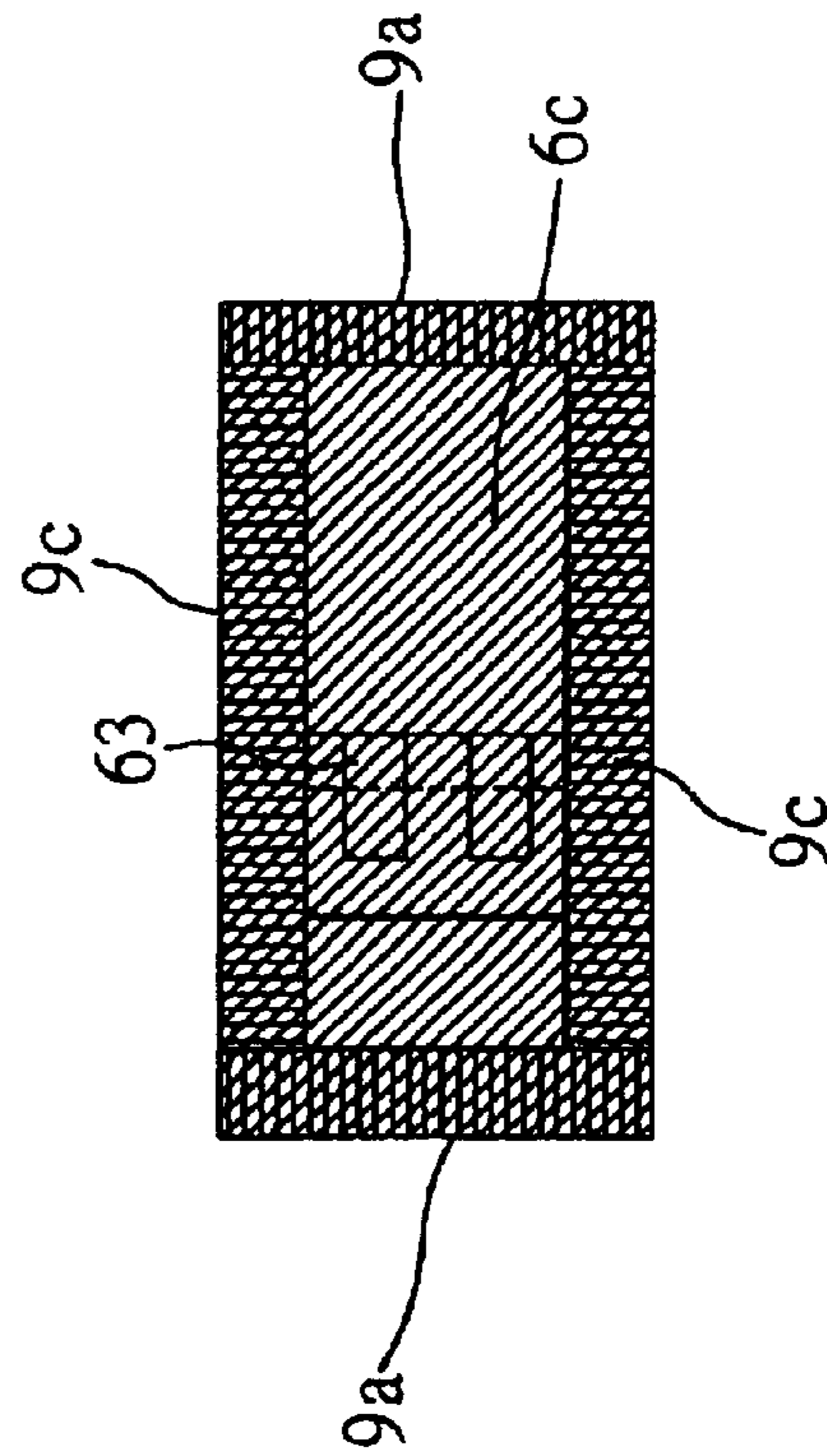
FIG. 9B
