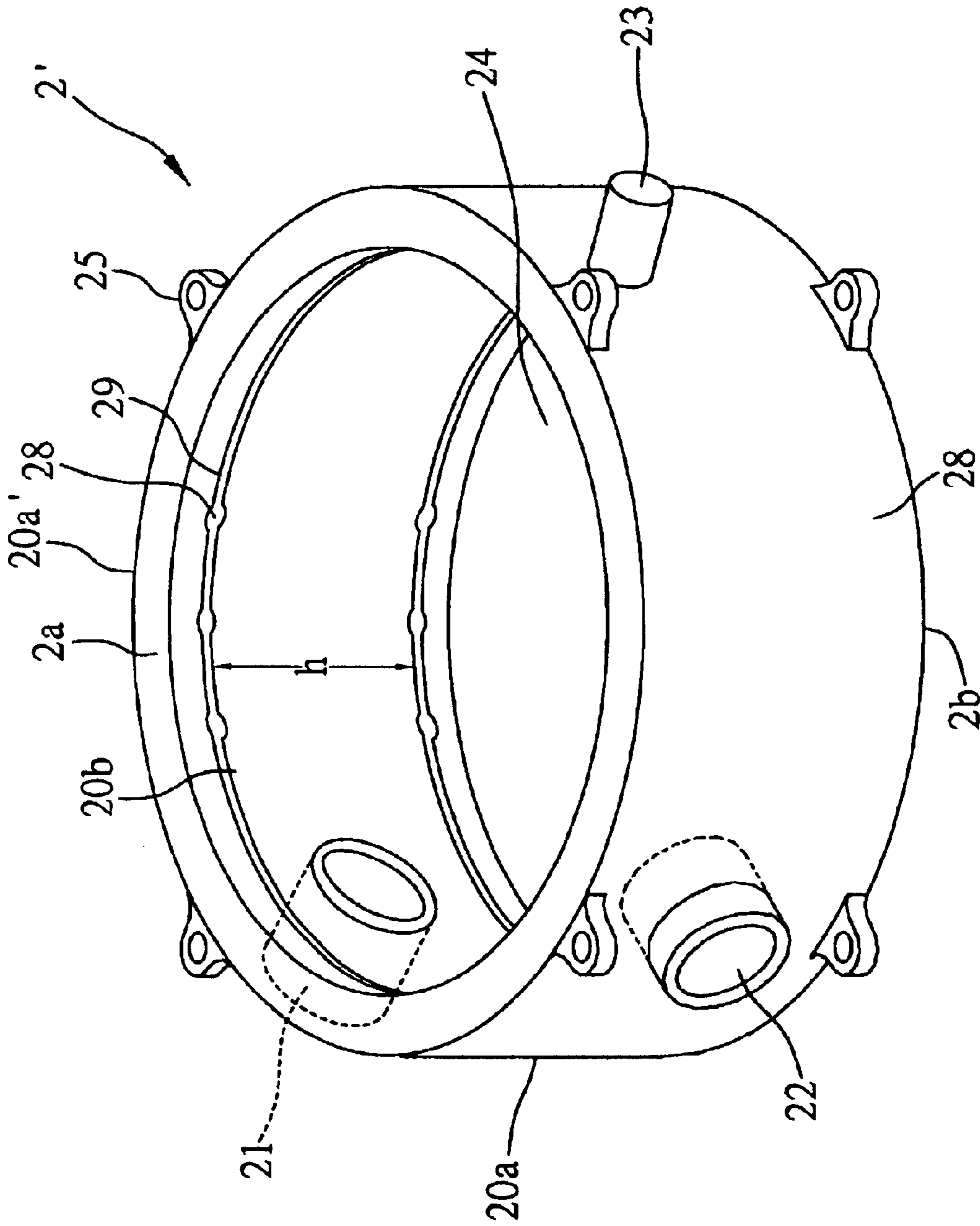
FIG. 18
