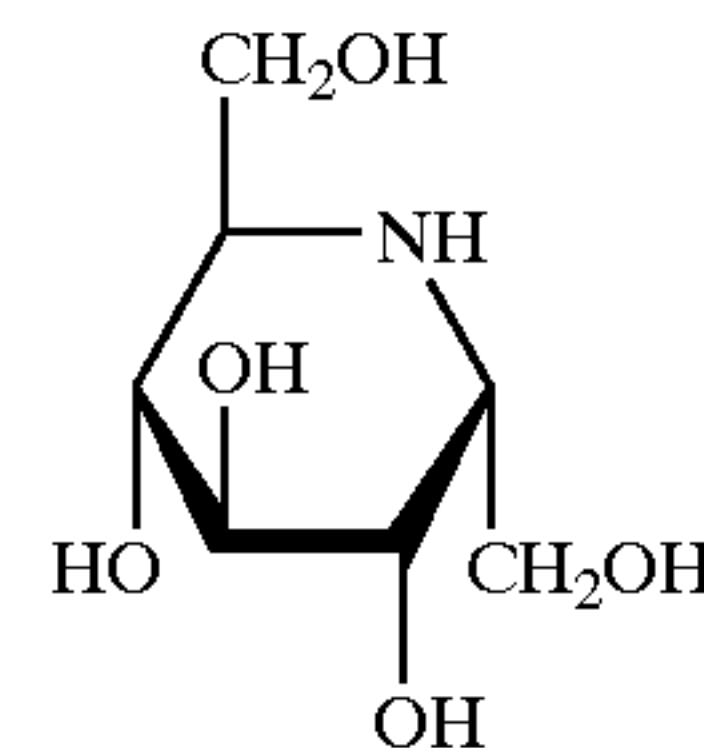
\alpha -Homonojirimycin
