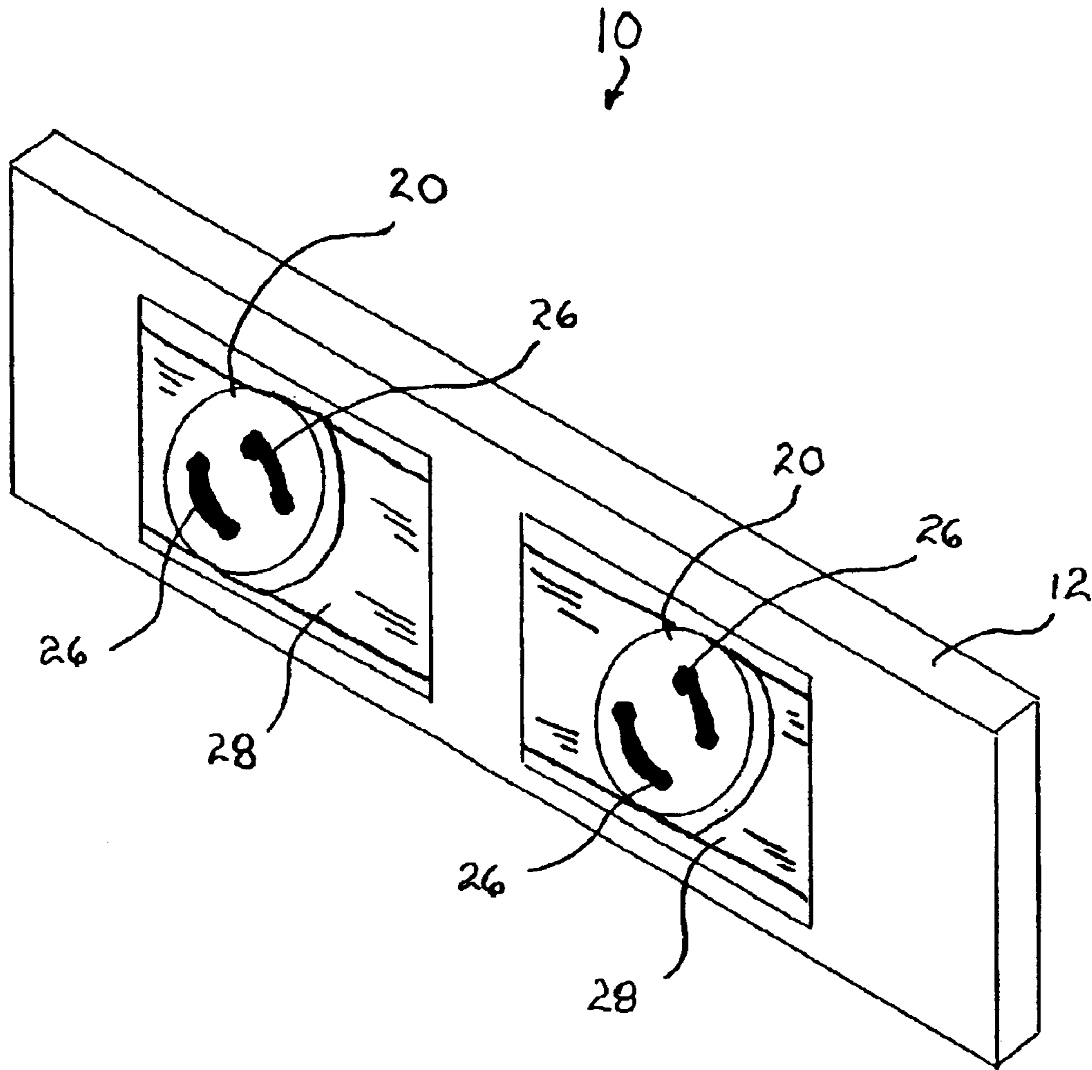
Fig. 4
