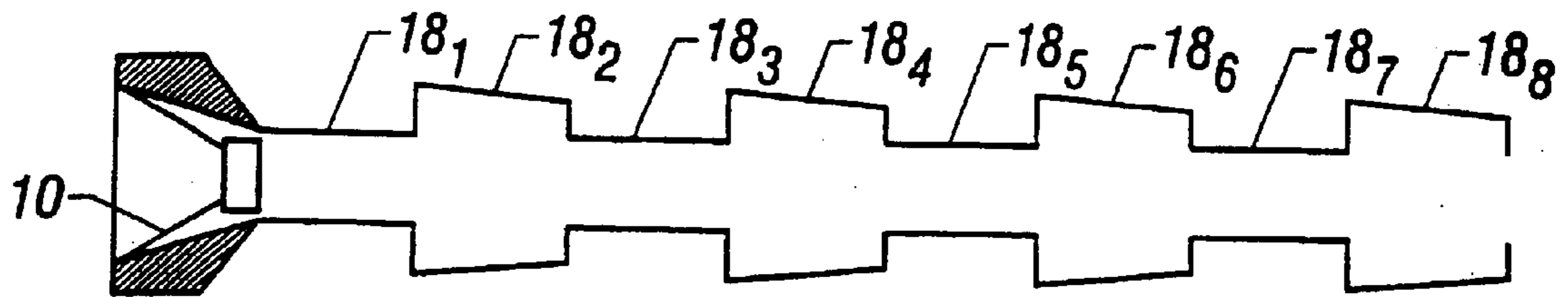
FIG. 14B
