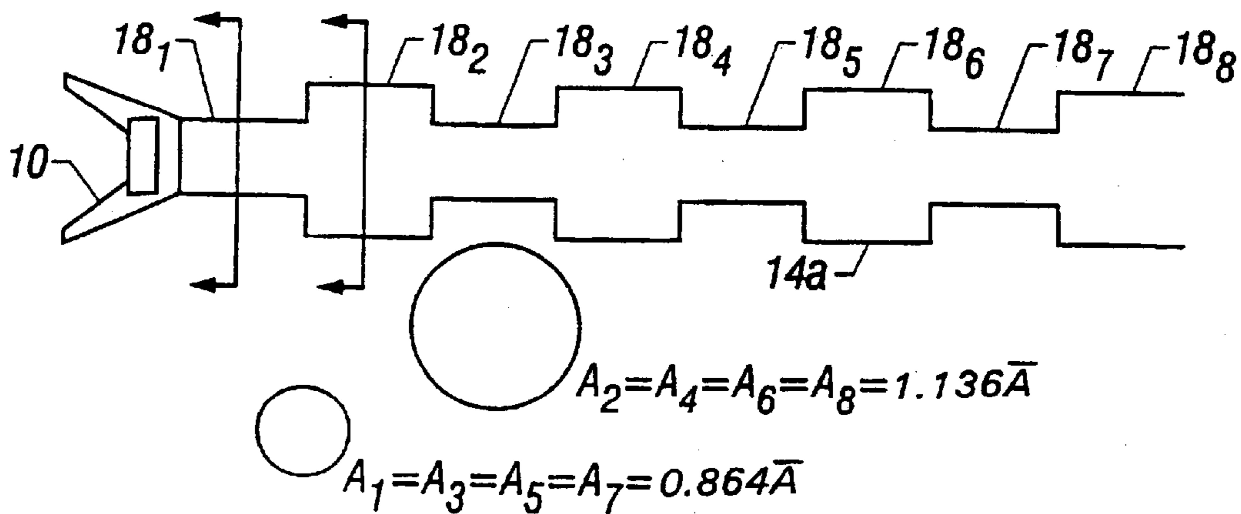
FIG. 6A
