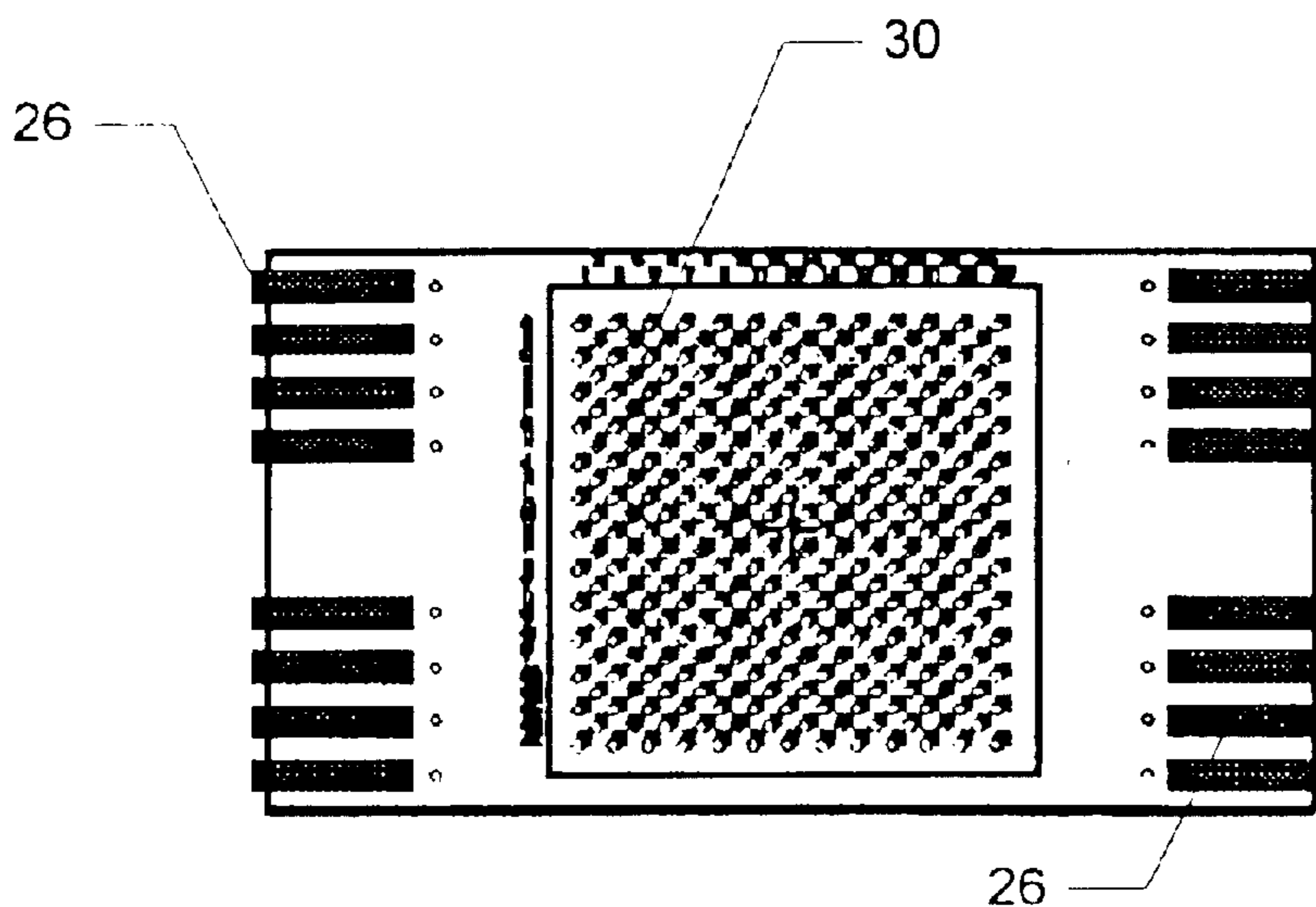
BOTTOM Layer 18
