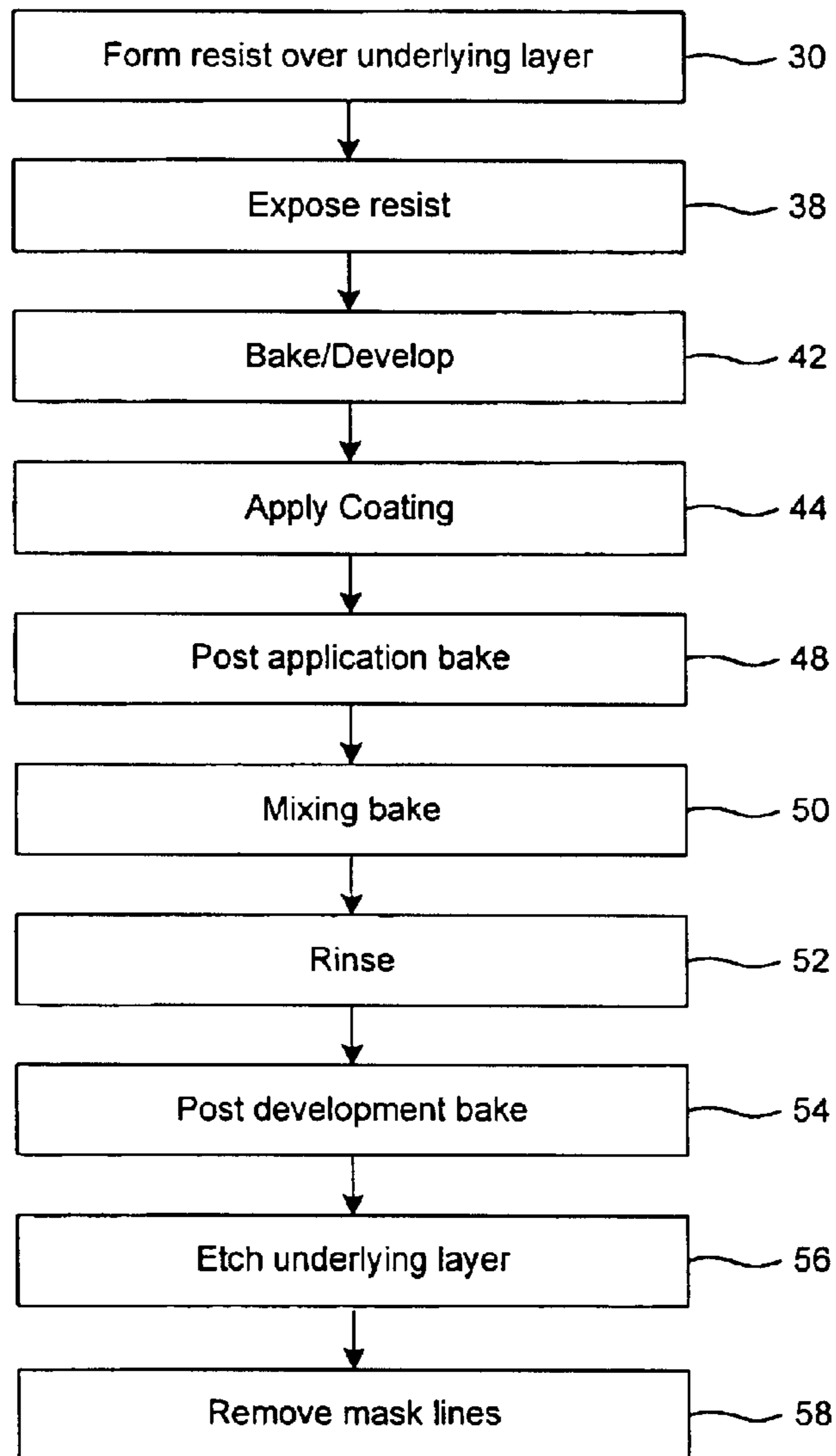
FIG. 2
