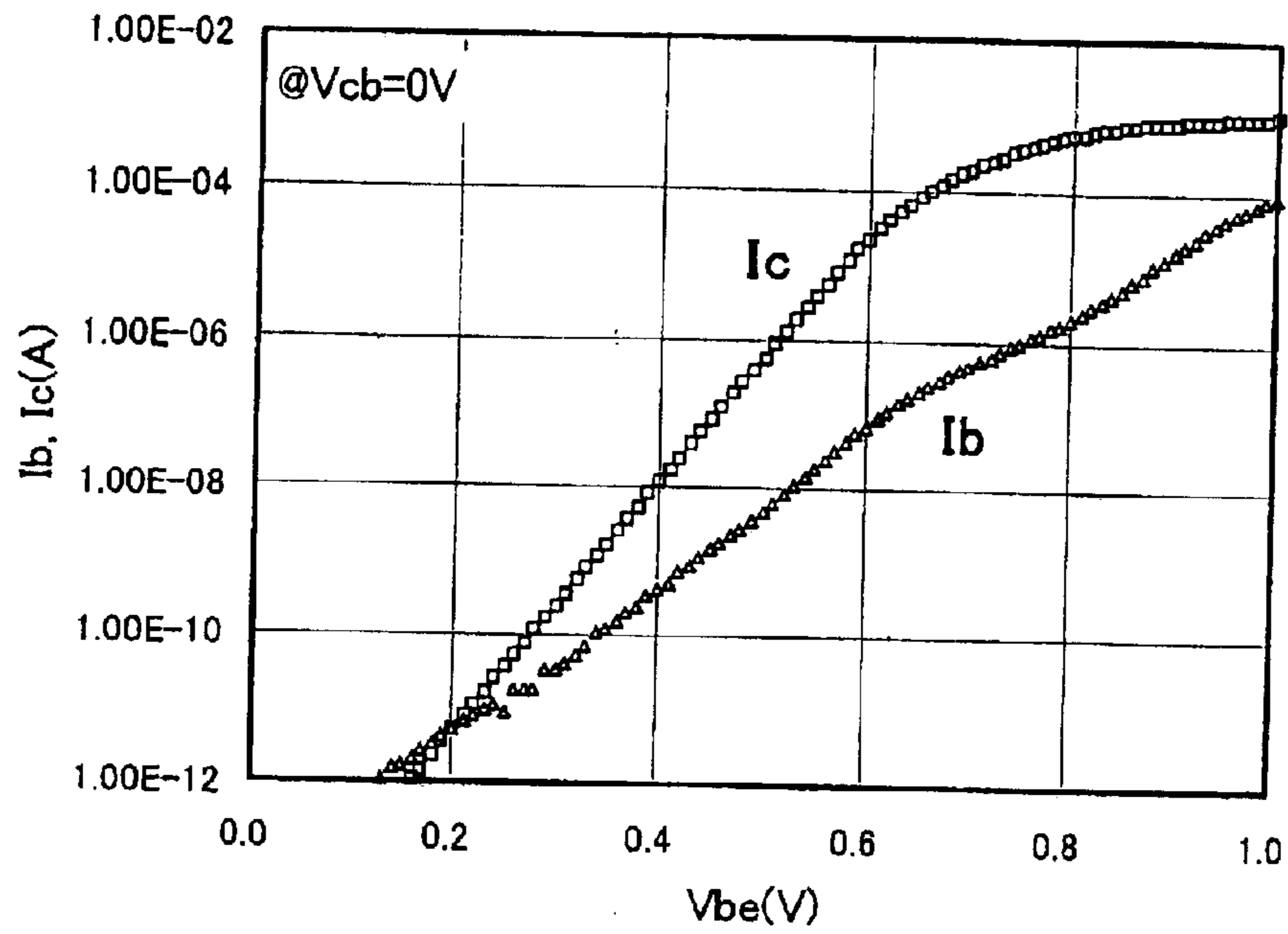
SiGe 0.268 HBT Gummel plot
