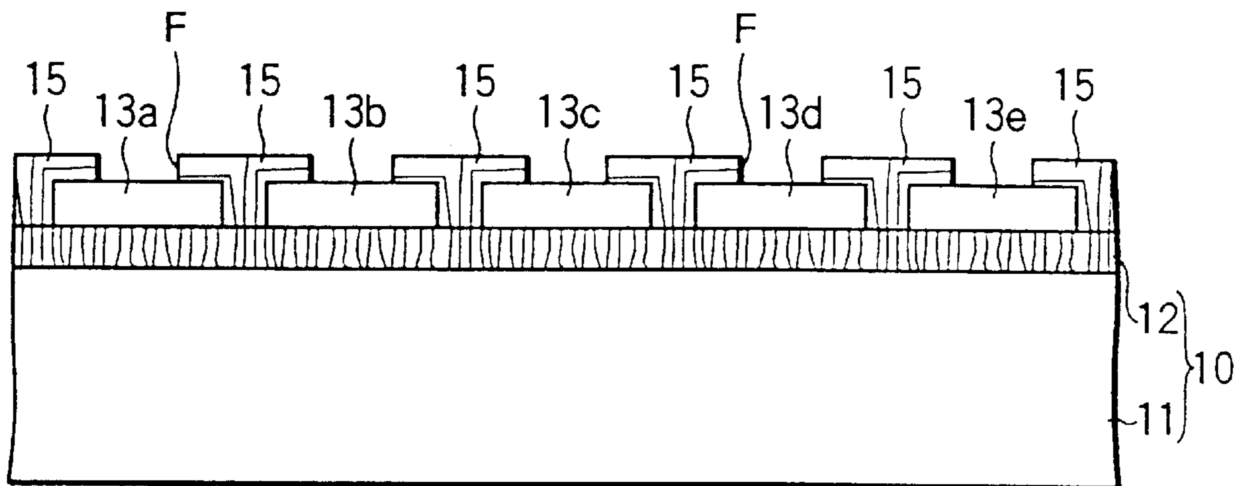
FIG. 1B
