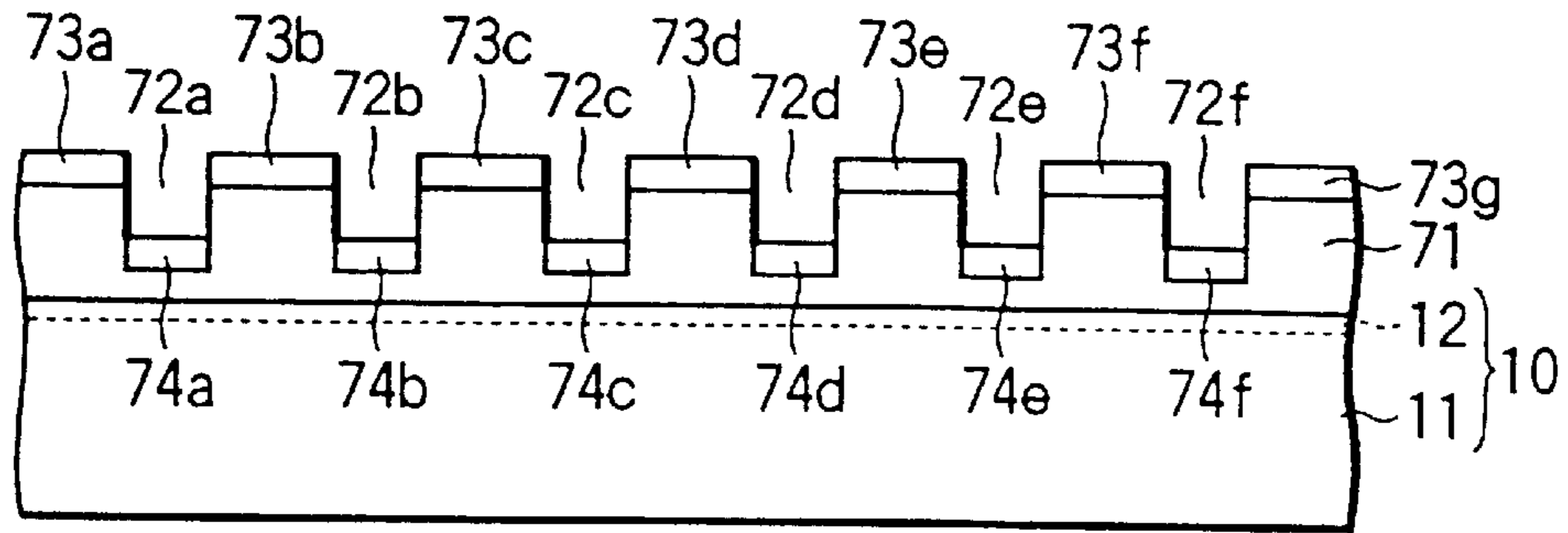
FIG. 7B
