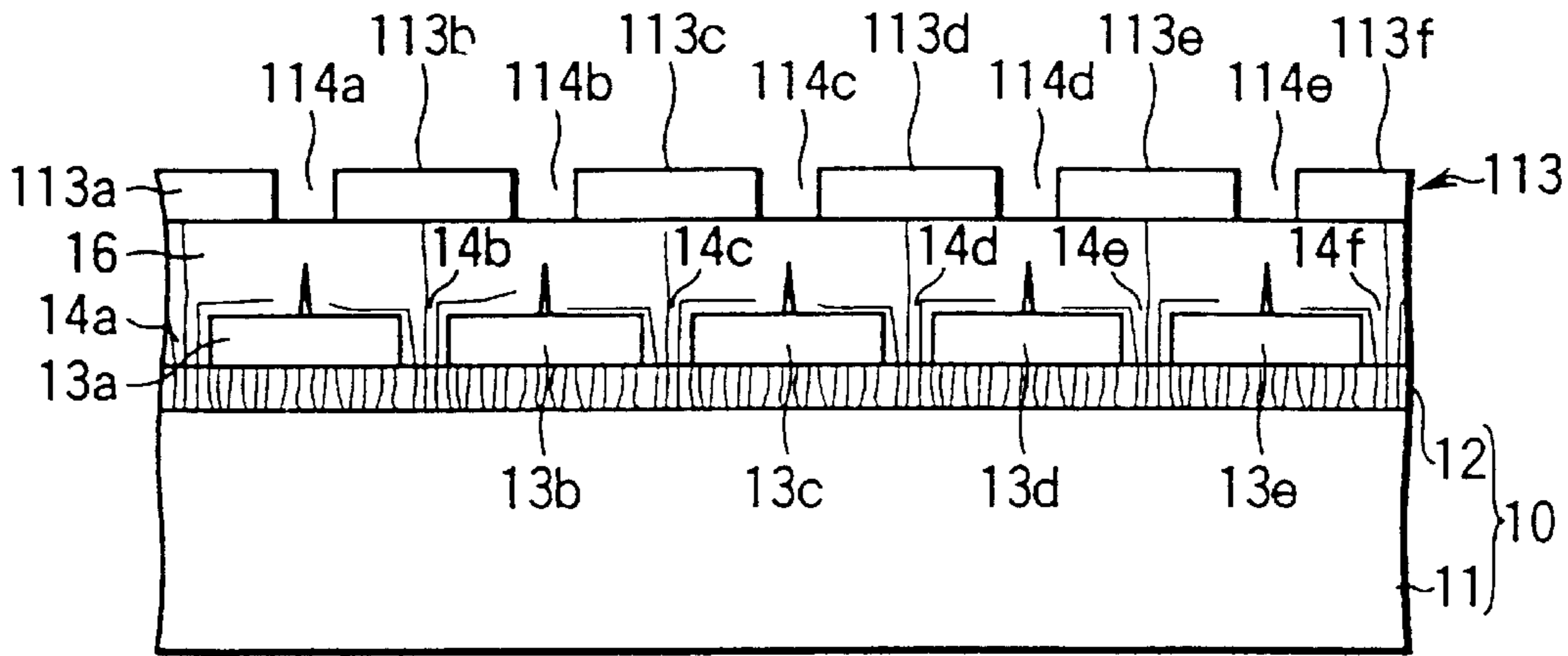
FIG. 6A
