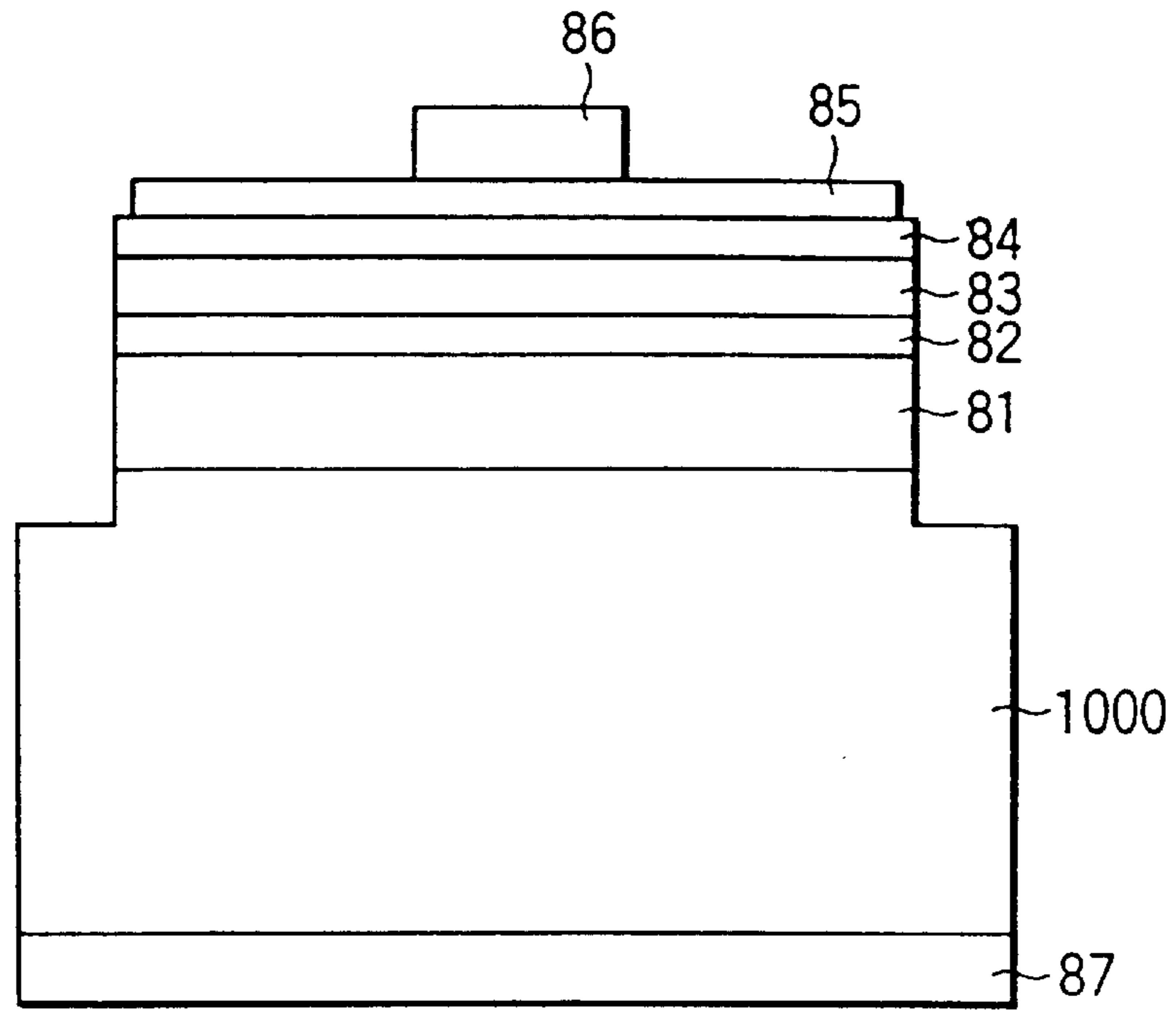
FIG. 8A
