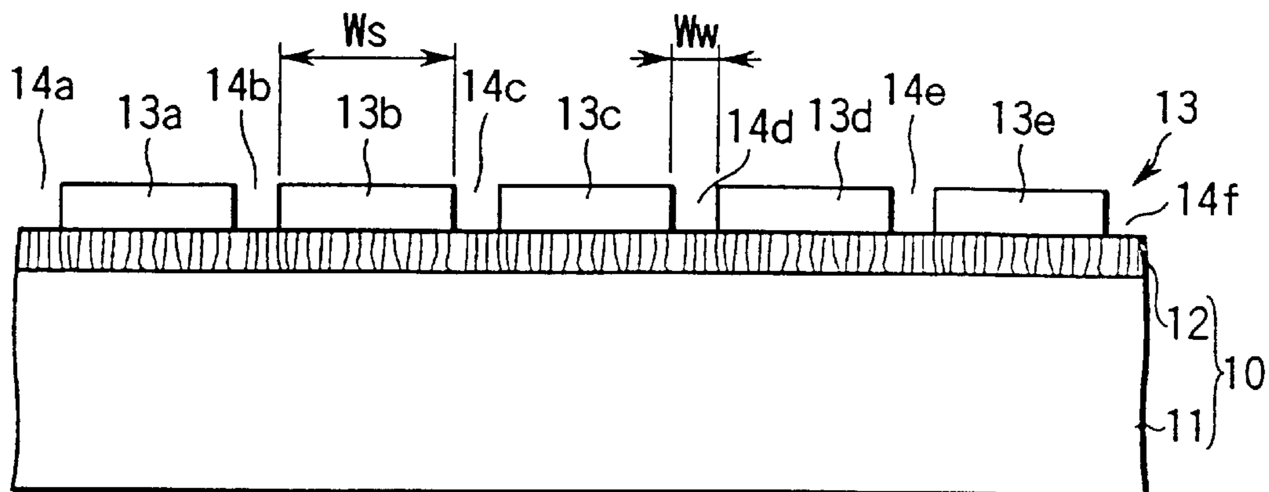
FIG. 1A
