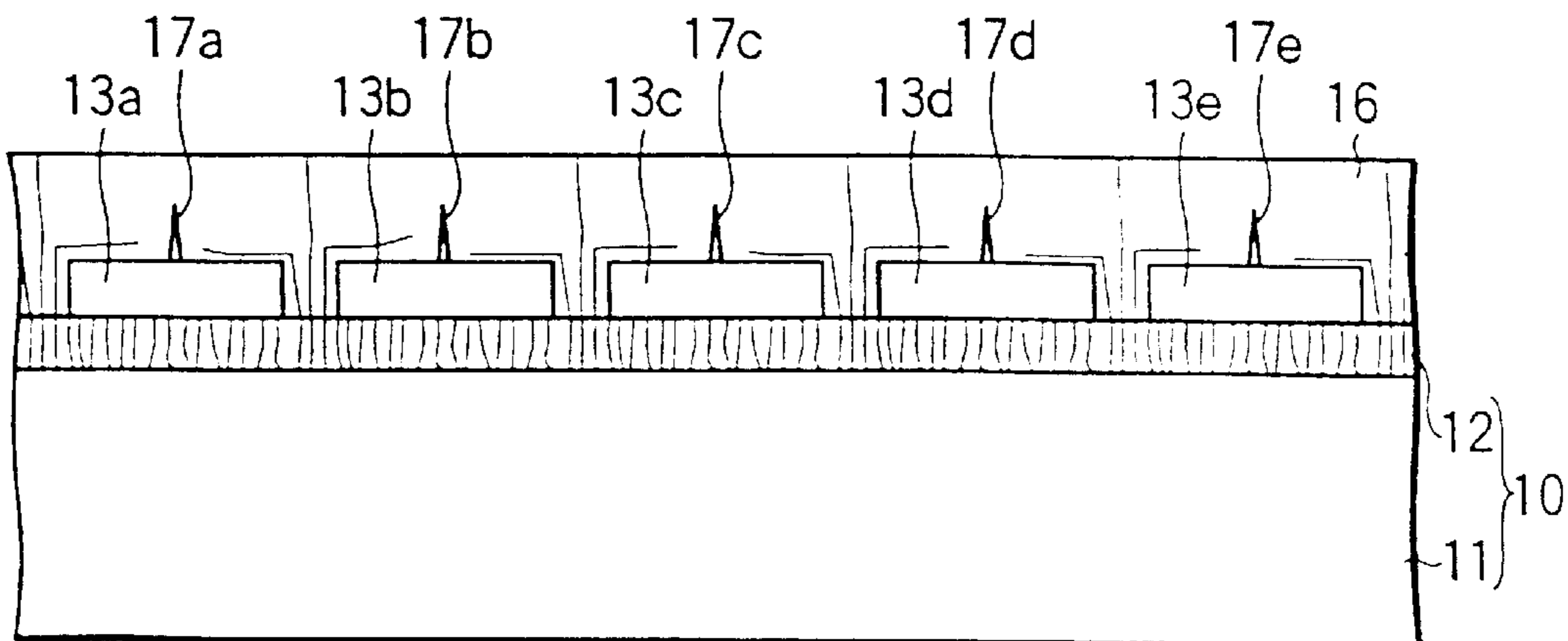
FIG. 1C
