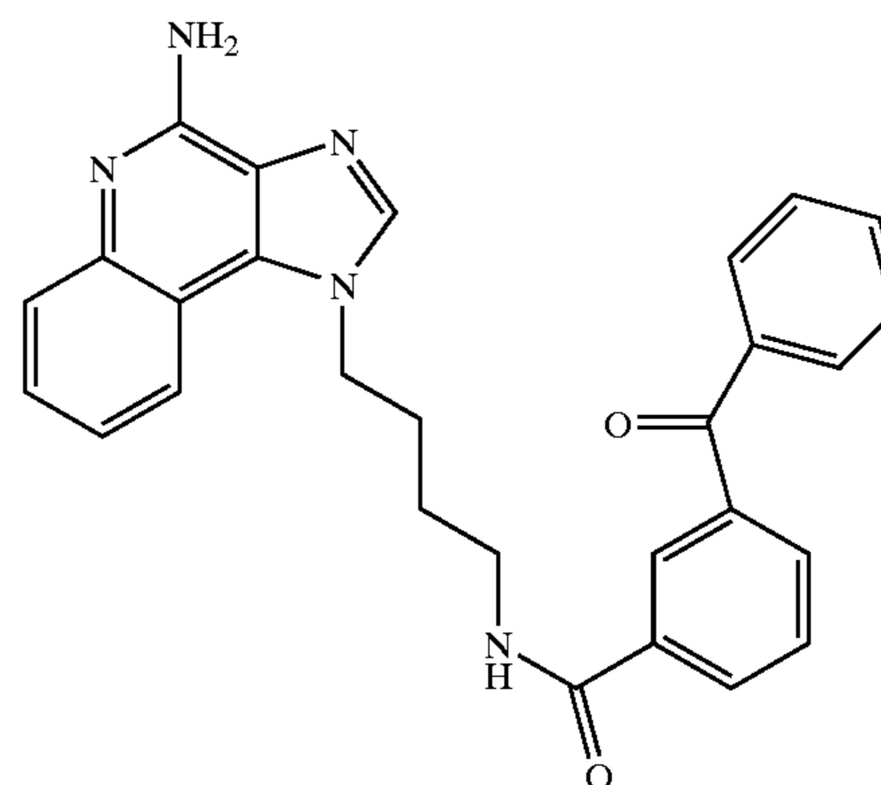
N 1 -[4-(4-Amino-1H-imidazo[4,5-c]quinolin-1-yl)butyl]-3-benzoylbenzamide
