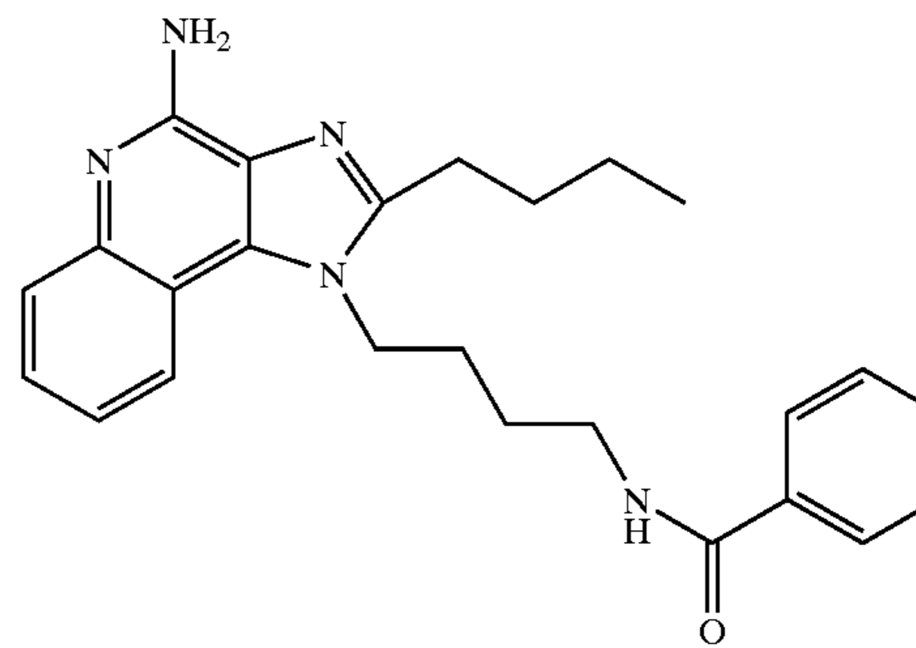
N 1 -[4-(4-Amino-2-butyl-1H-imidazo[4,5-c]quinolin-1-yl)butyl]benzamide
