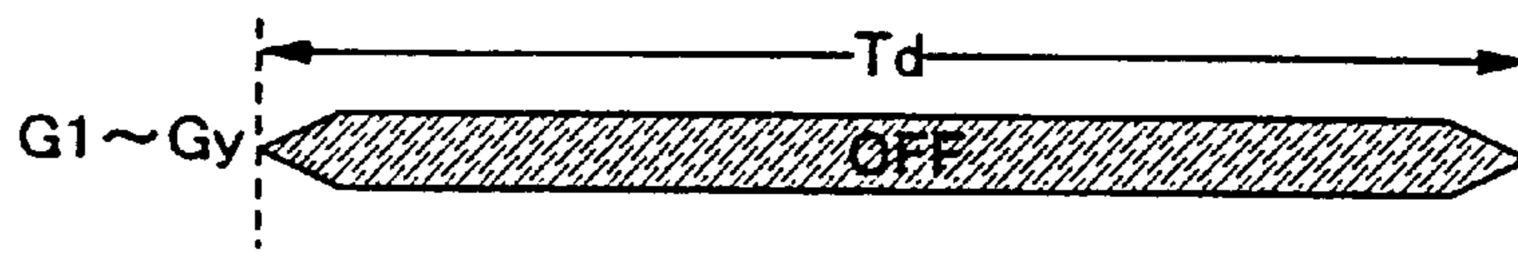
FIG. 3B DISPLAY PERIOD T_d
