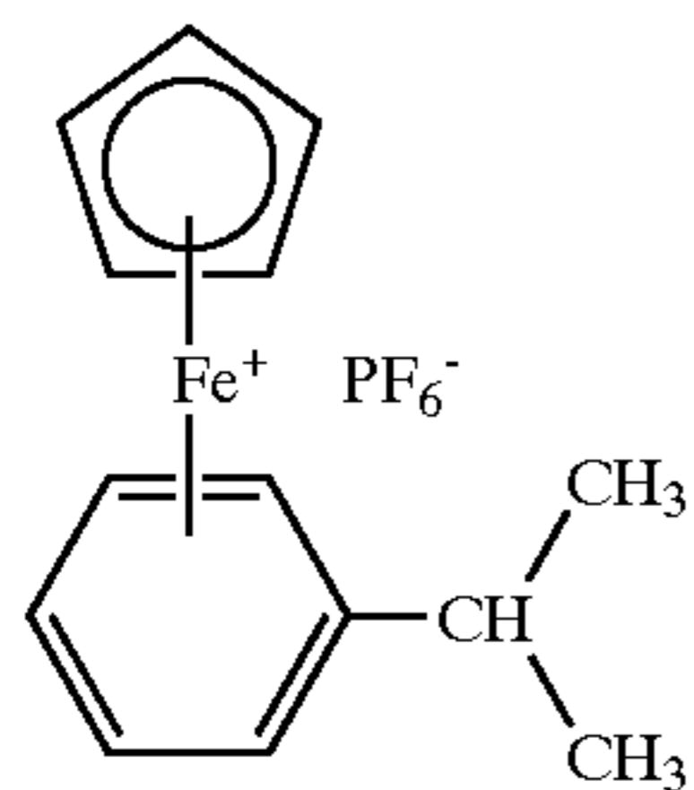
Irugacure 261
