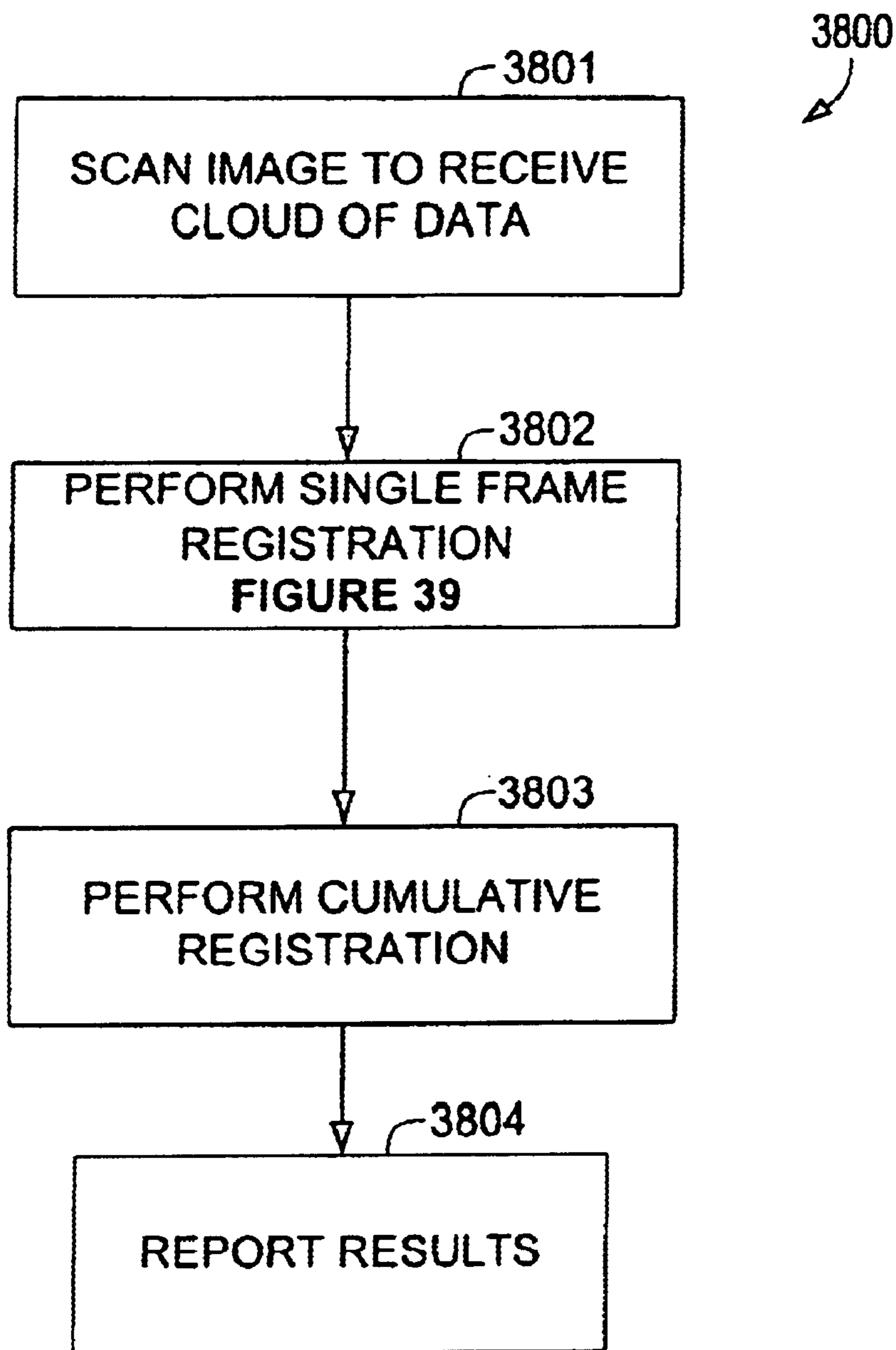
FIG. 38
