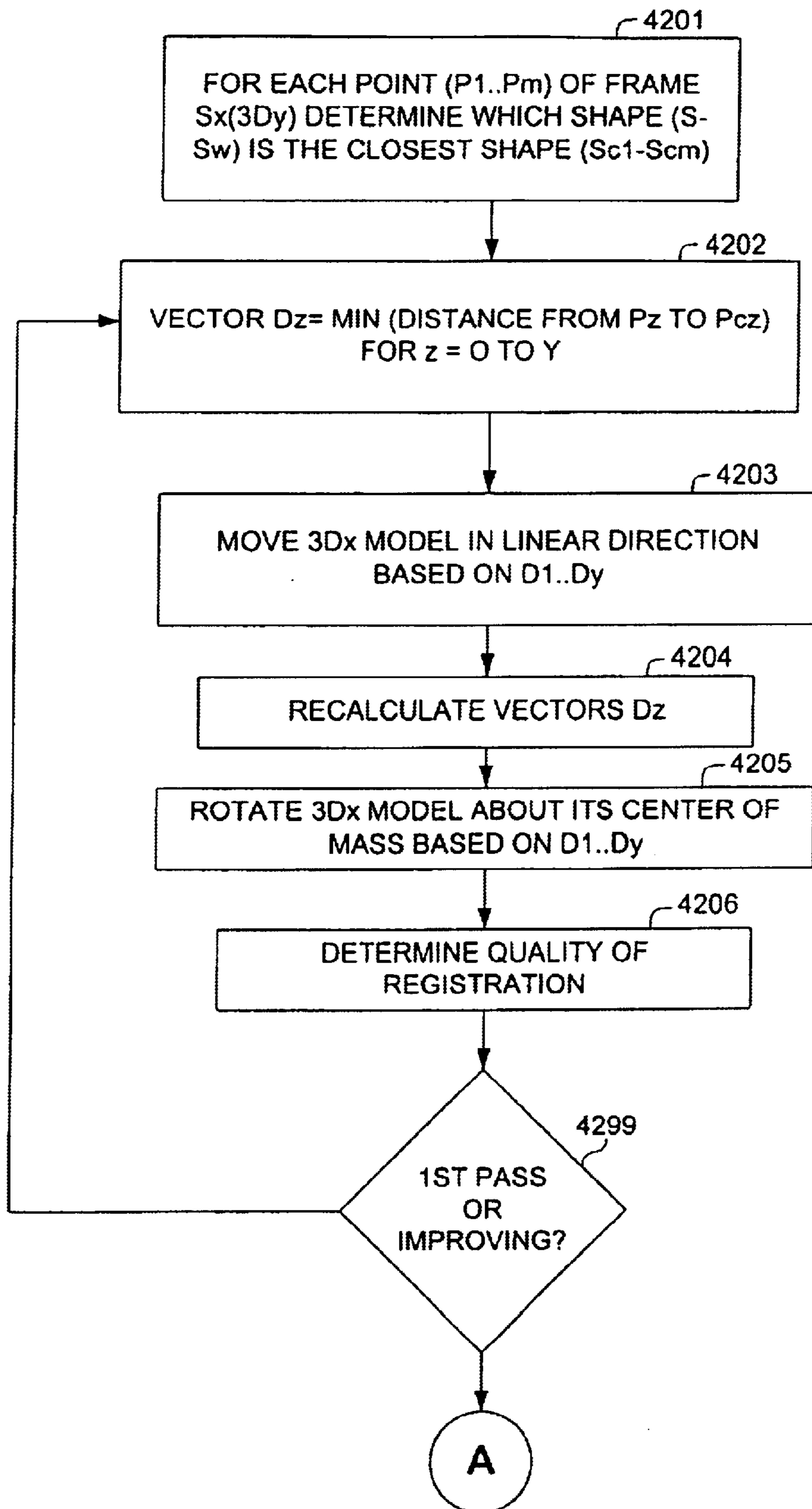
FIG. 42
