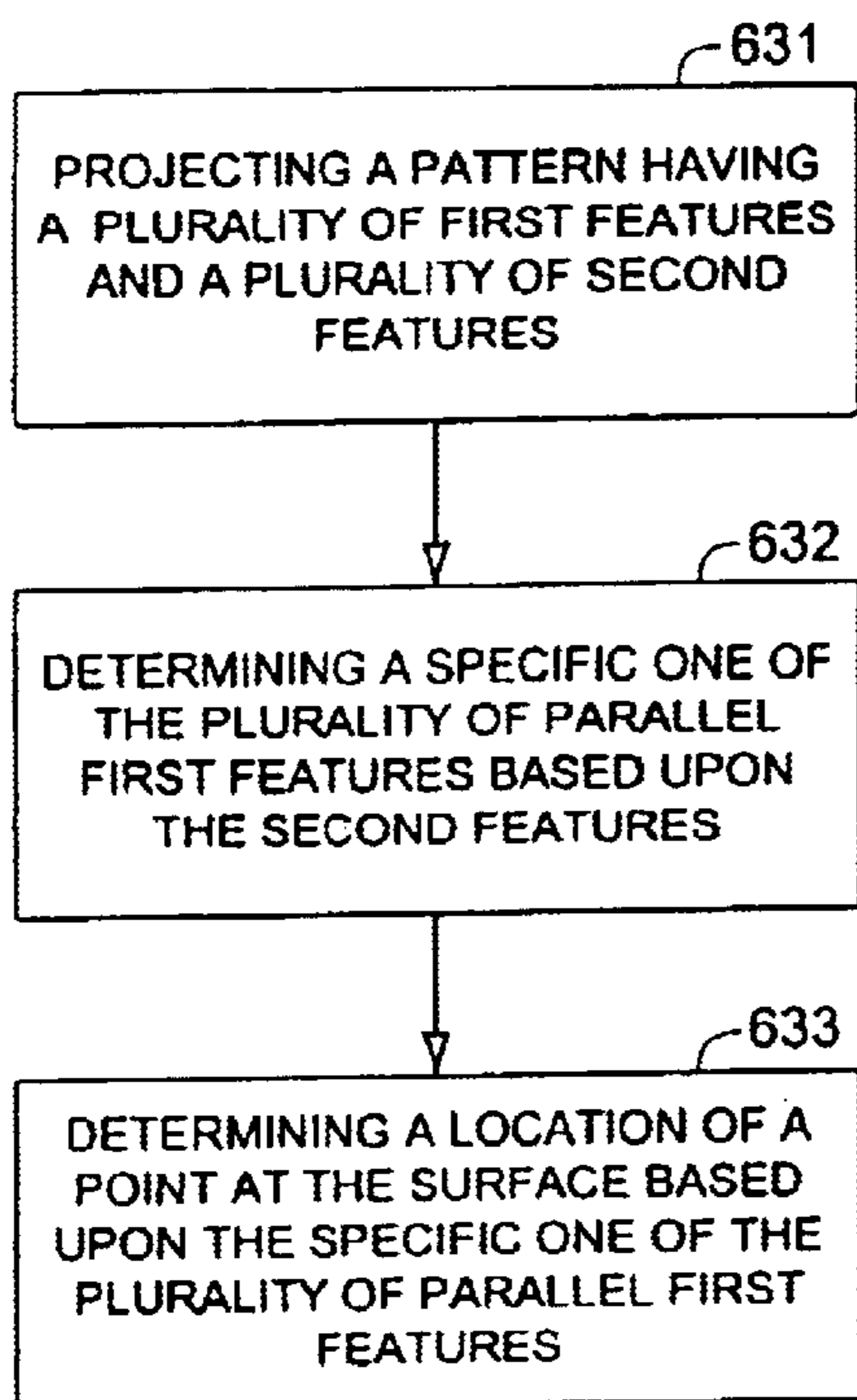
FIG. 21
