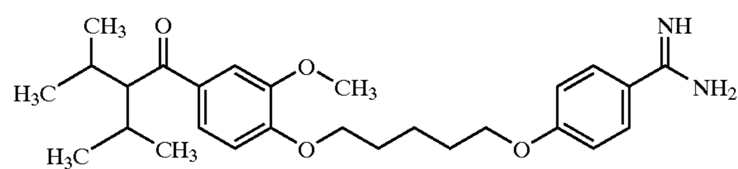
CGS-25019c
