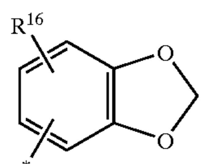
1,3-benzodioxolyl
