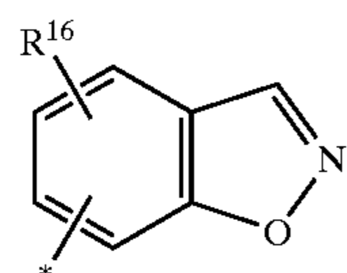
1,2-benzisoxazolyl
