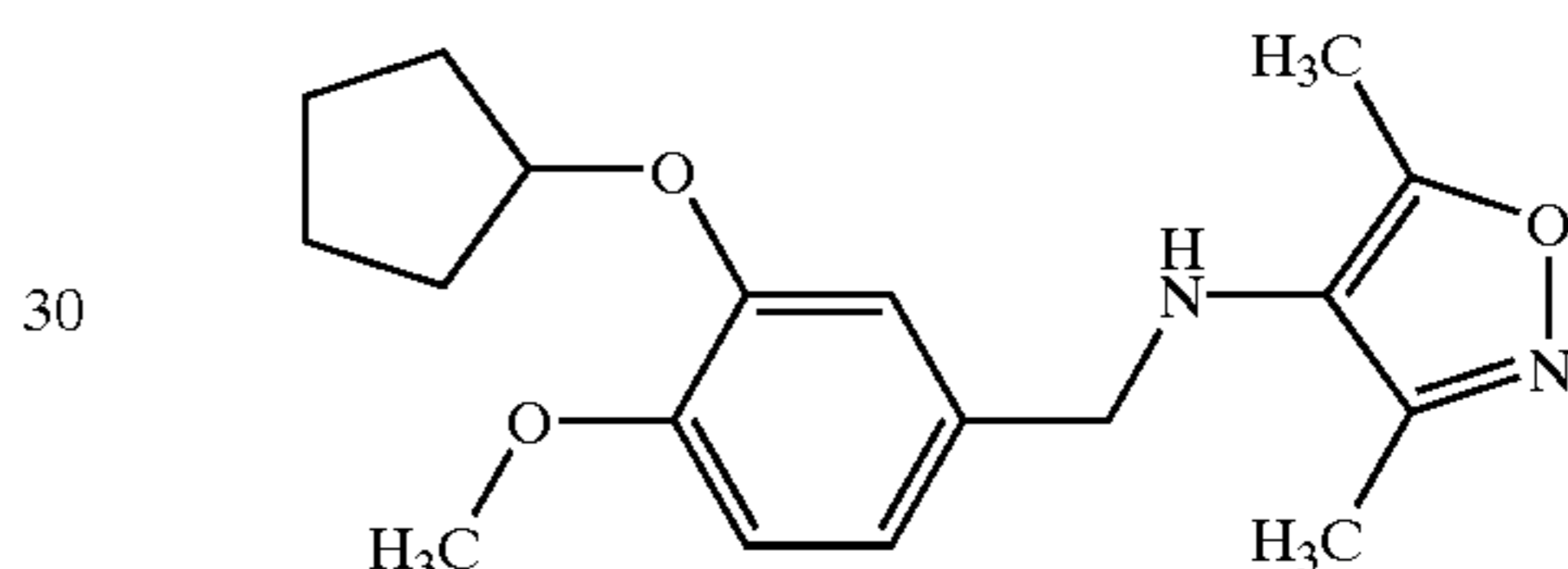
RPR-132294
