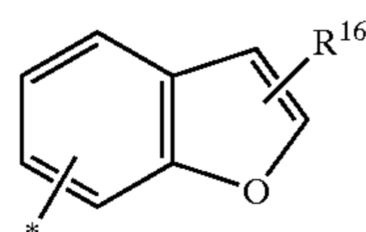
2,3-benzofuranyl
