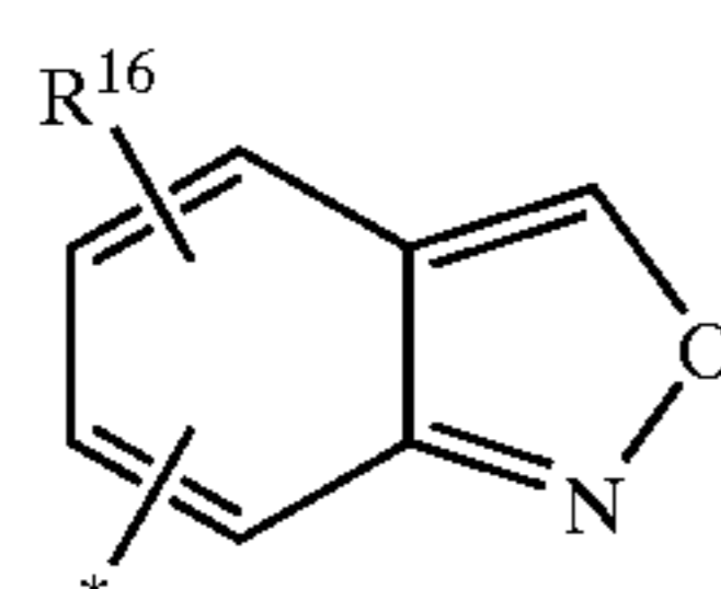
2,1-benzisoxazolyl
