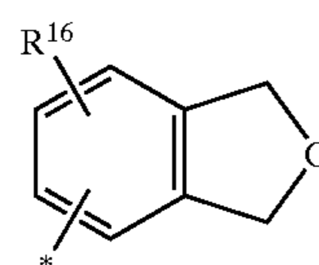
1,3-dihydroiso-benzofuranyl
