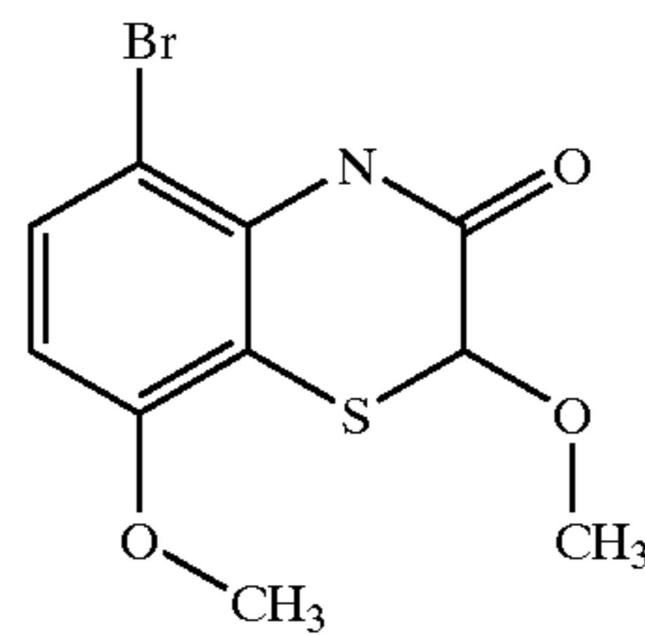
L-651,392
