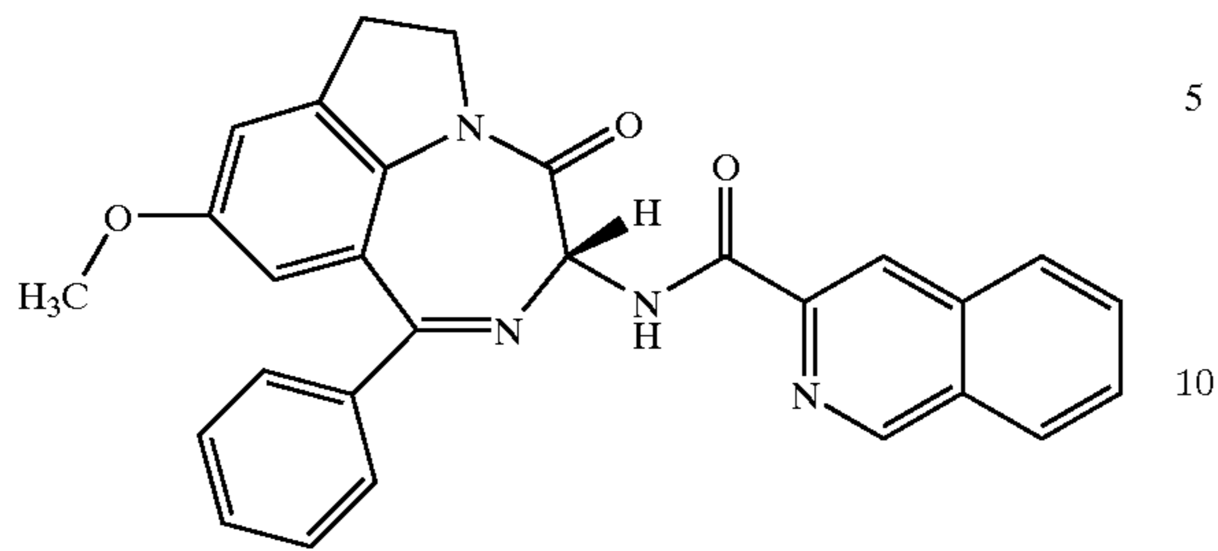
Cl-1018
