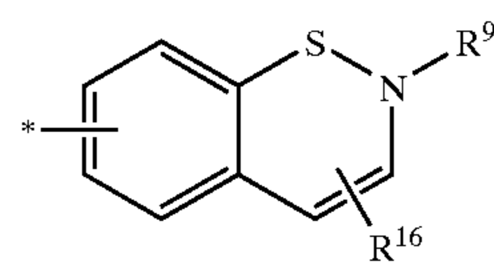
1,2-benzothiazinyl
