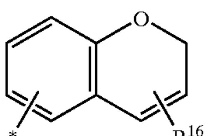
1H-2-benzopyranlyl
