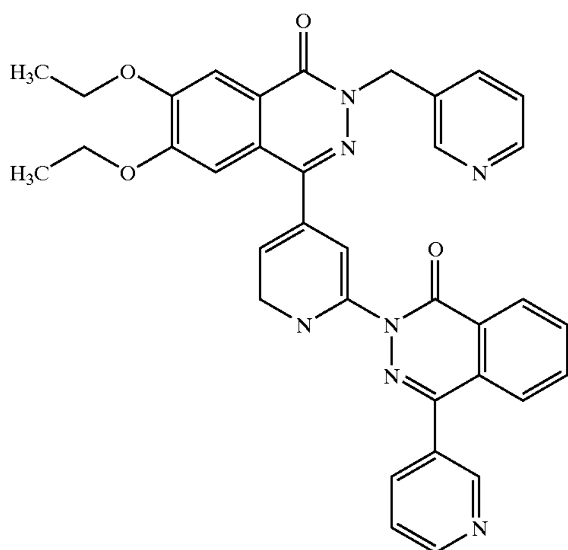
T-2585
