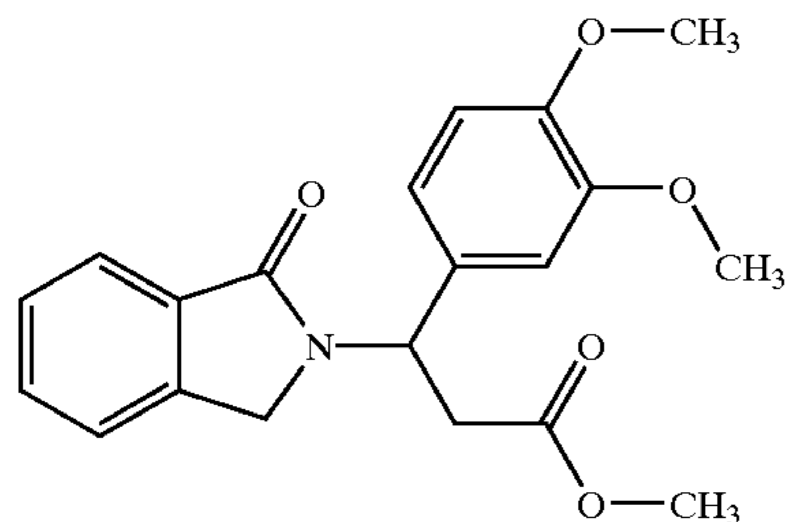
CDC-3052
