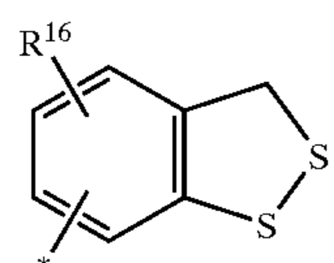
1,2-benzodithiolyl
