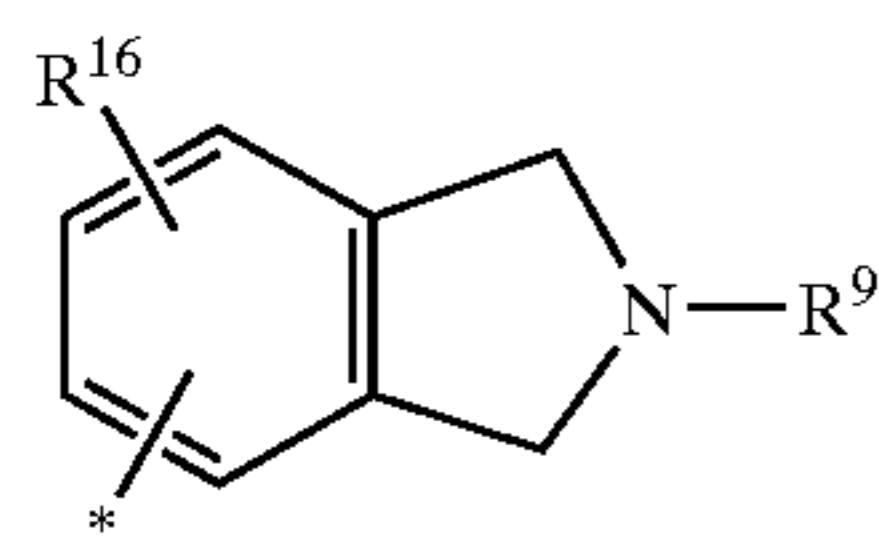
isoindolyl
