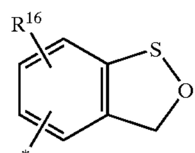
3H-2,1-benzoxathiolylyl
