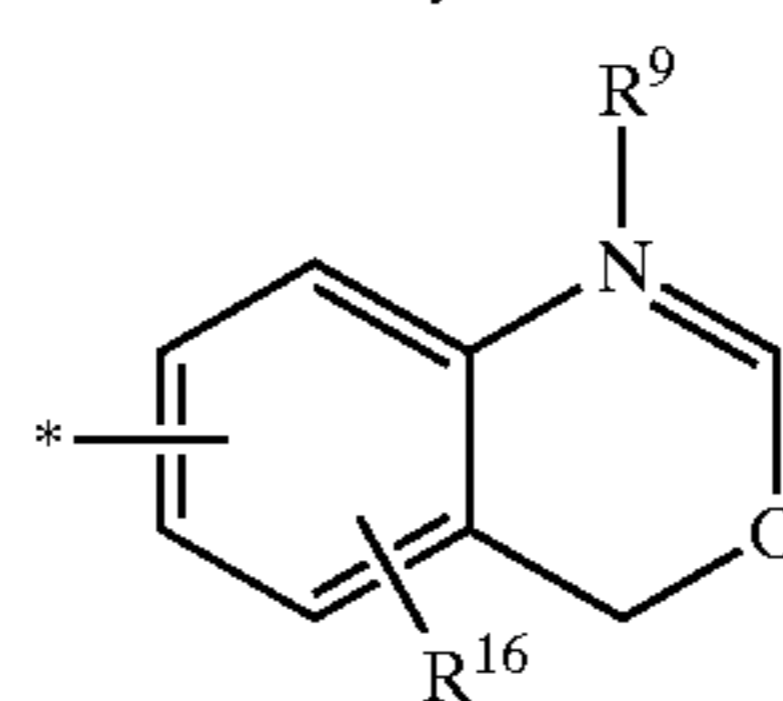
4H-3,1-benzoxazinyl
