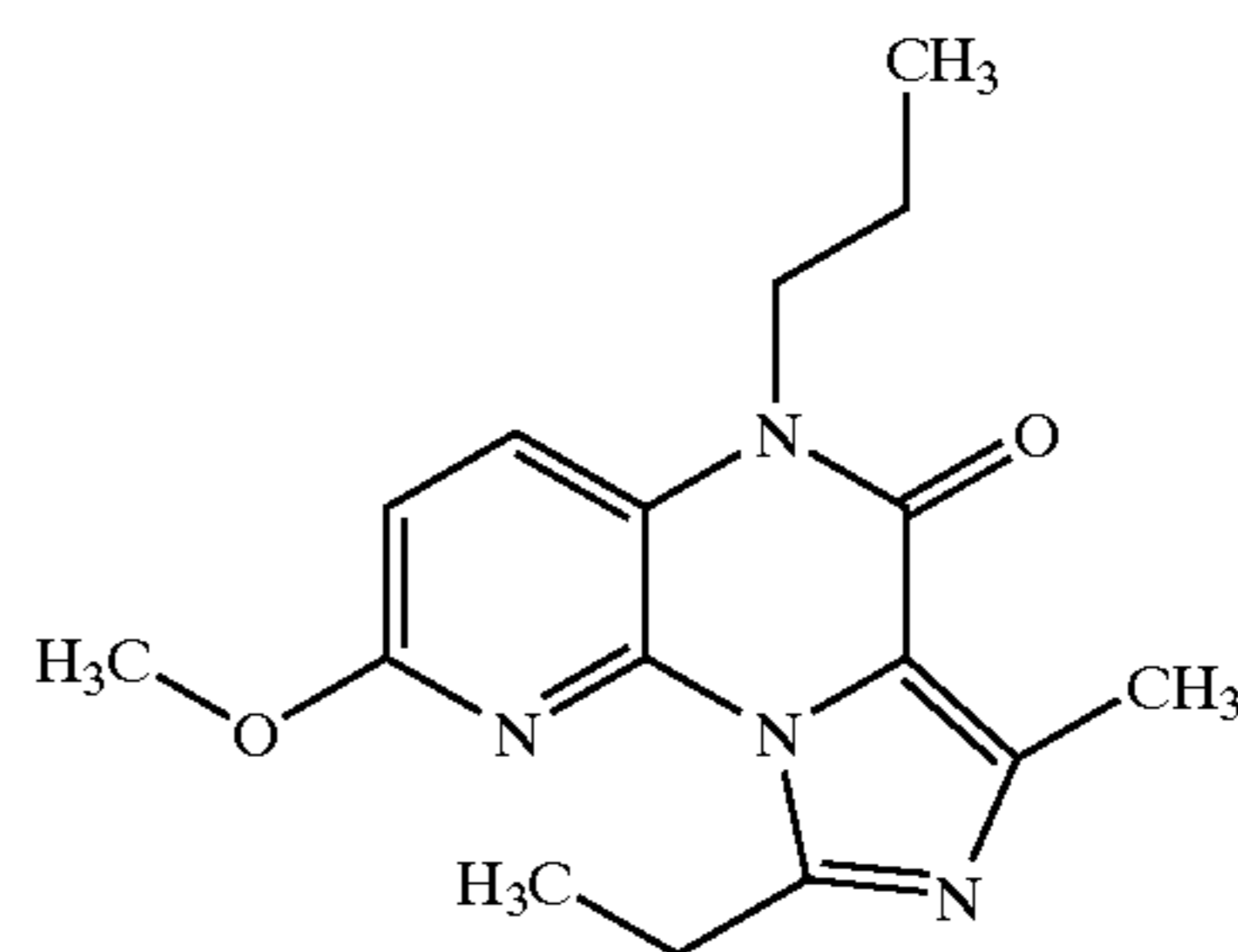
D-22888
