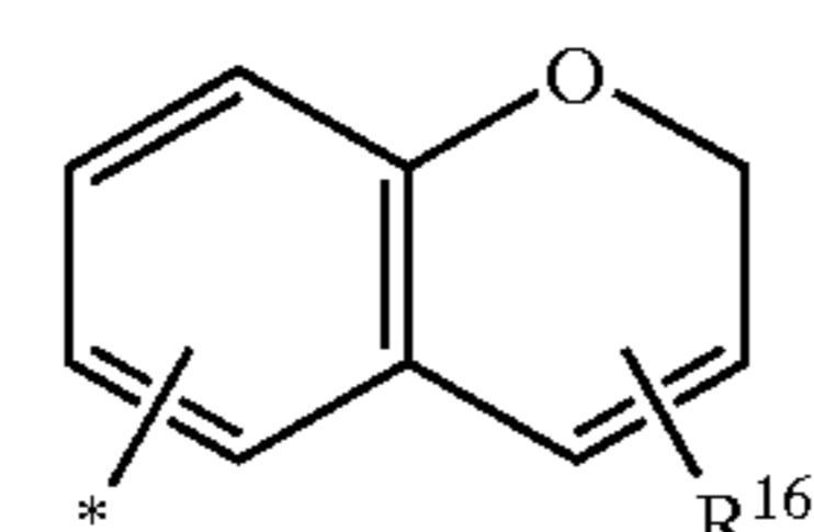
2H-1-benzopyranlyl
