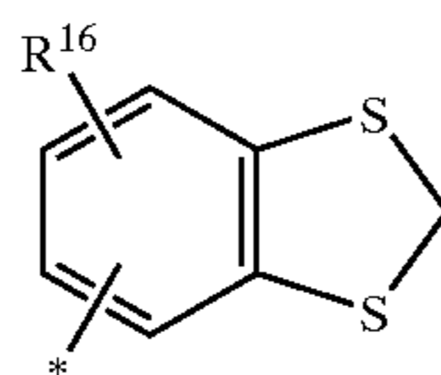
1,3-benzodithiolyl
