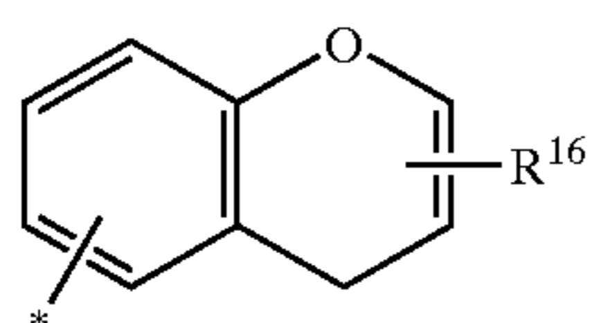
4H-1-benzopyranlyl
