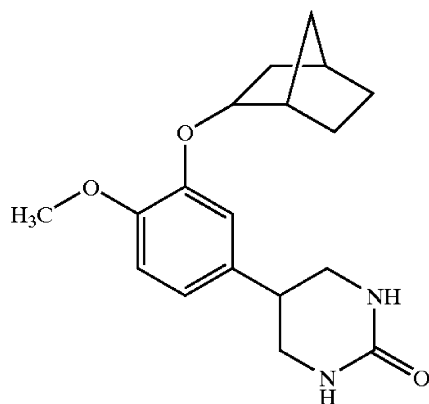
Atizoram (CP-80,633)
