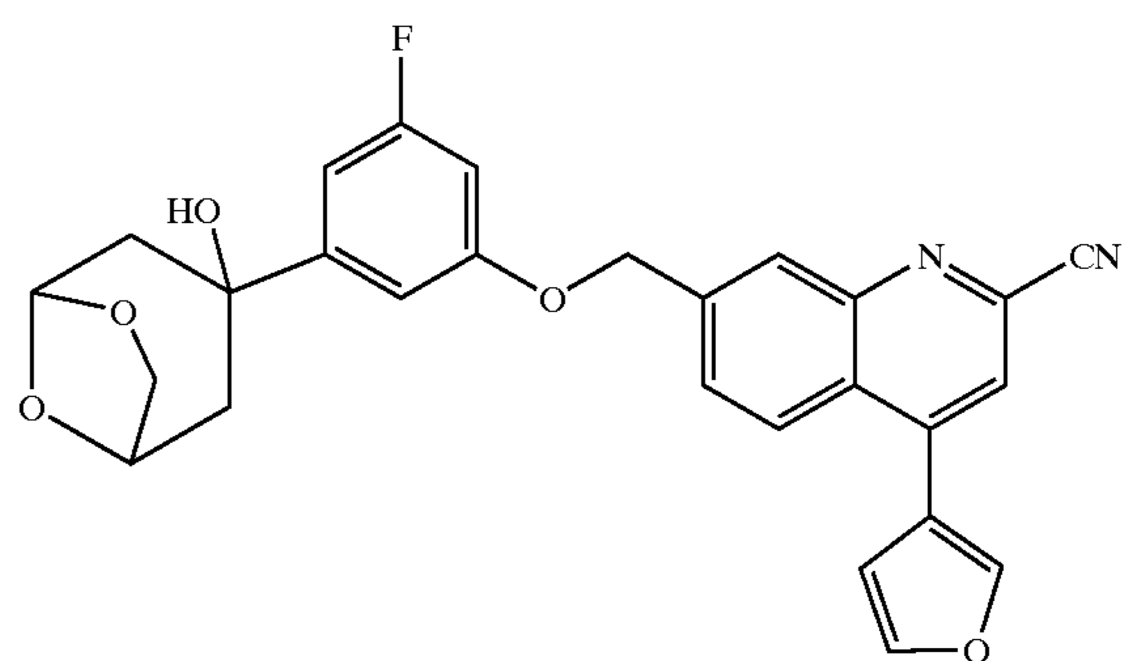
L-746,530
