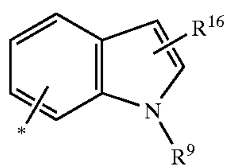
indolyl
