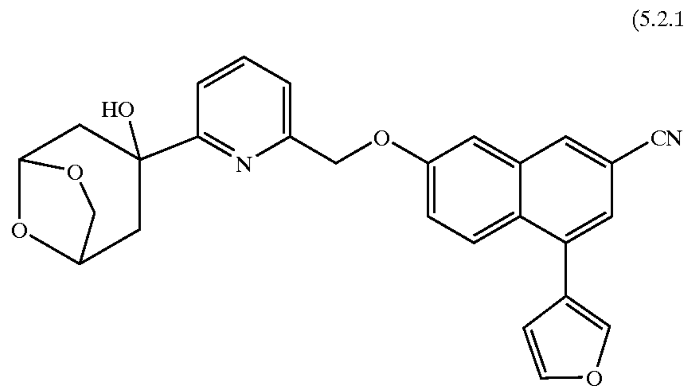
L-739,010
