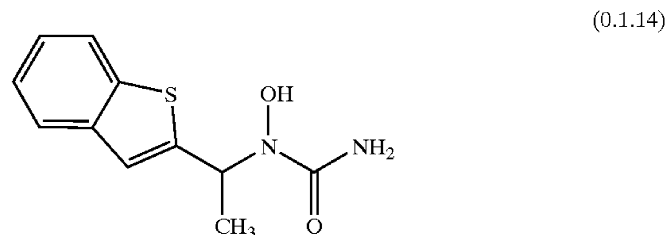
Zileuton
