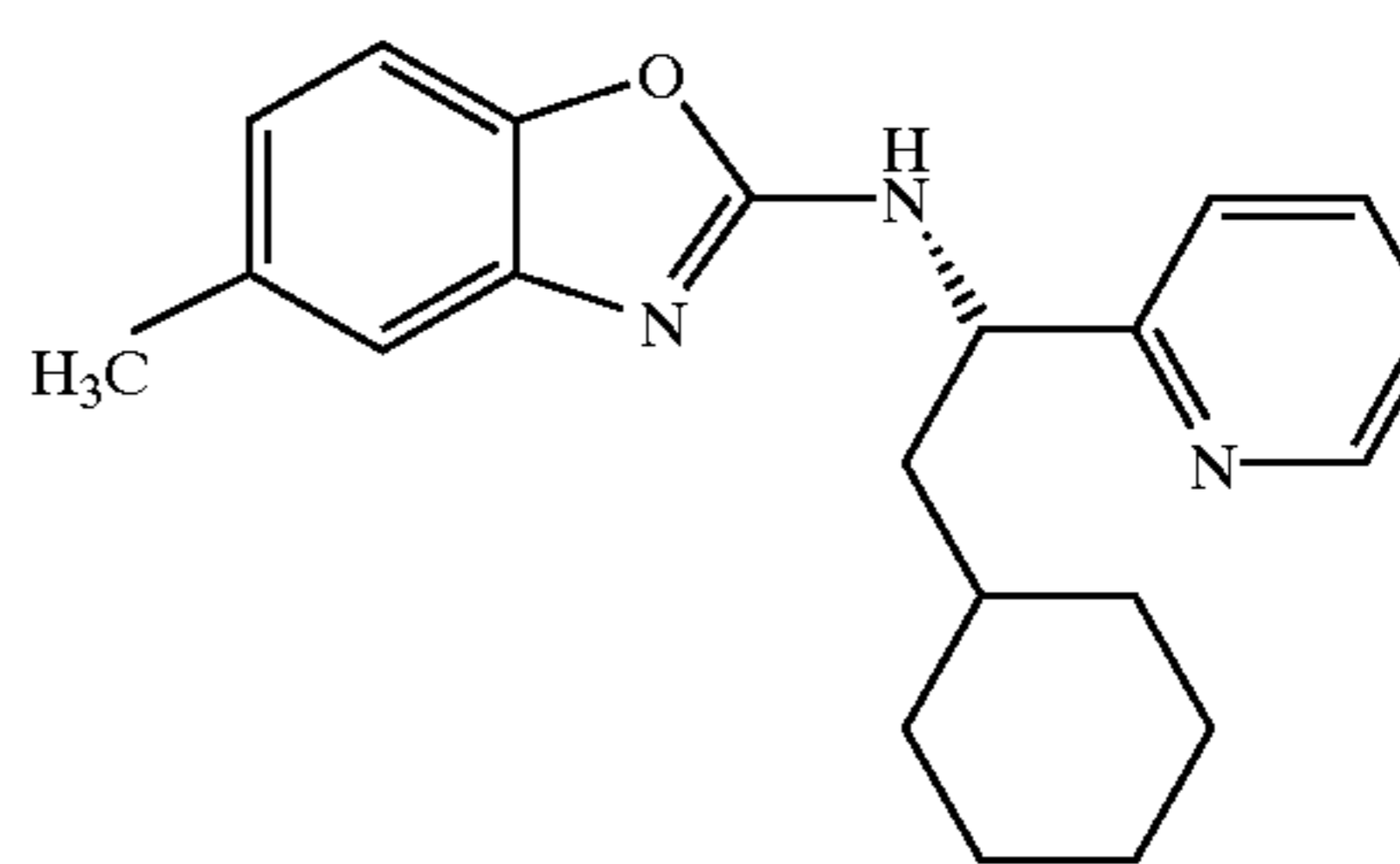
Ontazolast
