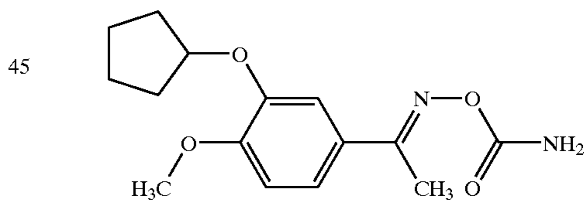
Flaminast (WAY-PDA-641)
