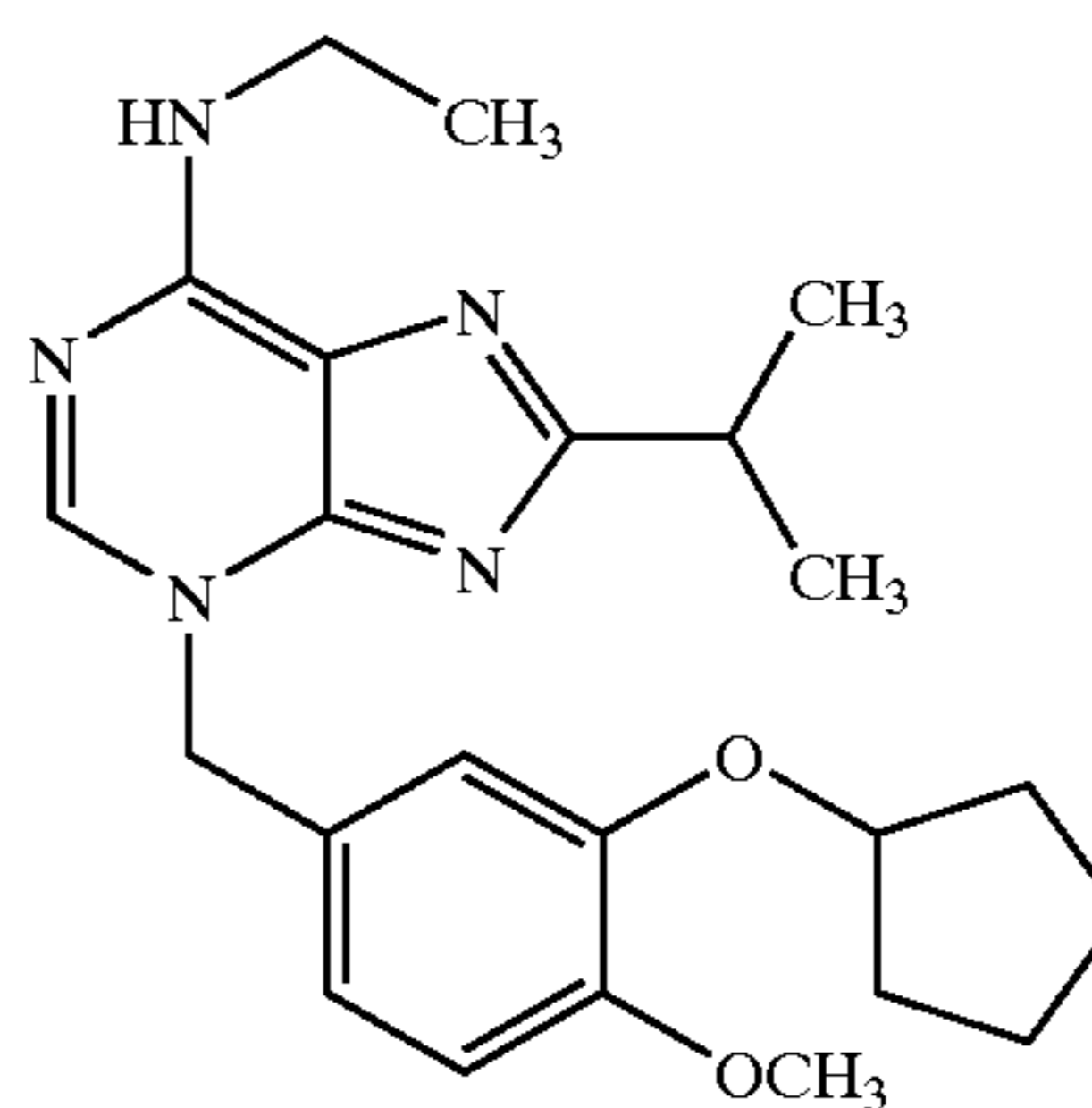
V-11294A
