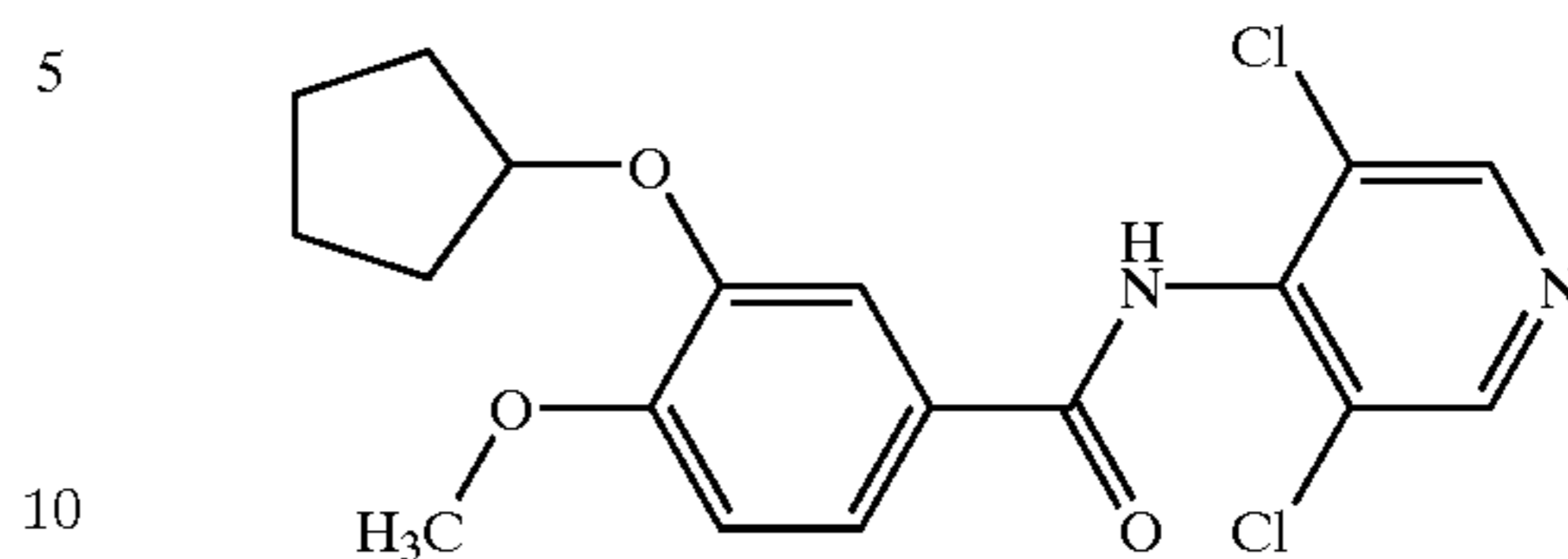
Piclamilast (RP-73,401)
