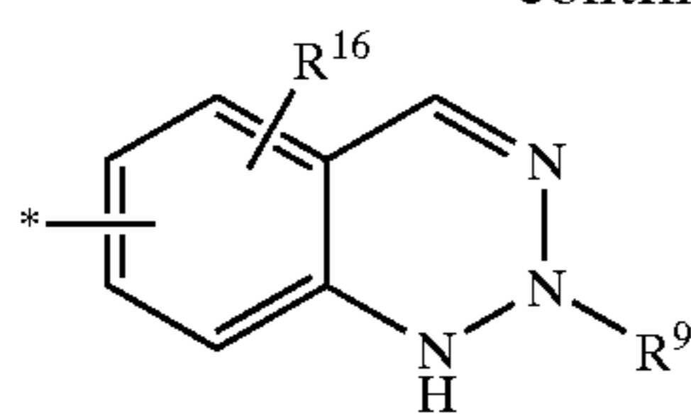
1,2,3-benzotriazinyl
