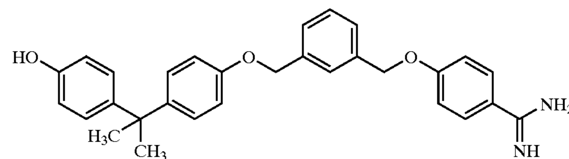
BIIL 284/260
