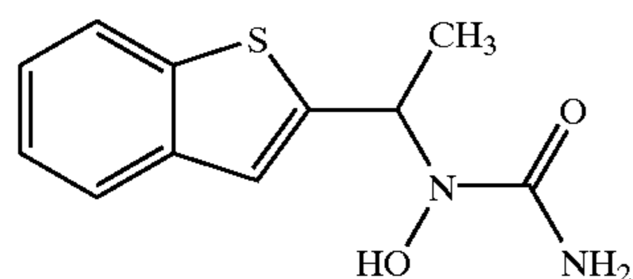
ZYFLO®
