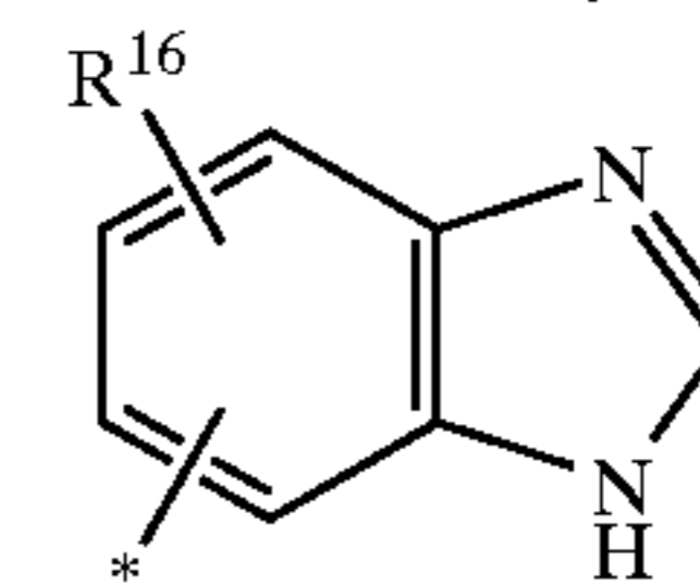
benzimidazolyl
