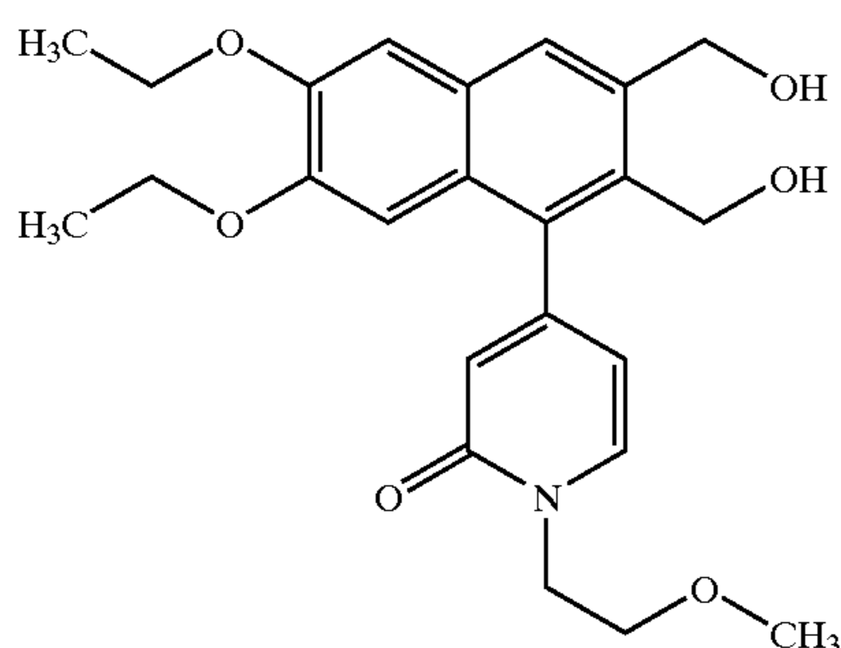
T-440
