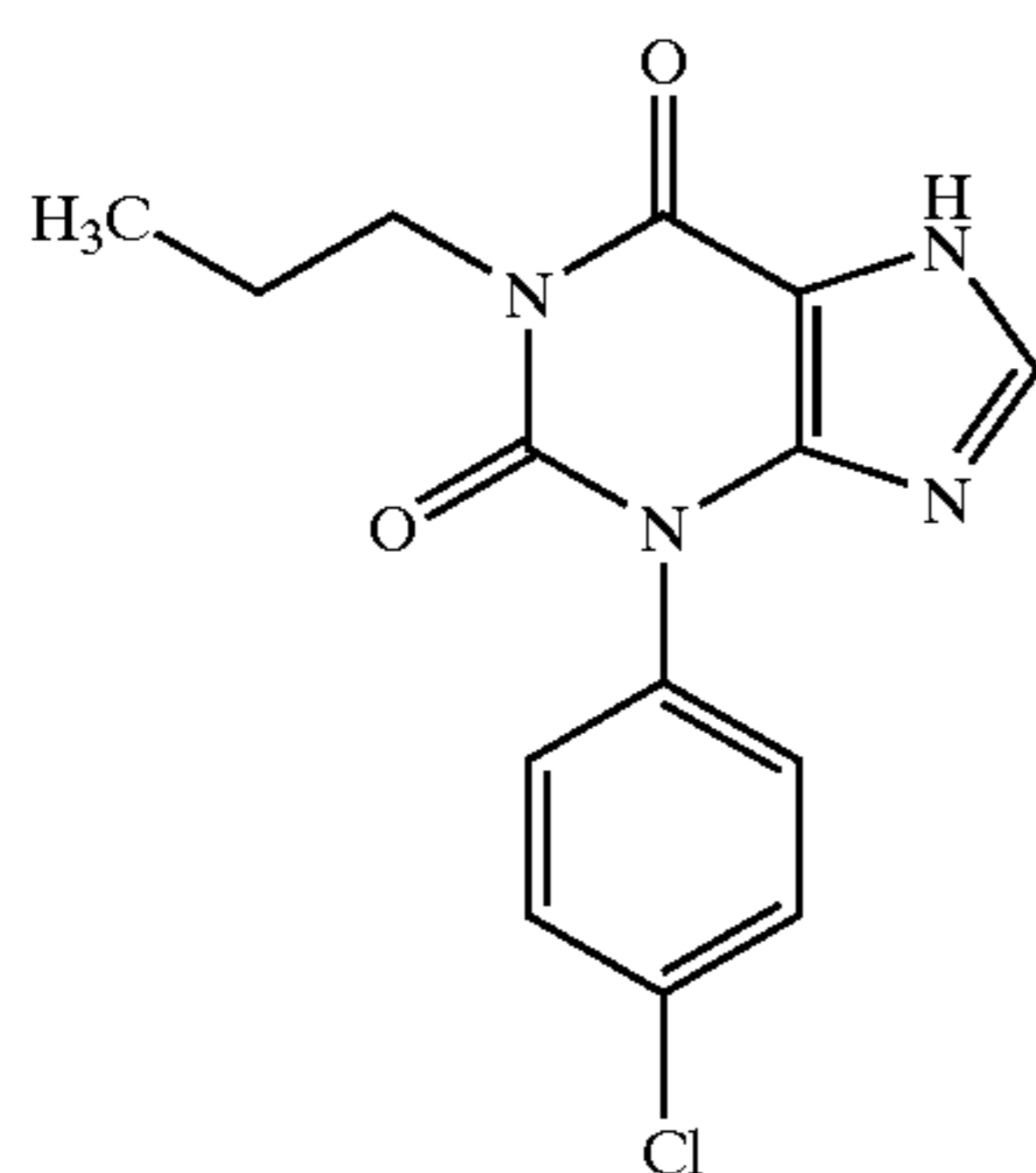
Arofylline (LAS-31025)
