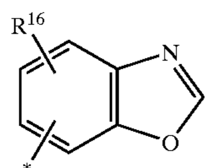
benzoxazolyl
