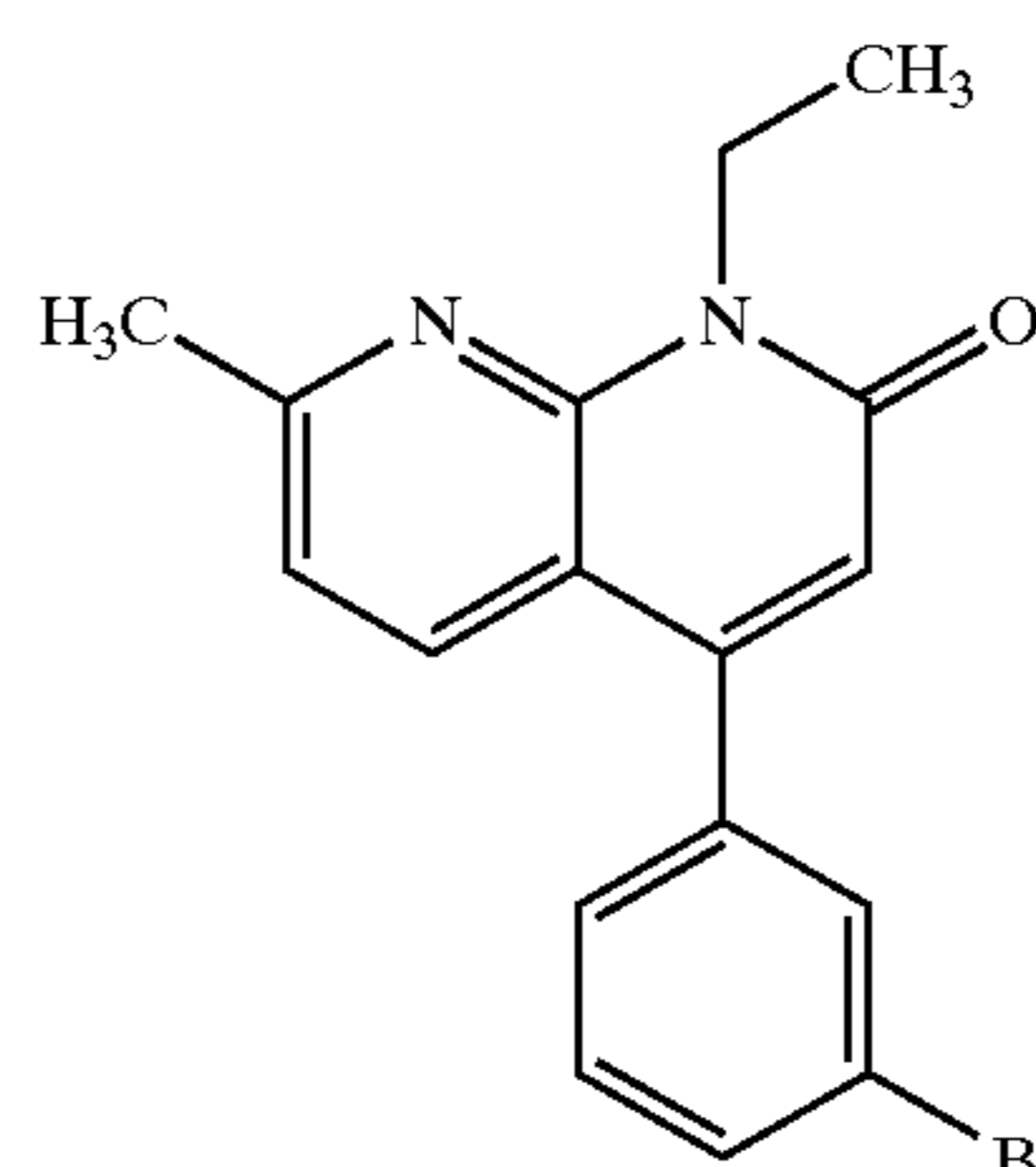
YM-58977
