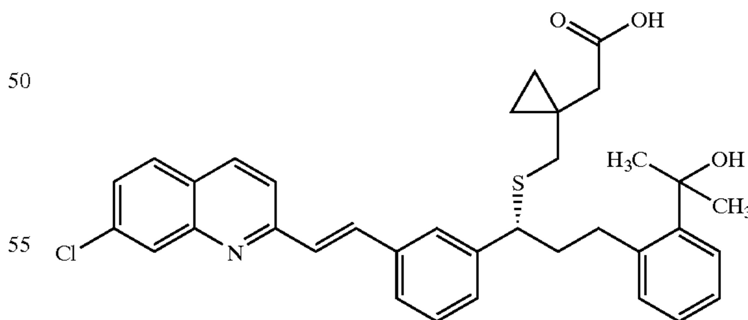
SINGULAIR® Montelukast
