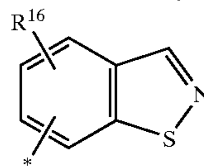
1,2-benzisothiazolyl
