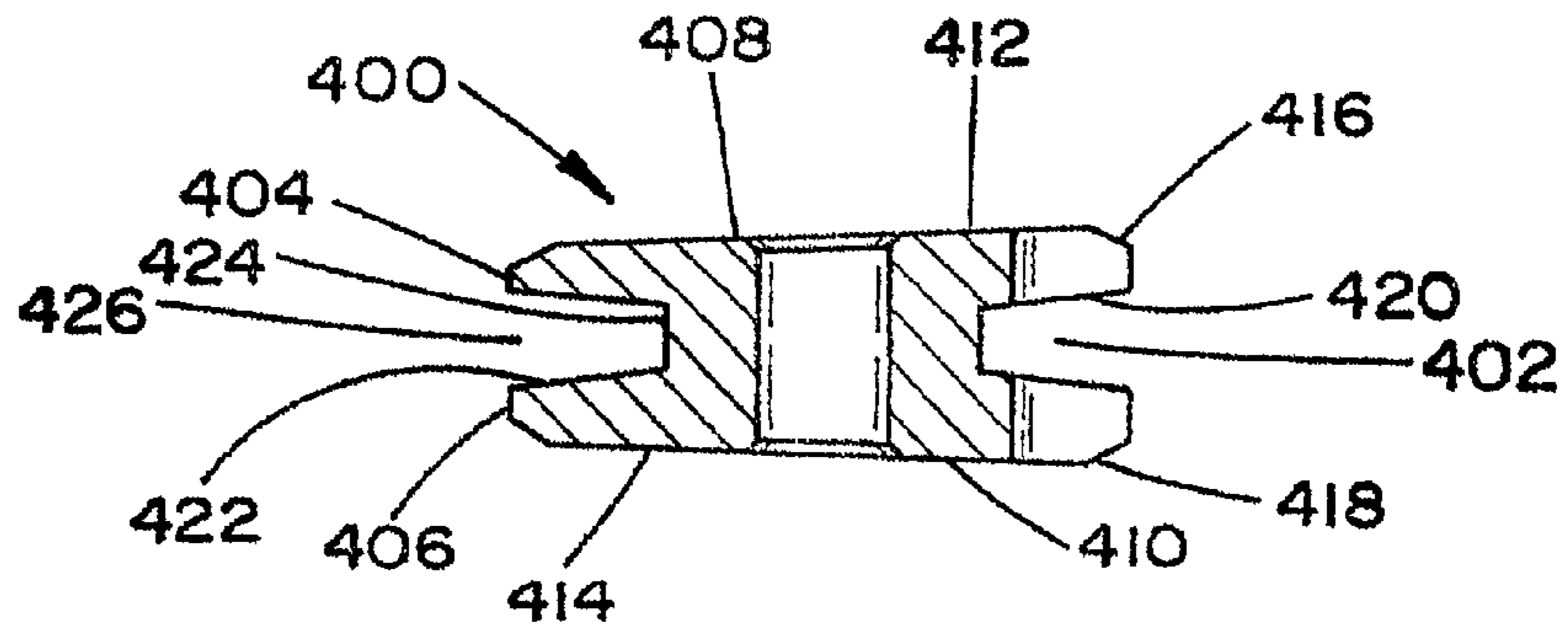
Section A-A FIG. 4c
