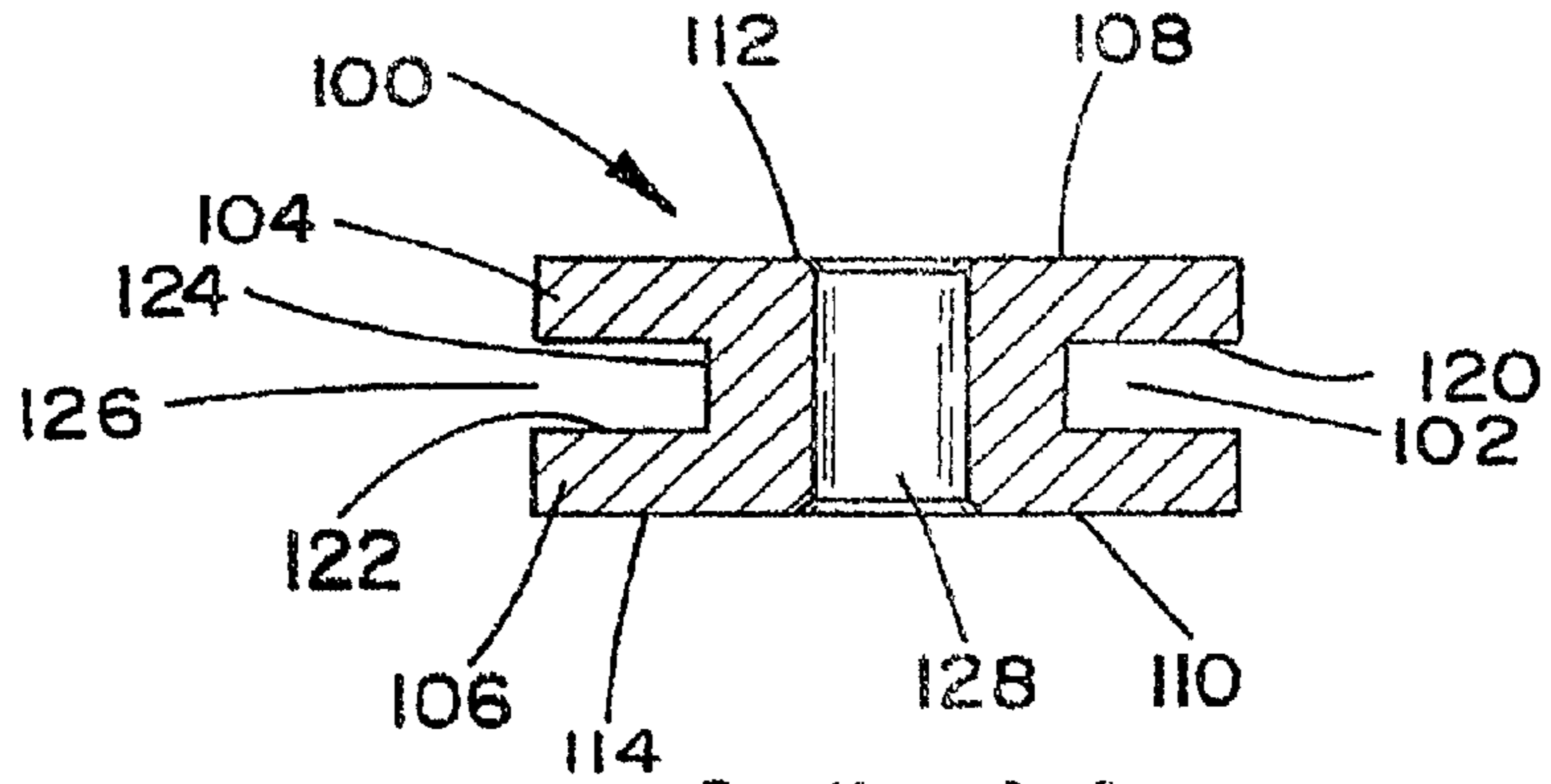
Section A-A
