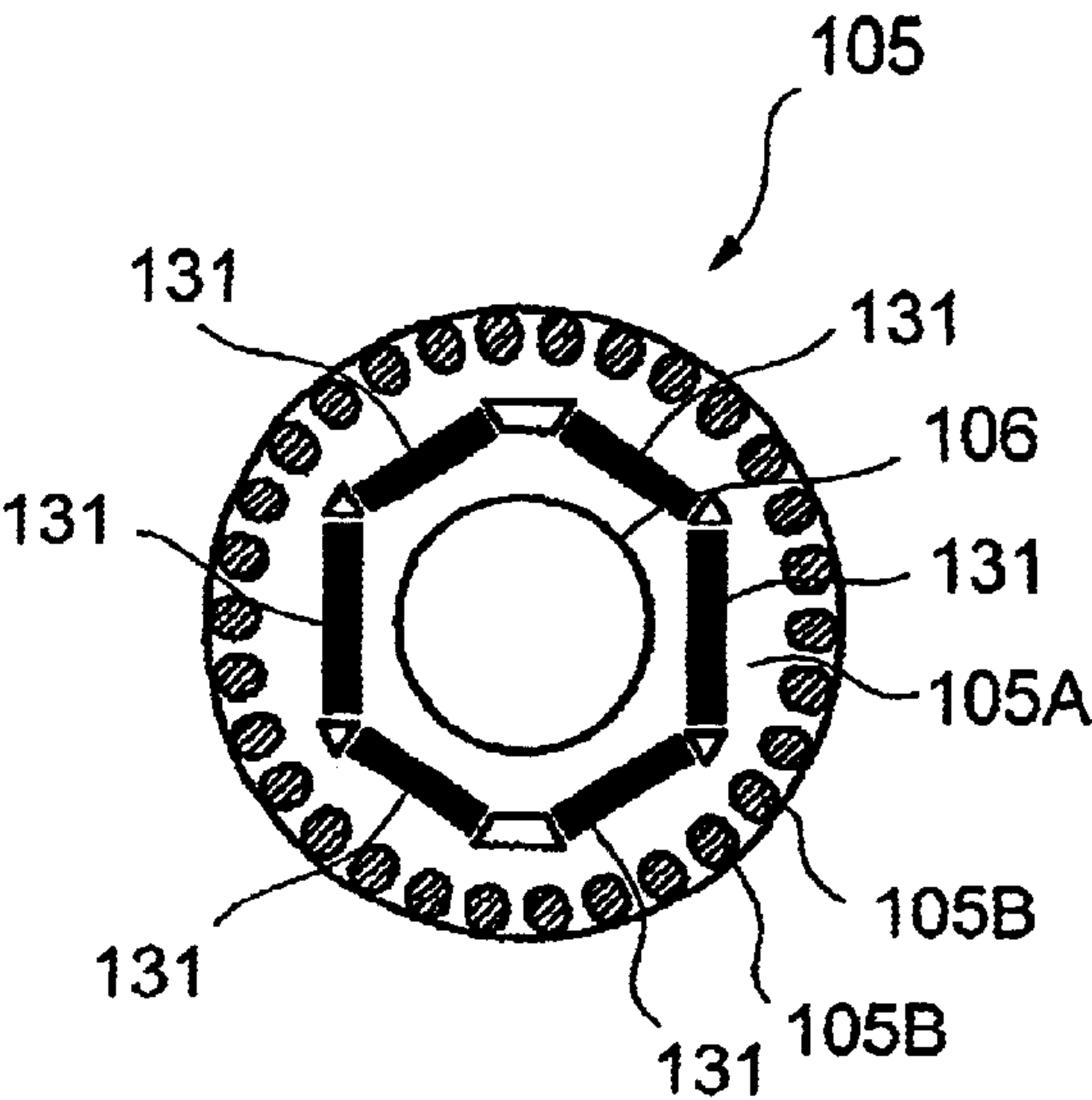
FIG.21
