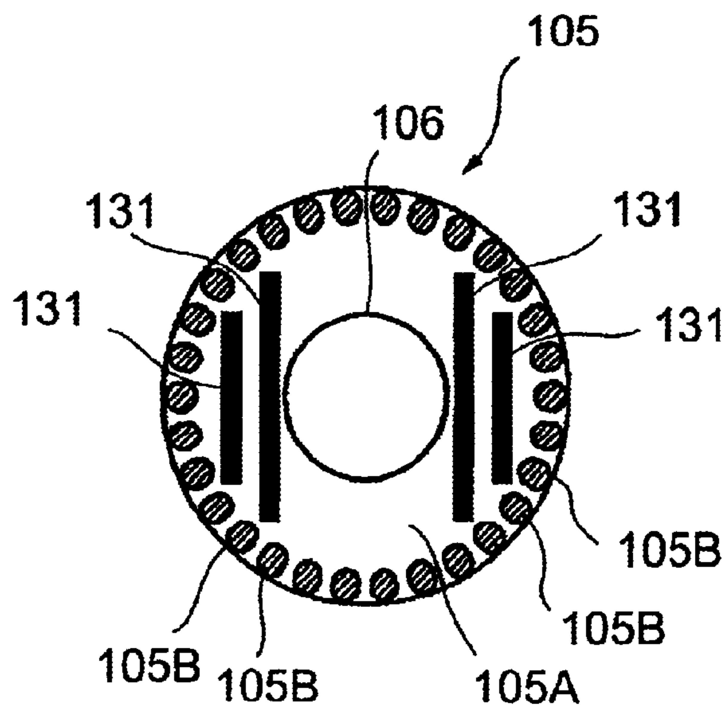
FIG.20
