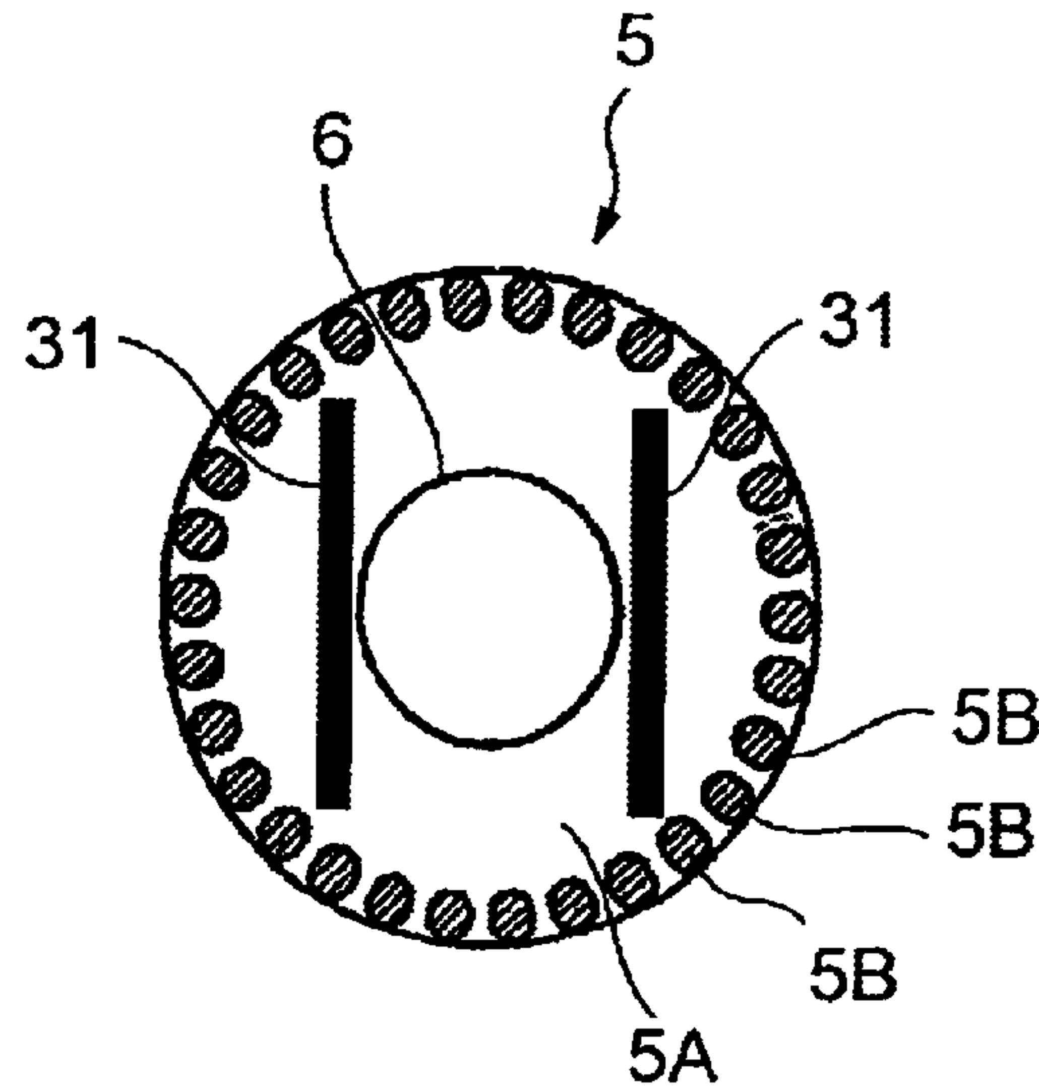
FIG.3
