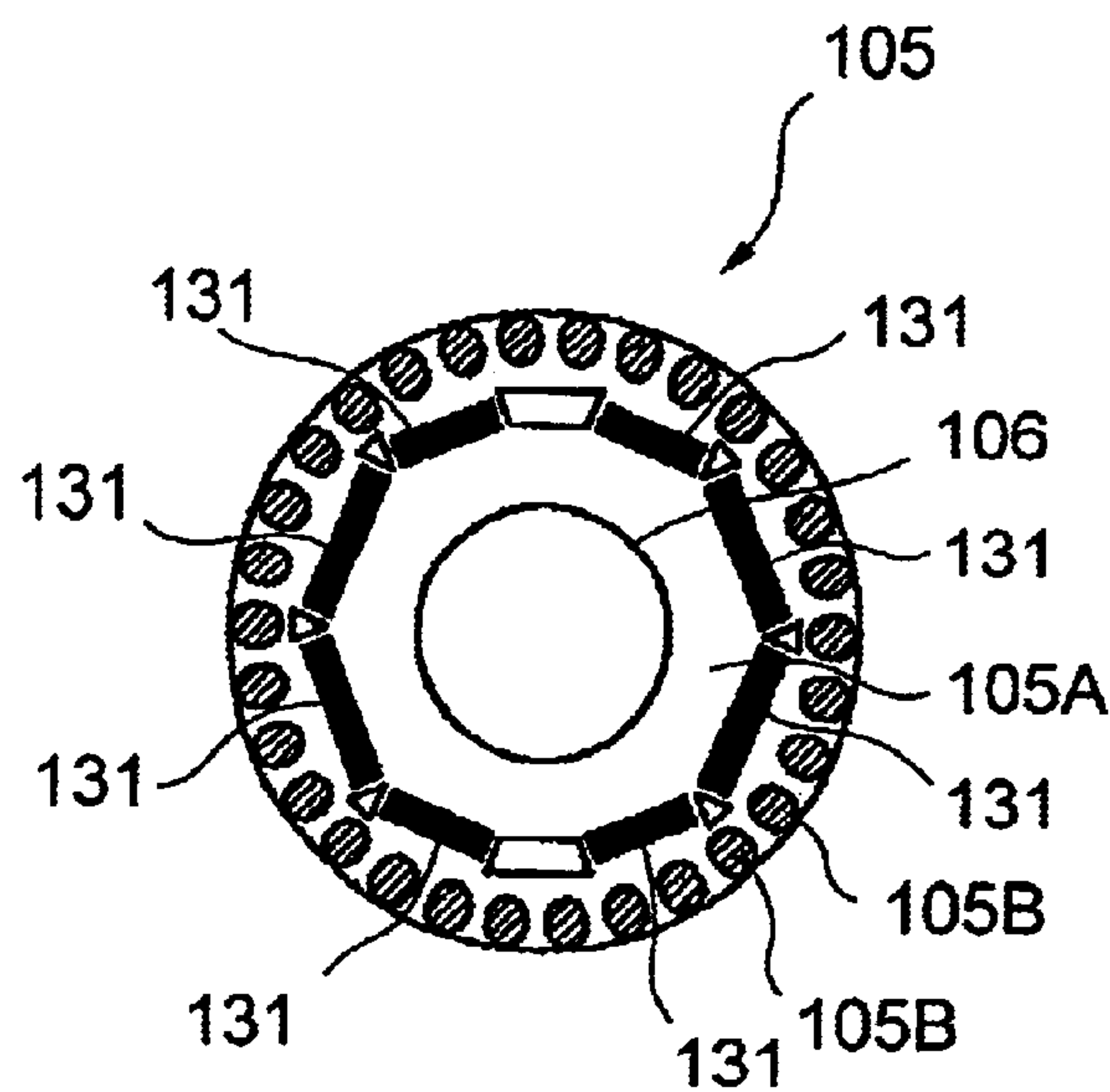
FIG.23
