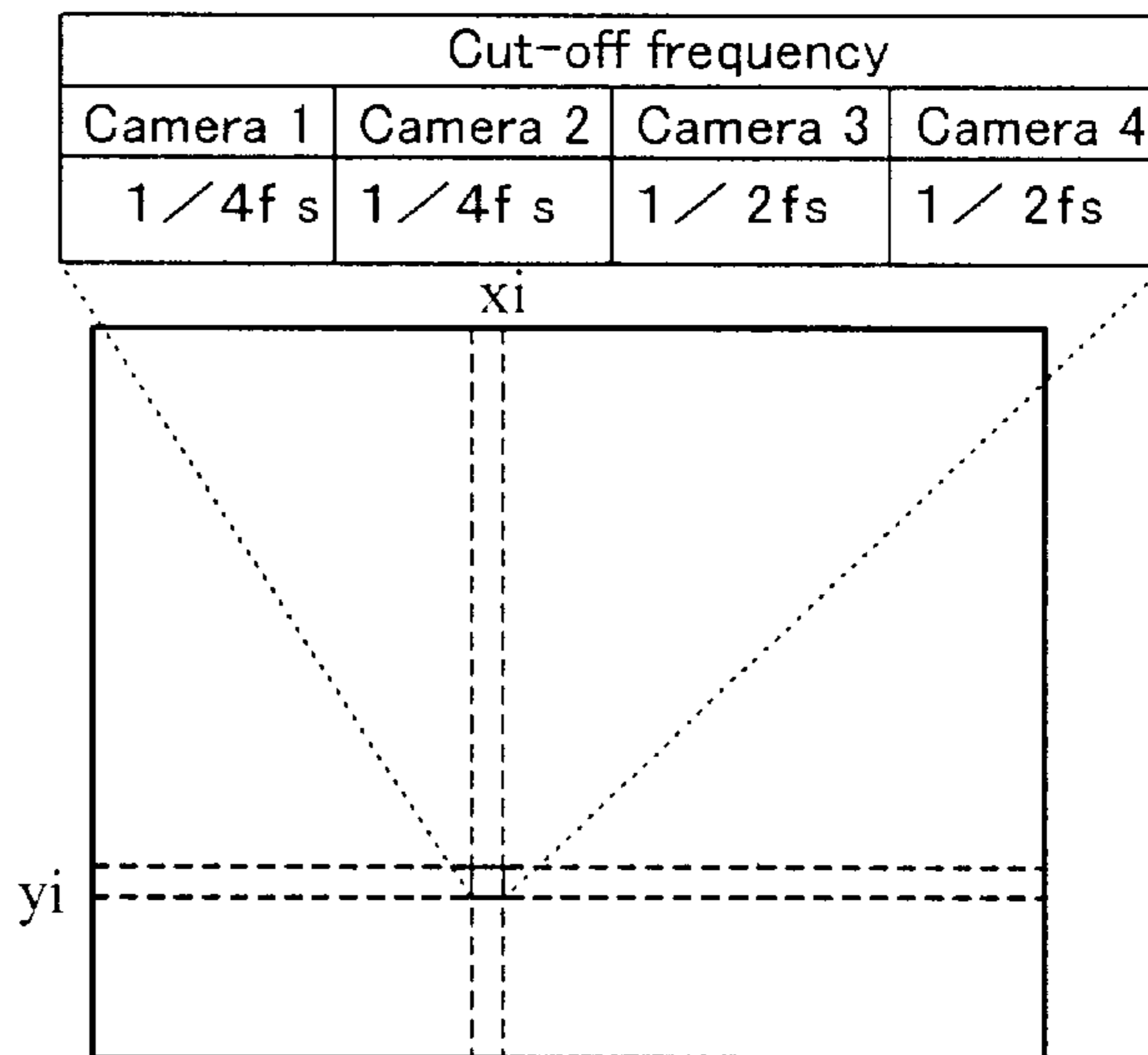
Filter parameter group
