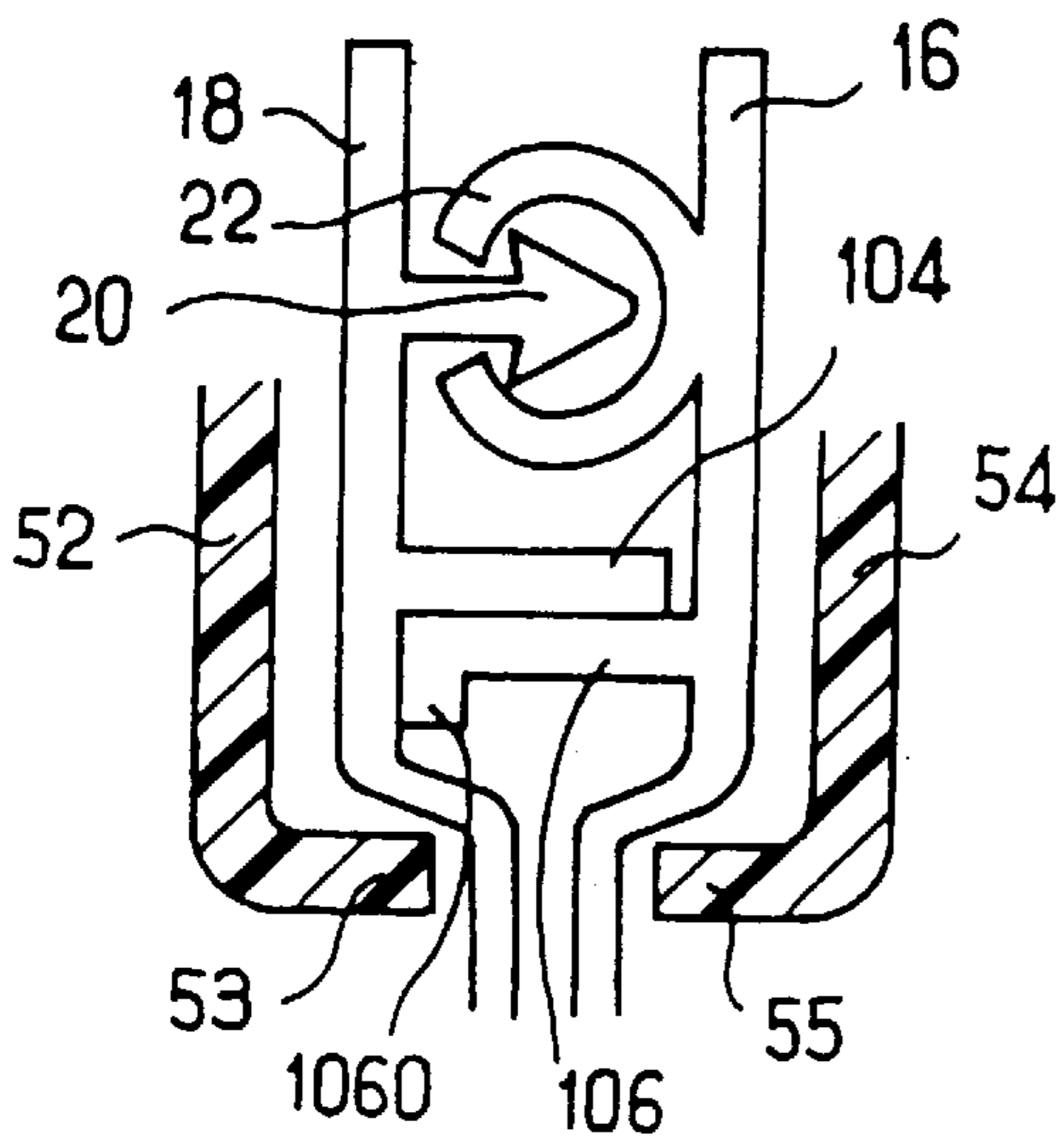
FIG. 16
