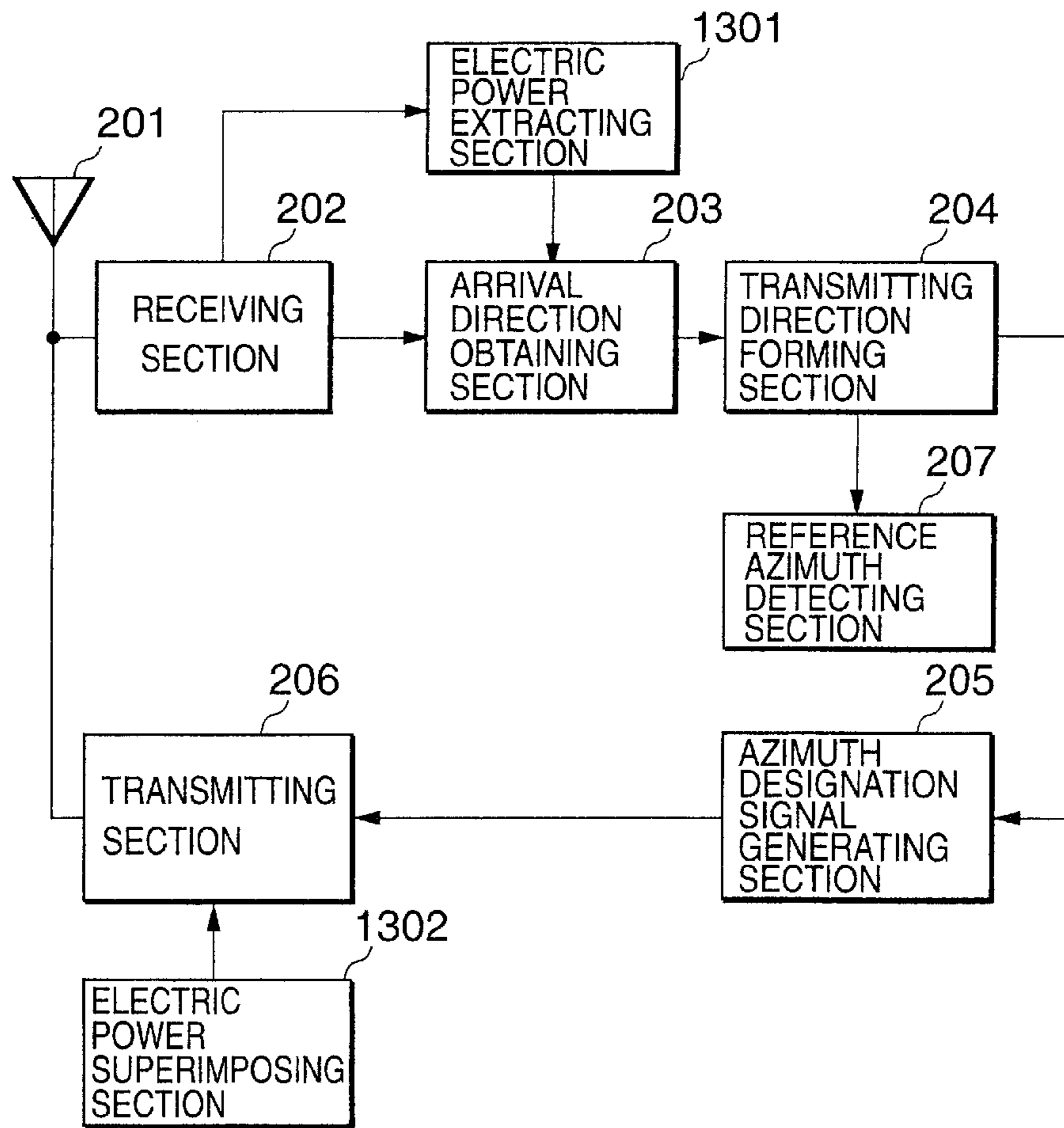
FIG. 13
