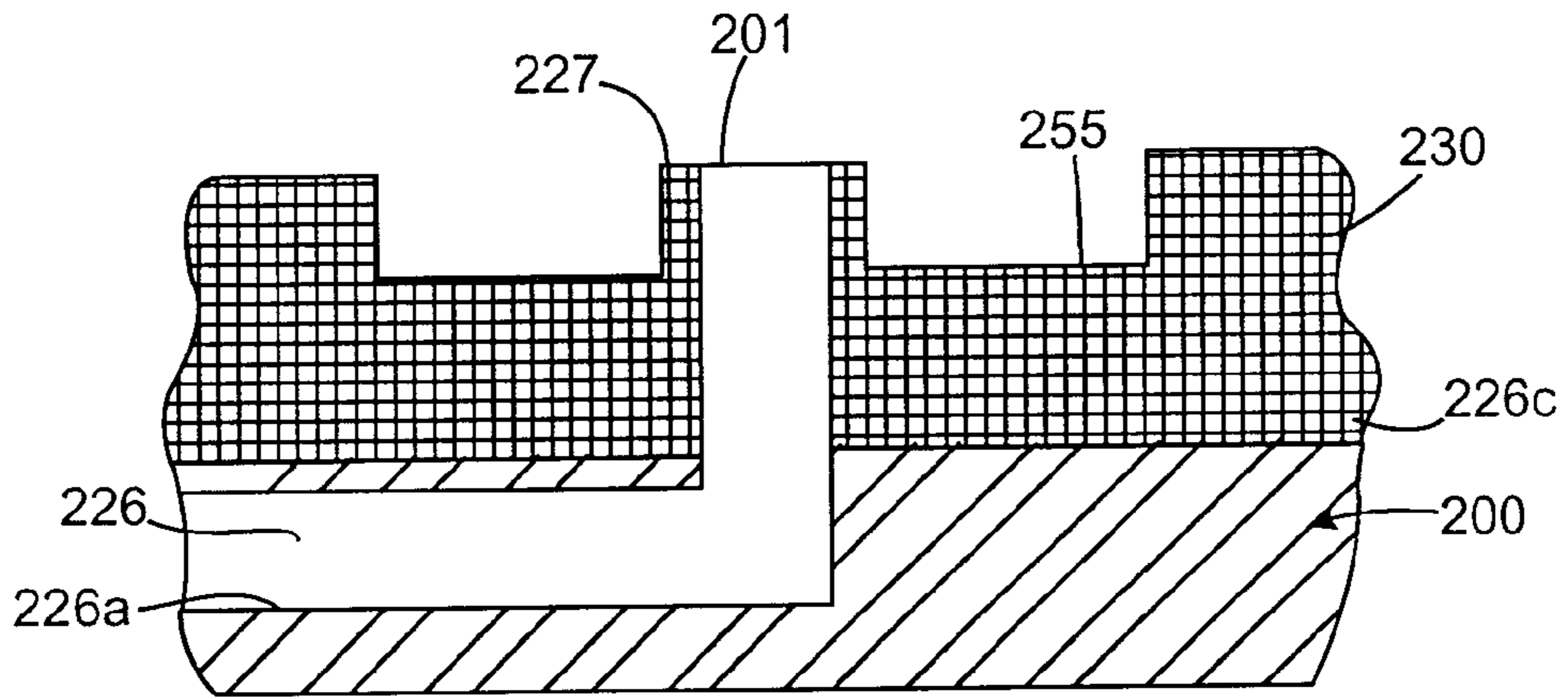
FIG. 31
