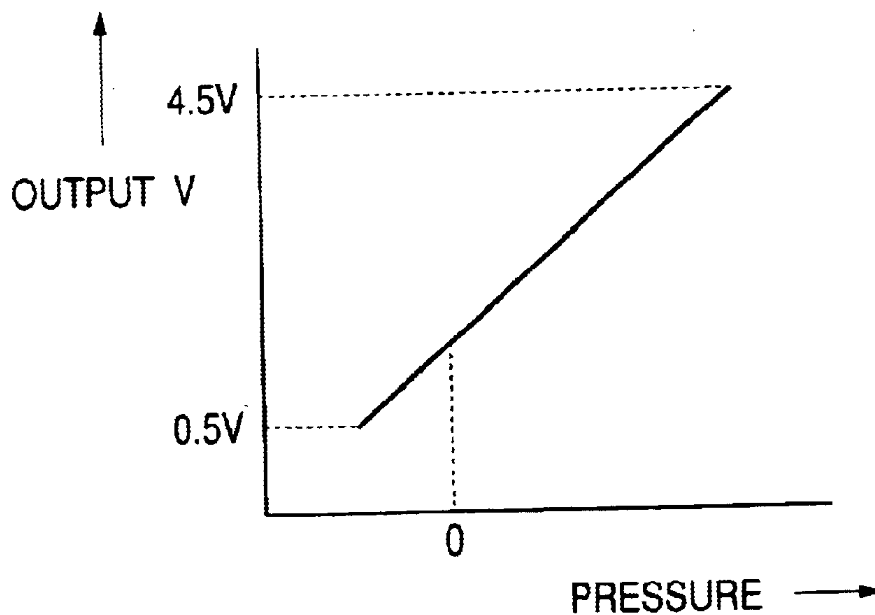
FIG. 12
