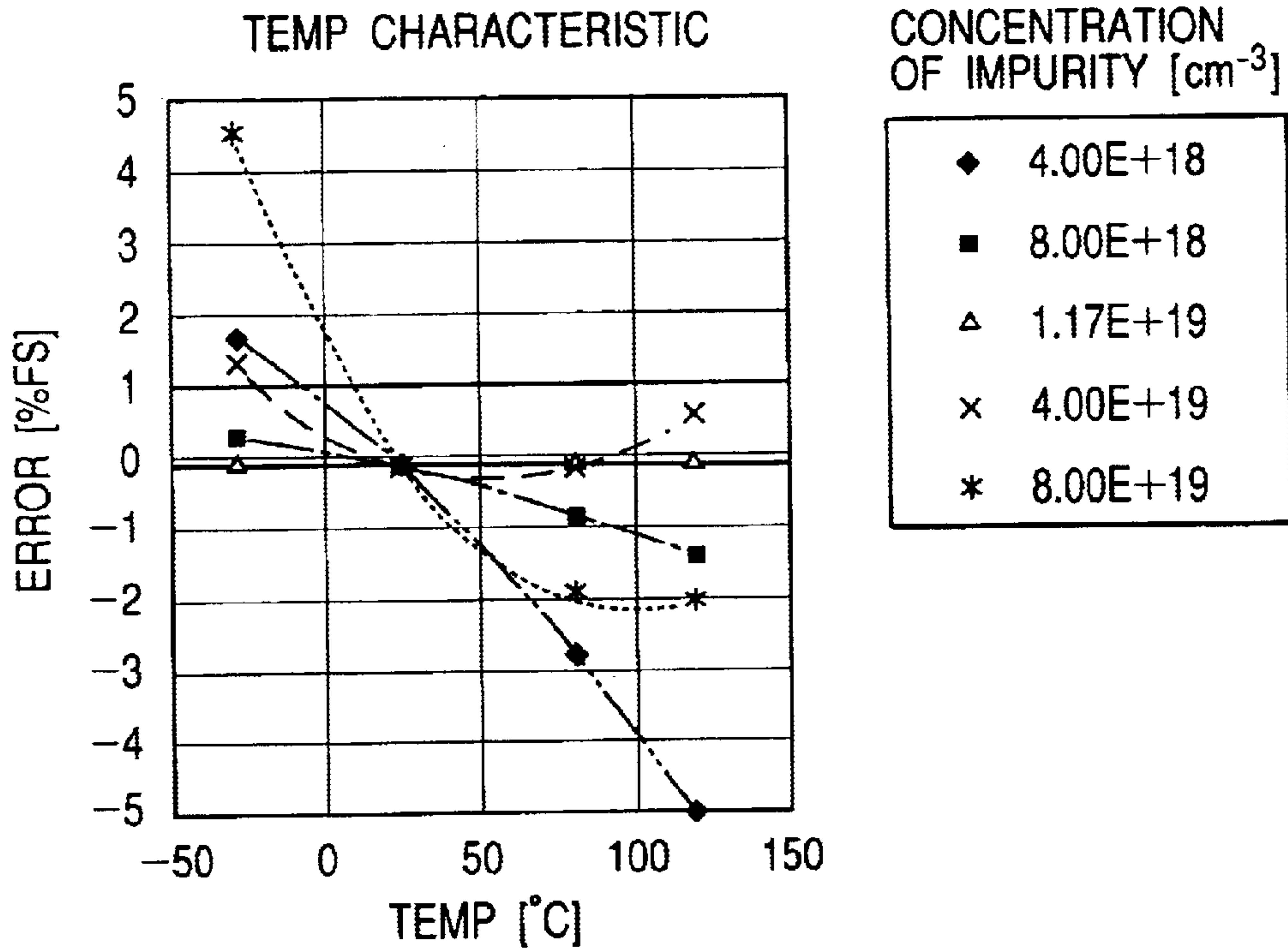
FIG. 4A
