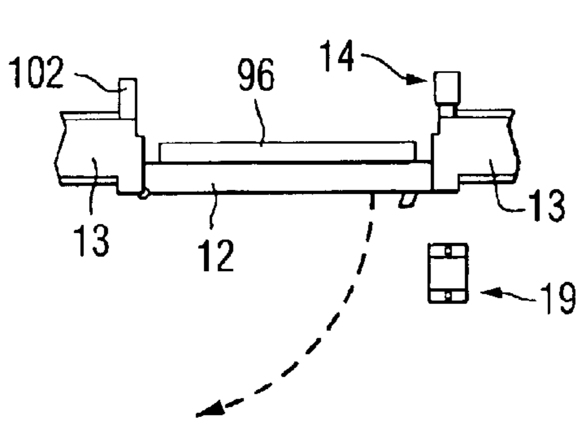
LEFT HAND REAR DOOR FIG. 4C
