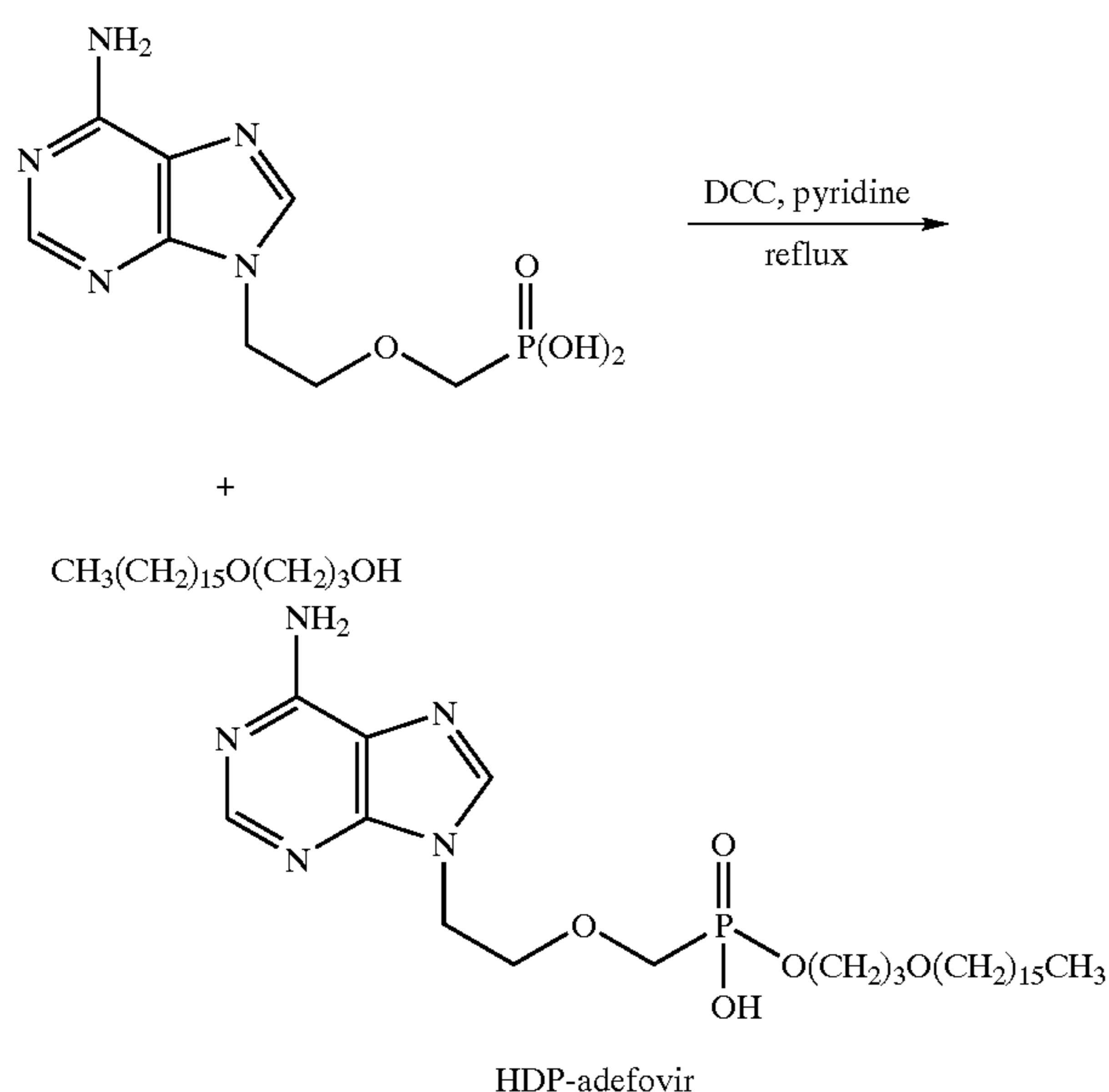
Scheme VI
