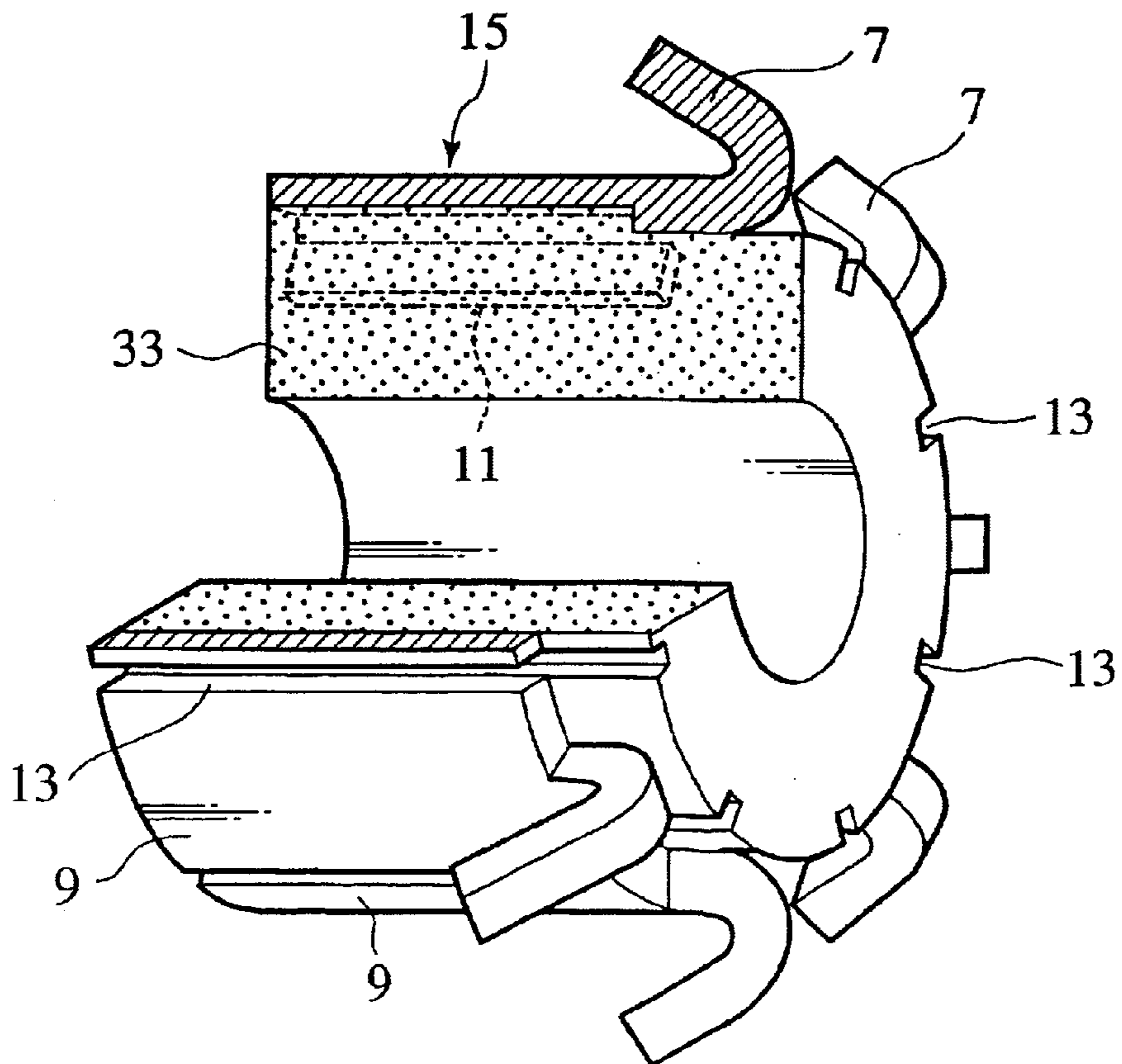
FIG. 8
