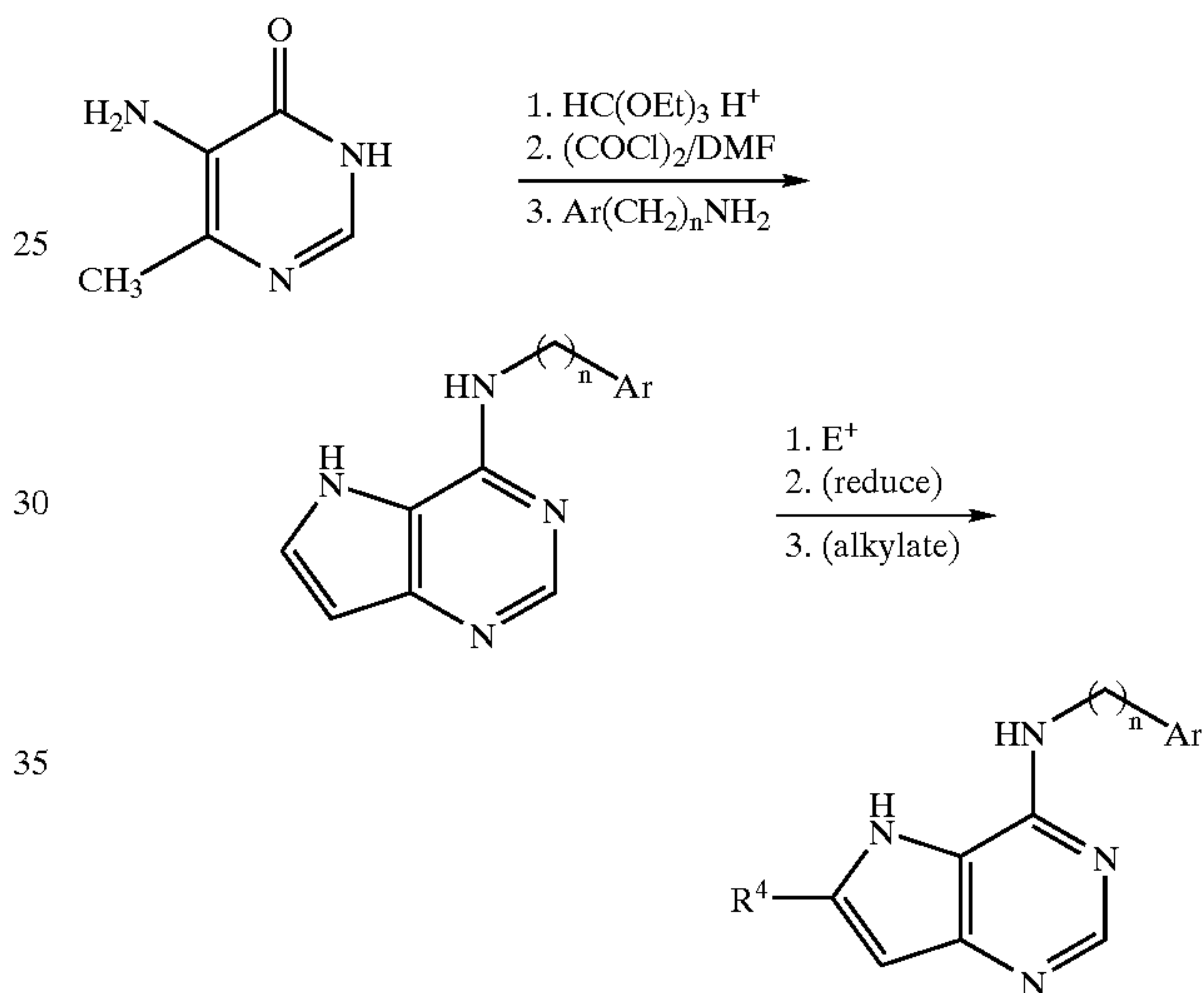
Scheme 23.
