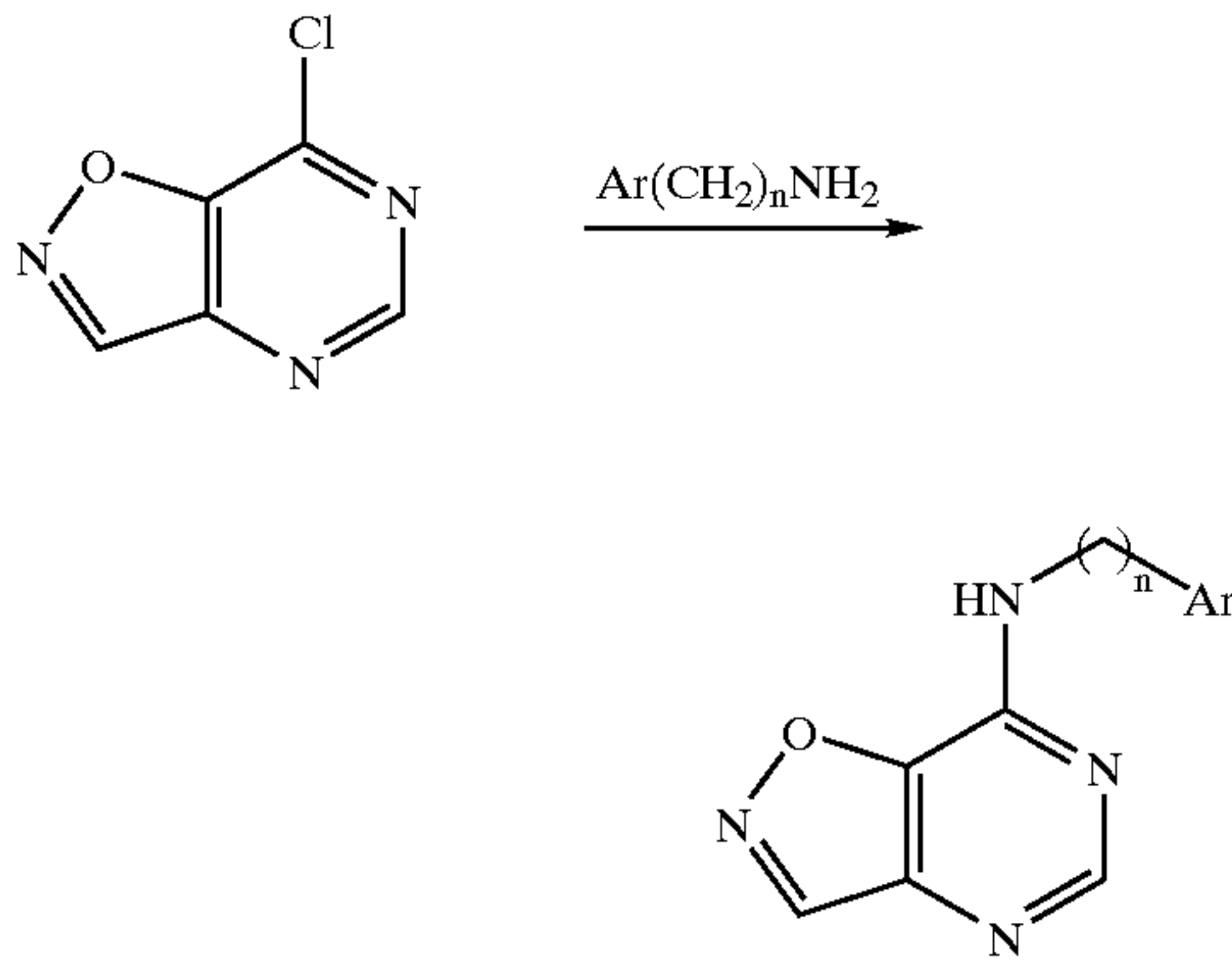
Scheme 30.
