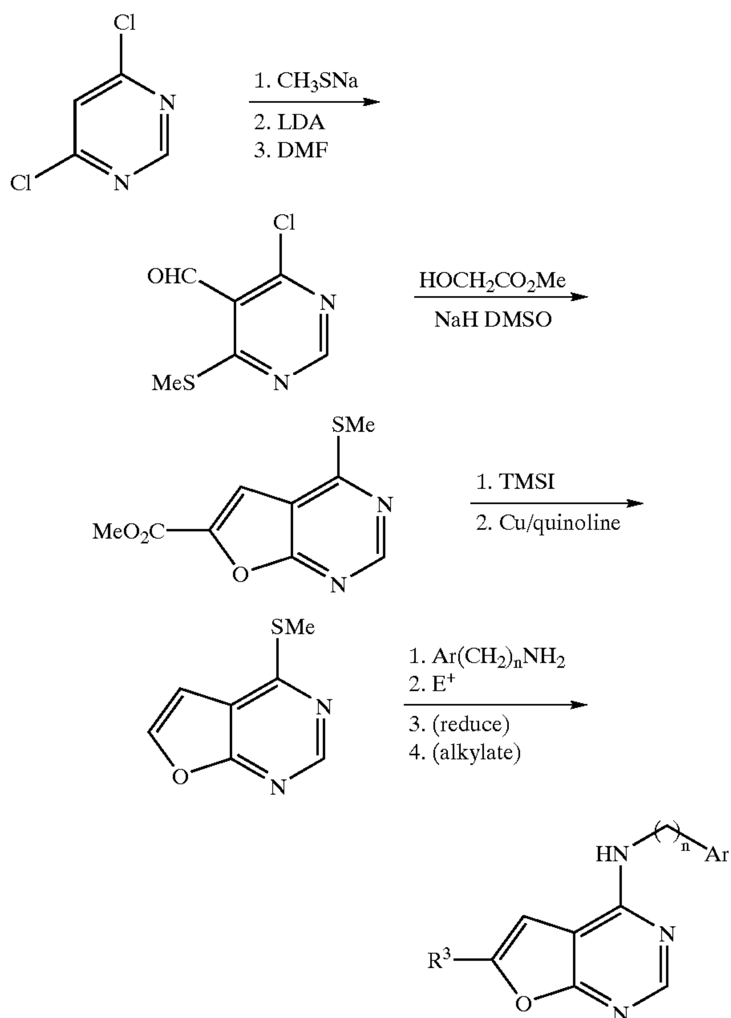
Scheme 21.
