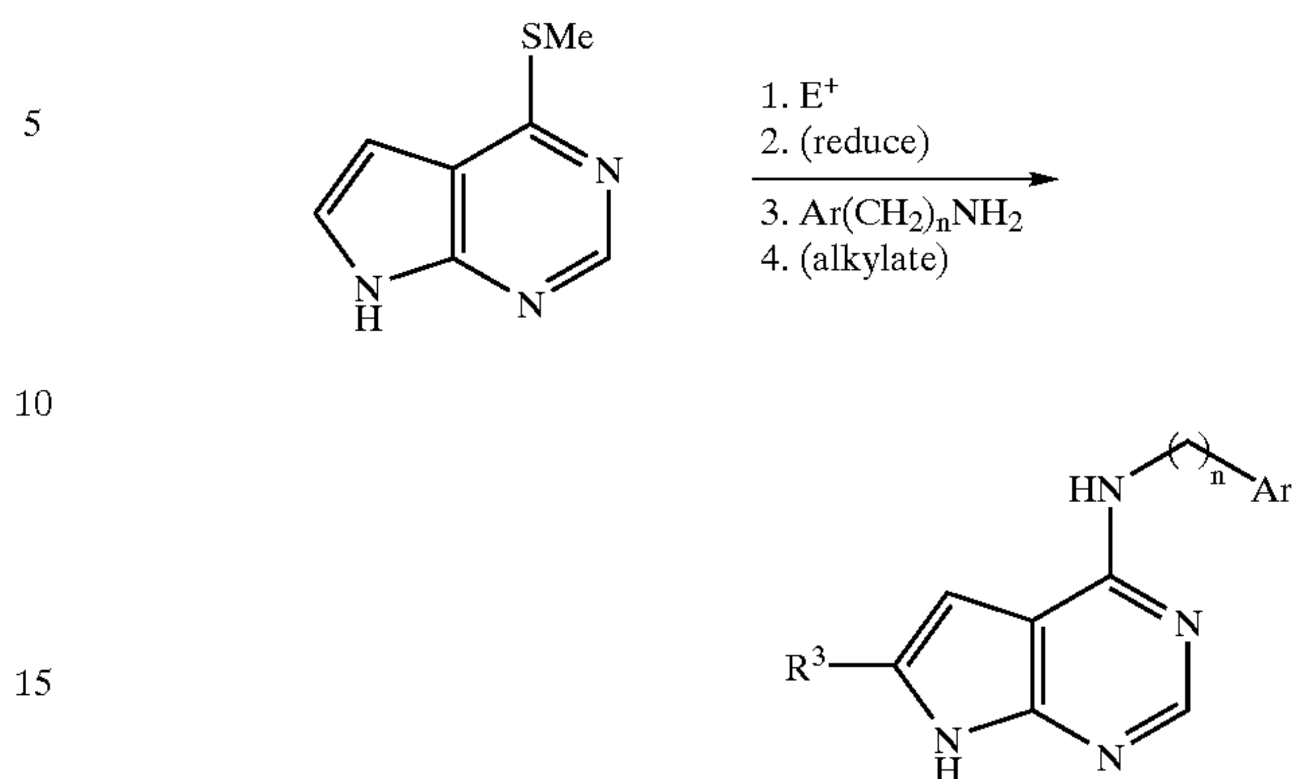
Scheme 22.
