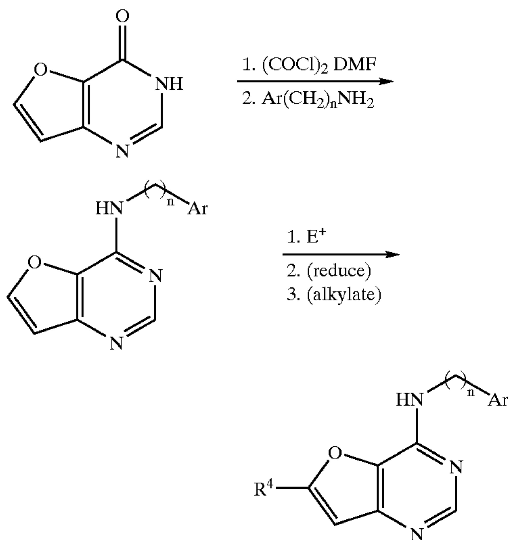
Scheme 20.
