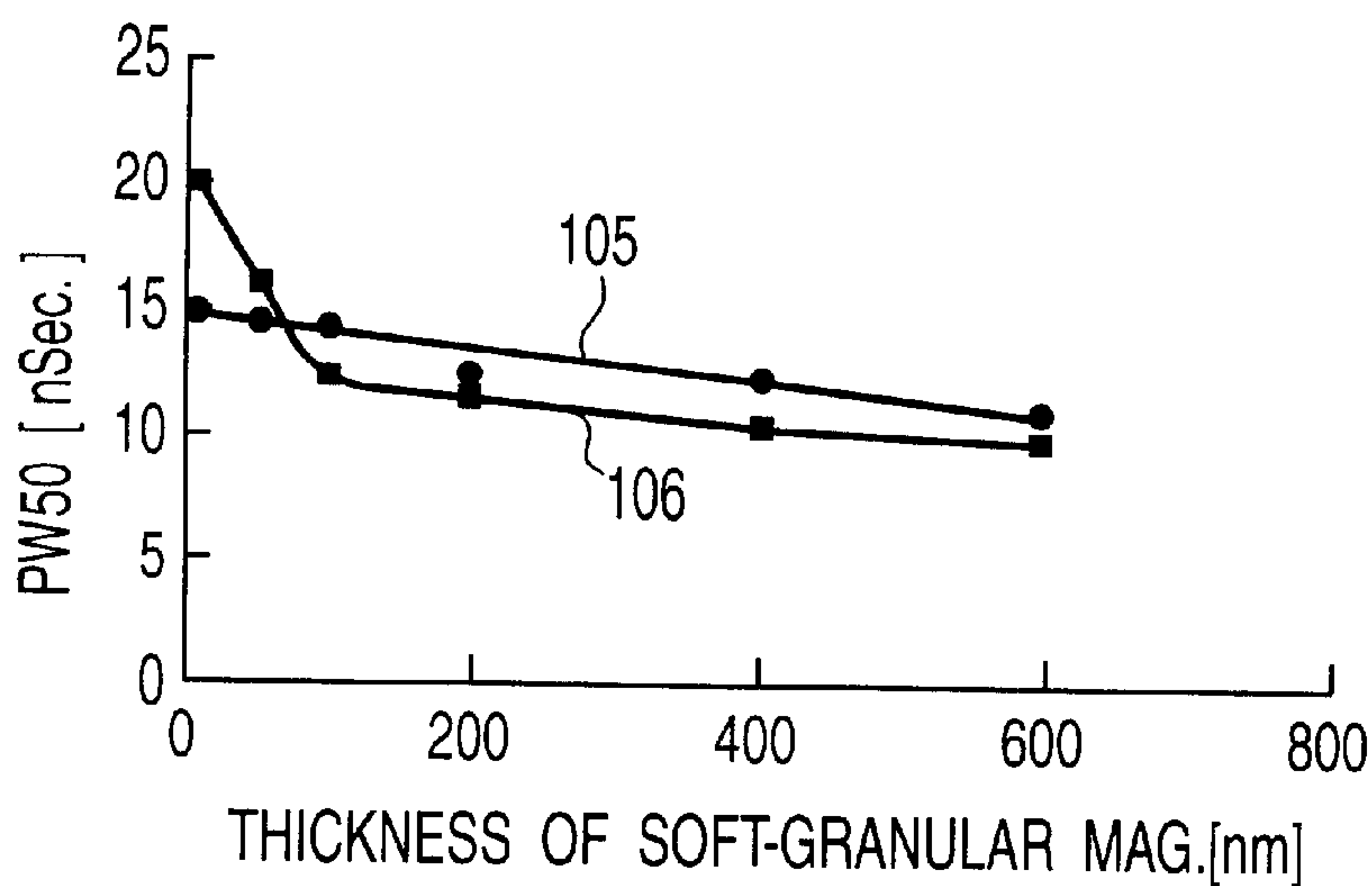
FIG. 16
