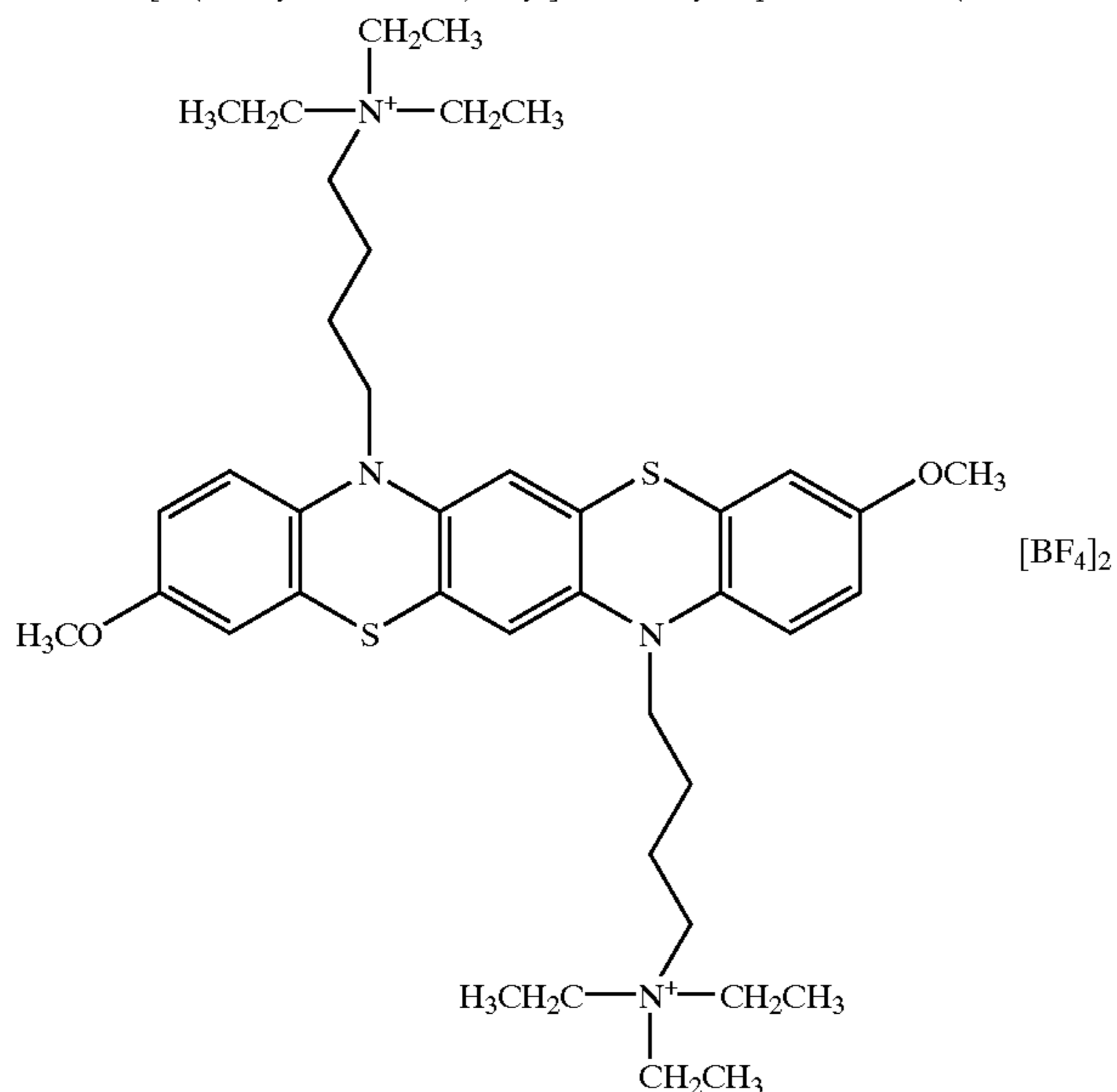
3,10-dimethoxy-7,14-(4-triethylammoniumbutyl)triphenodithiazine bis(tetrafluoroborate)
