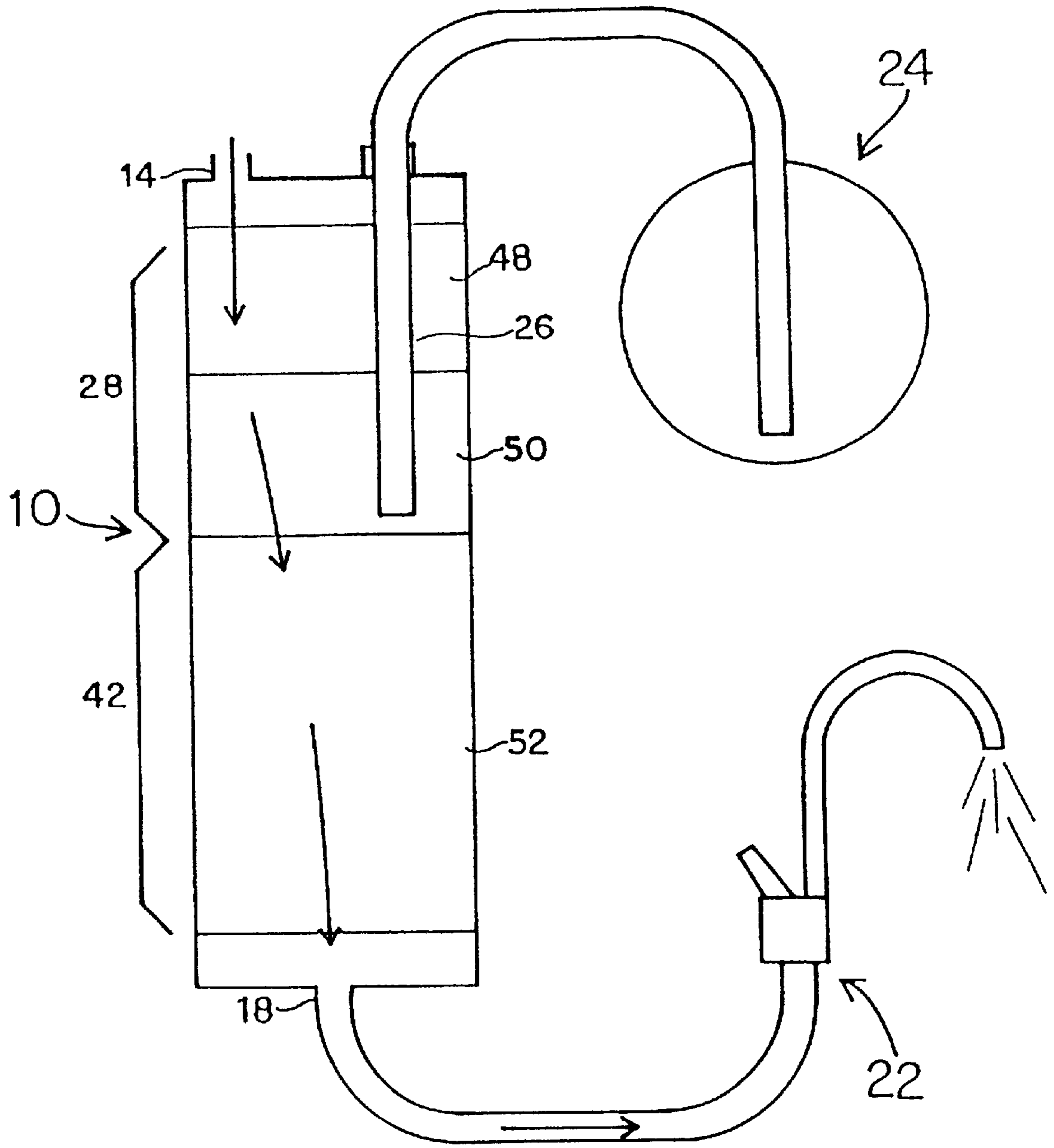
FIG. 2C
