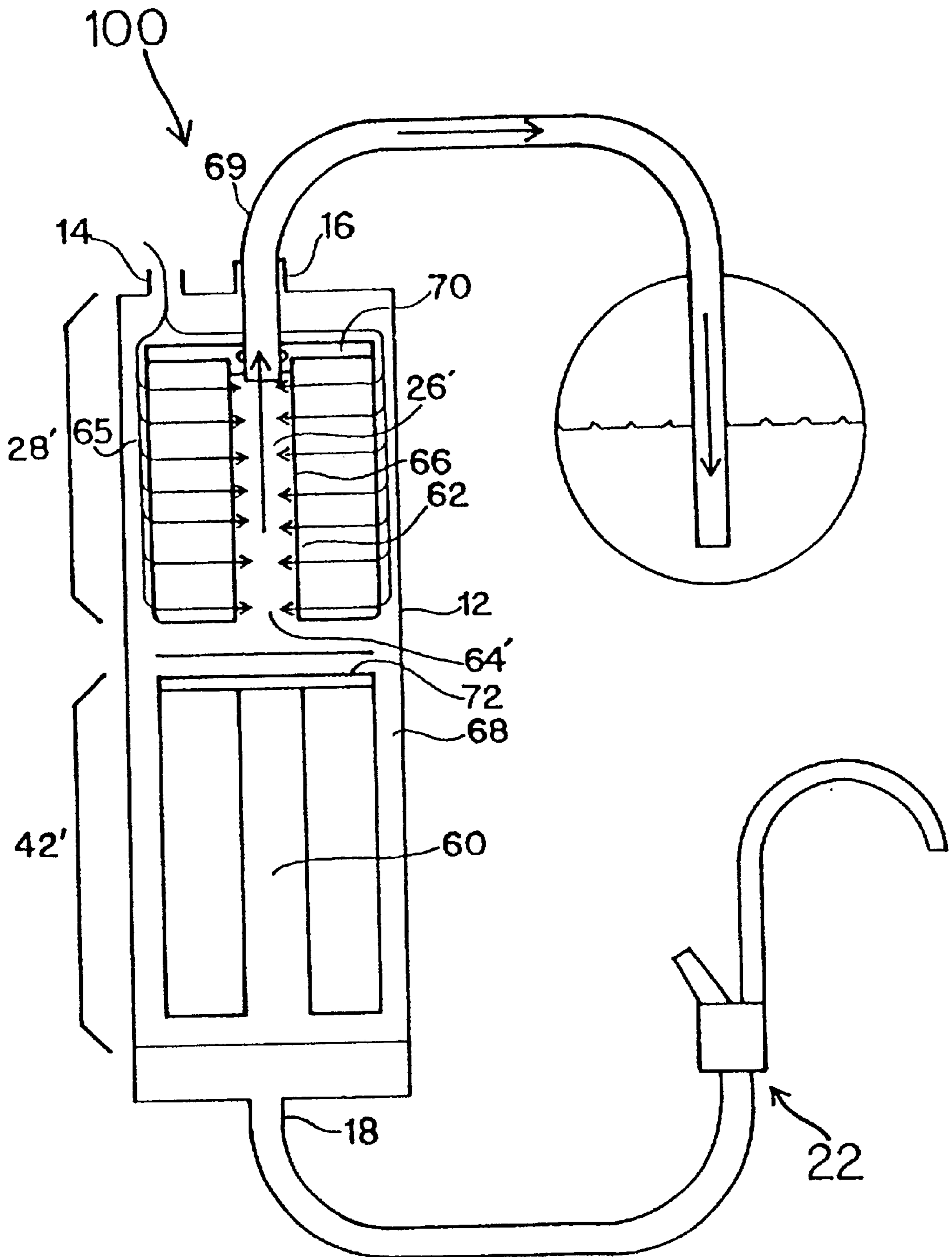
FIG. 3A
