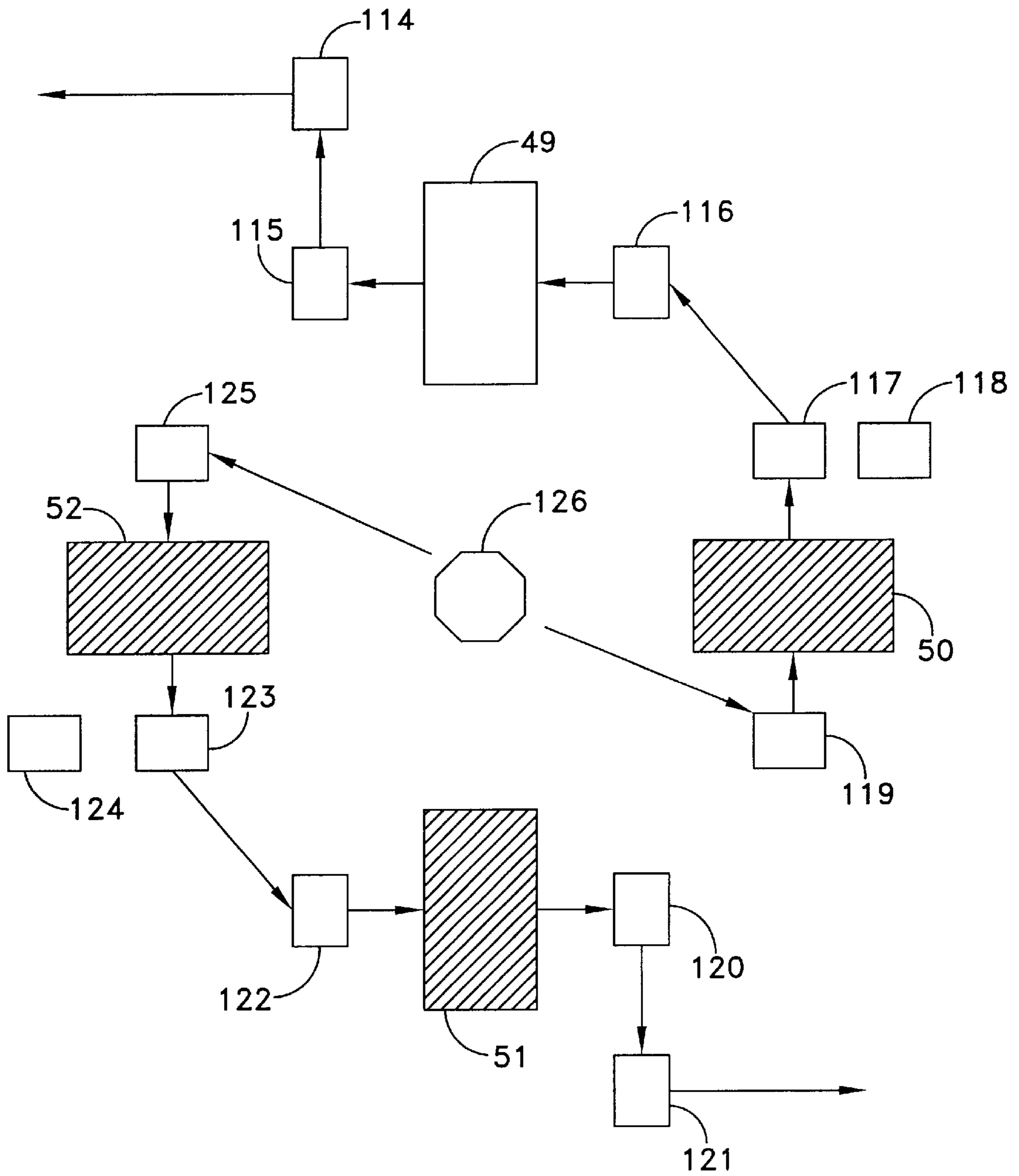
FIG. 13
