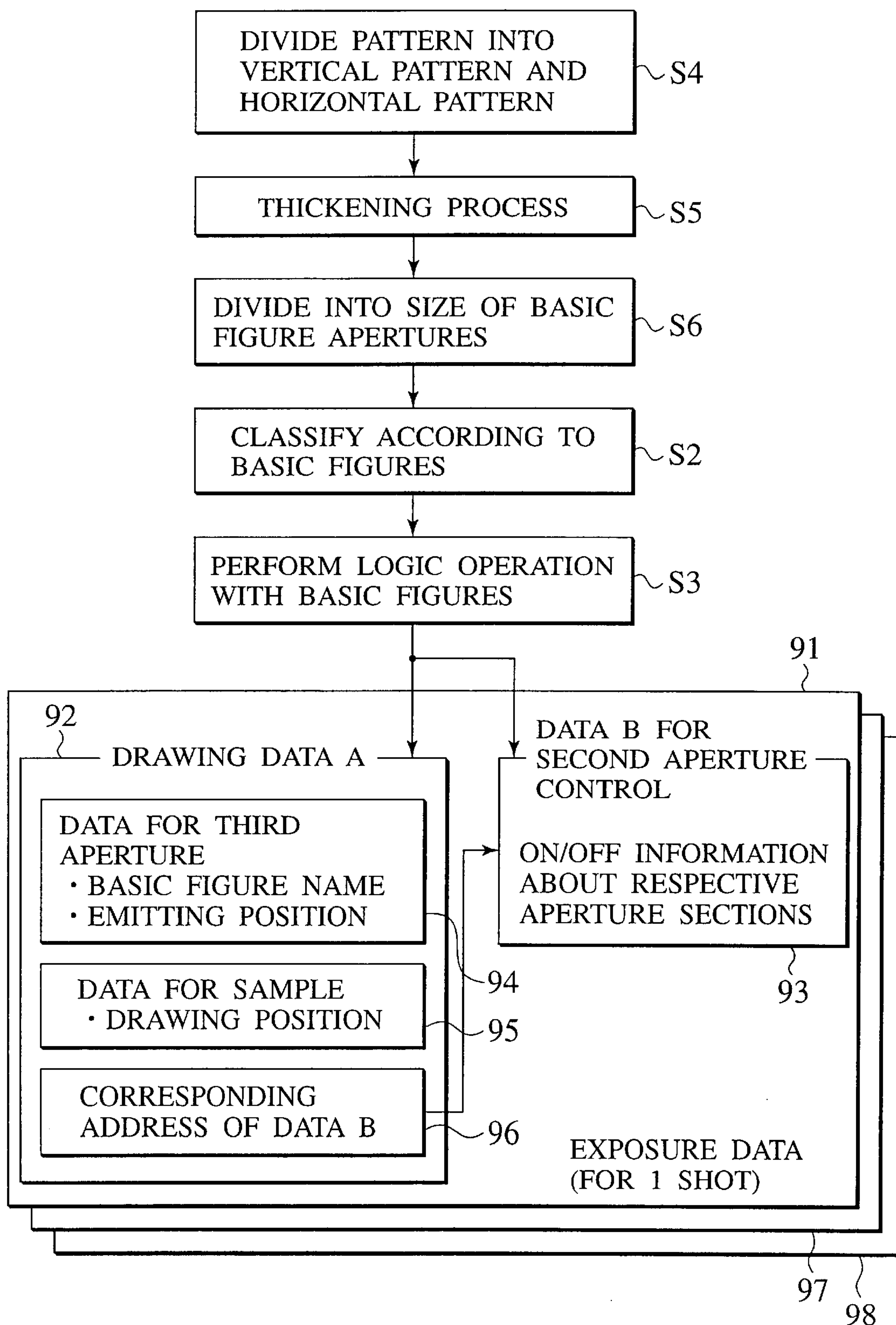
FIG.11
