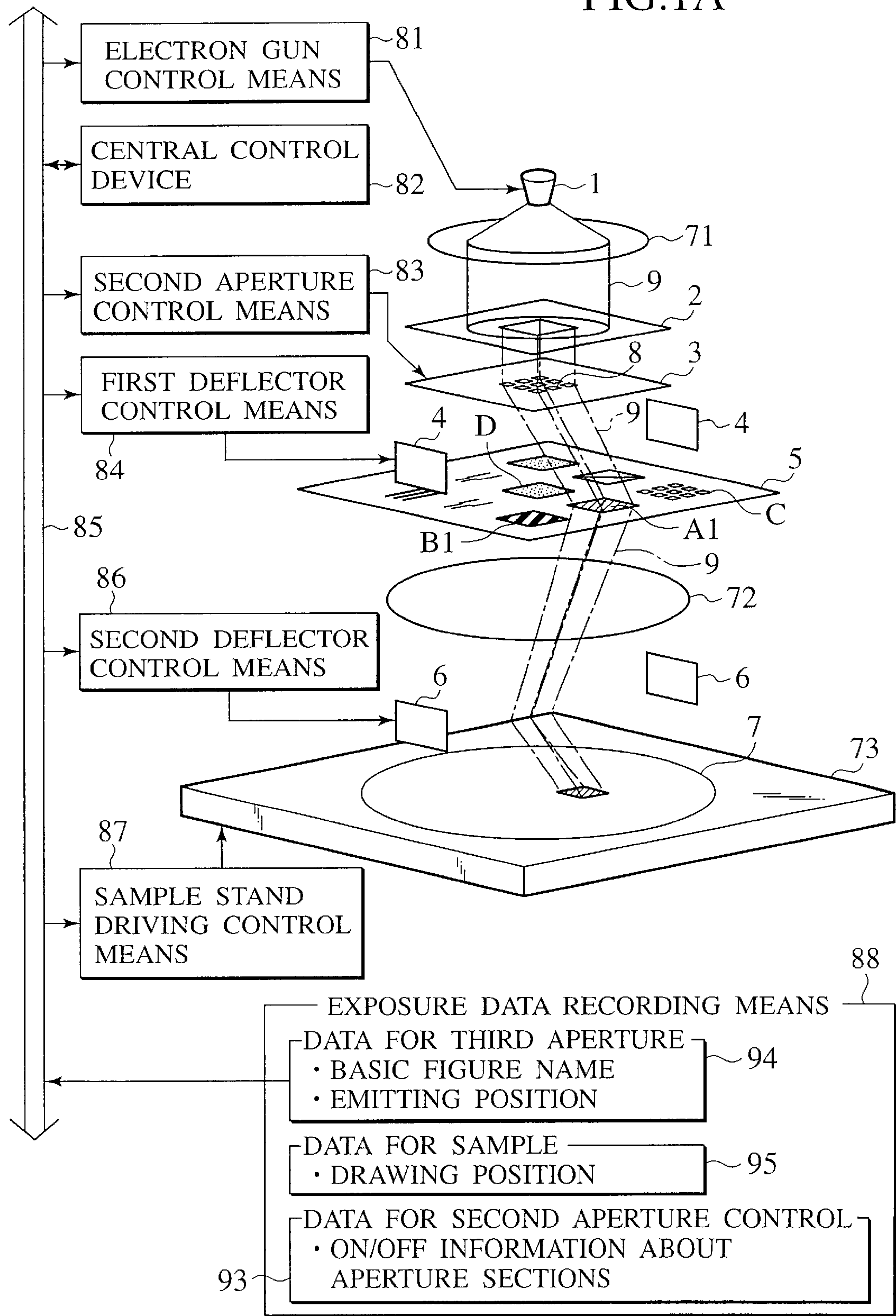
FIG.1A
