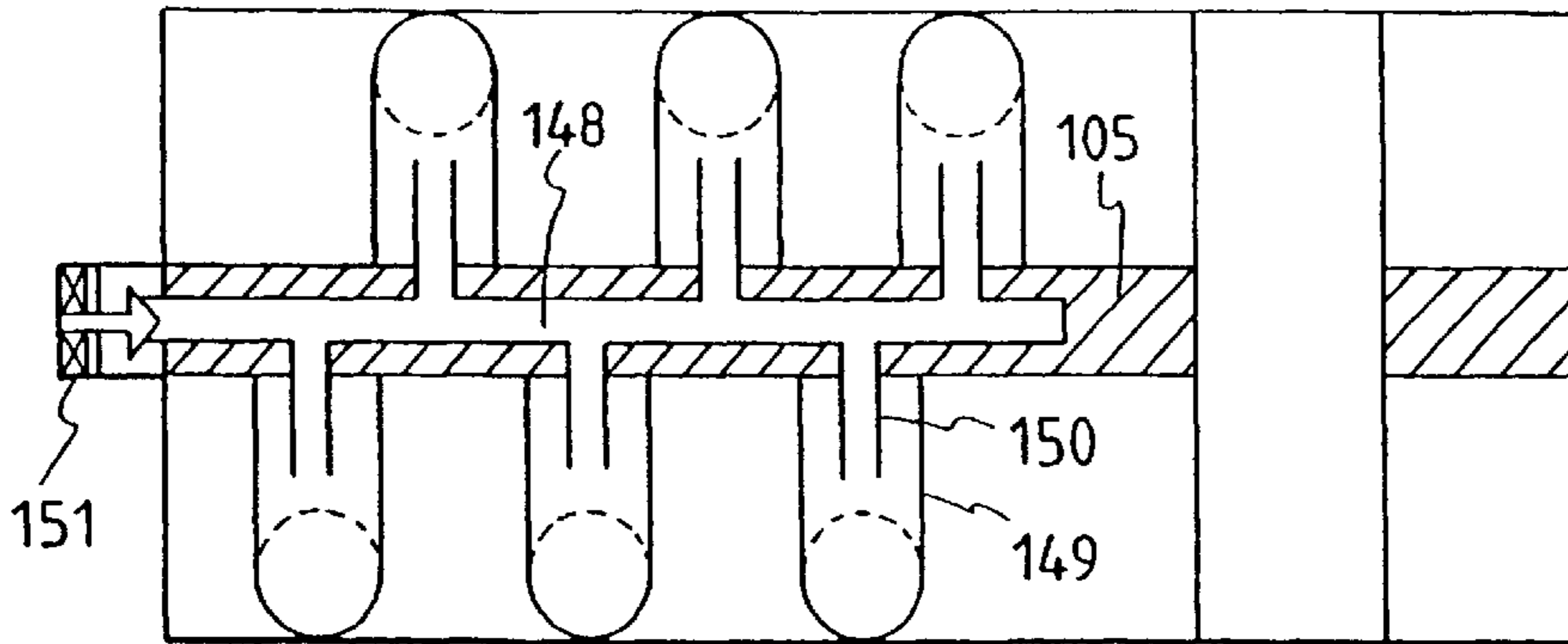
SECTION A-A
