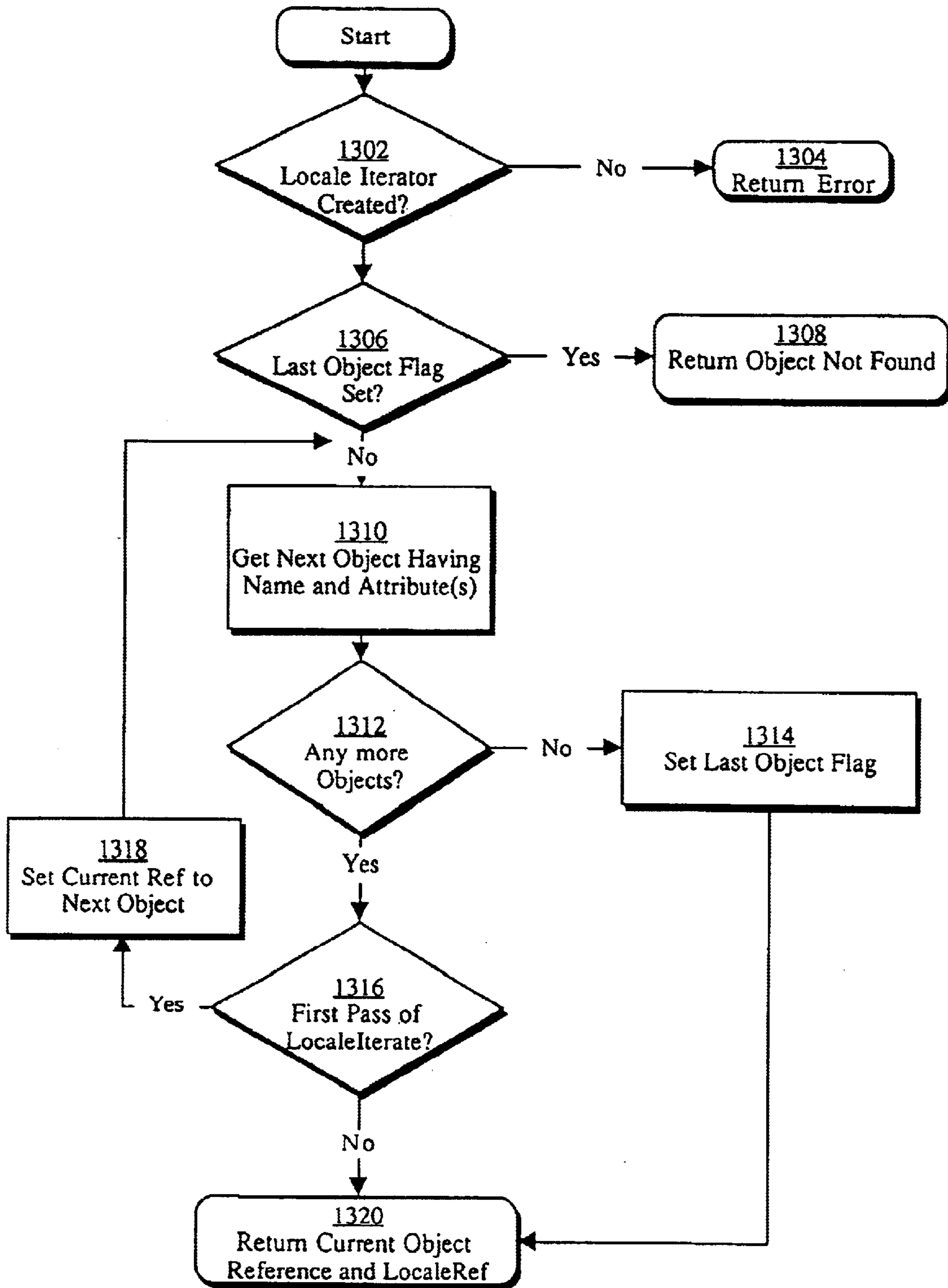
FIG. 13 LocaleIterate 1007
